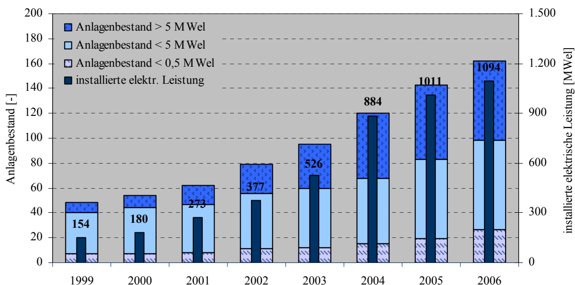
Abbildung 2-1: Anlagenbestand und installierte Leistung der Biomasse(heiz)kraftwerke
