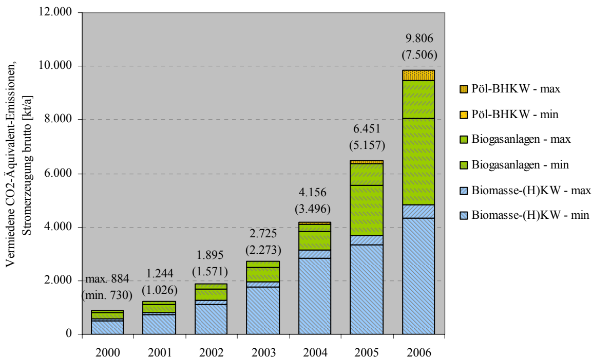
Abbildung 2-4: Entwicklung der vermiedenen CO 2 -Emissionen durch Einsatz von Biomasse zur Stromerzeugung (Bruttobilanz ohne Berücksichtigung von Wärmegutschriften aus KWK)
