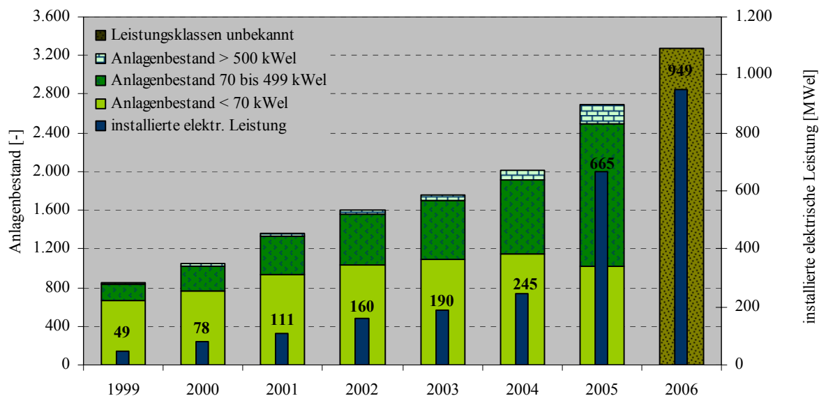
Abbildung 2-3: Anlagenbestand und installierte elektrische Leistung der Biogasanlagen
