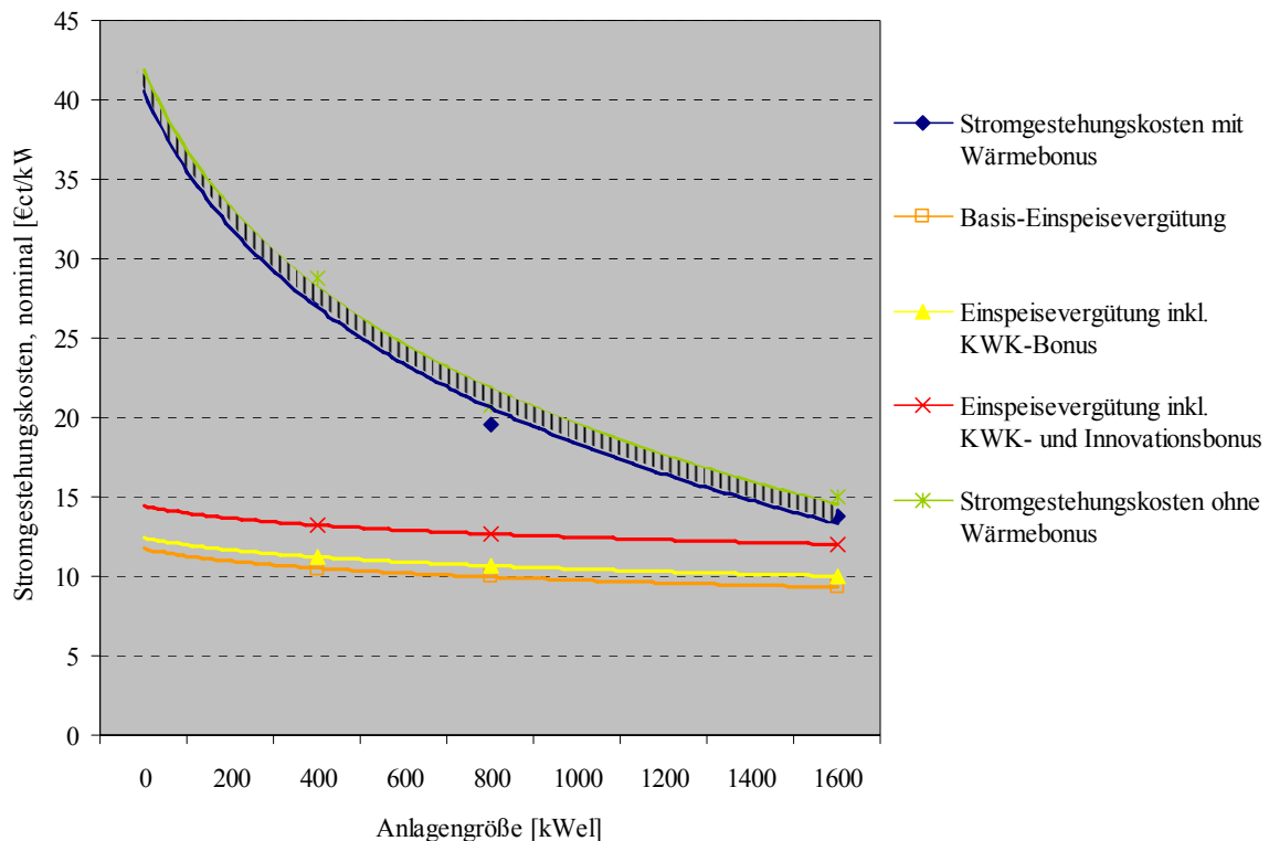
Abbildung 5-2: Stromgestehungskosten und Vergütungen in Abhängigkeit von der Anlagengröße (Vergütungsbasis: 2006, Bioabfallerlös: 60 €/t)
