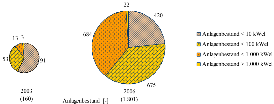
Abbildung 2-2: Anlagenbestand der Pflanzenöl-BHKW für 2003 (inkl. RME-BHKW) und 2006
