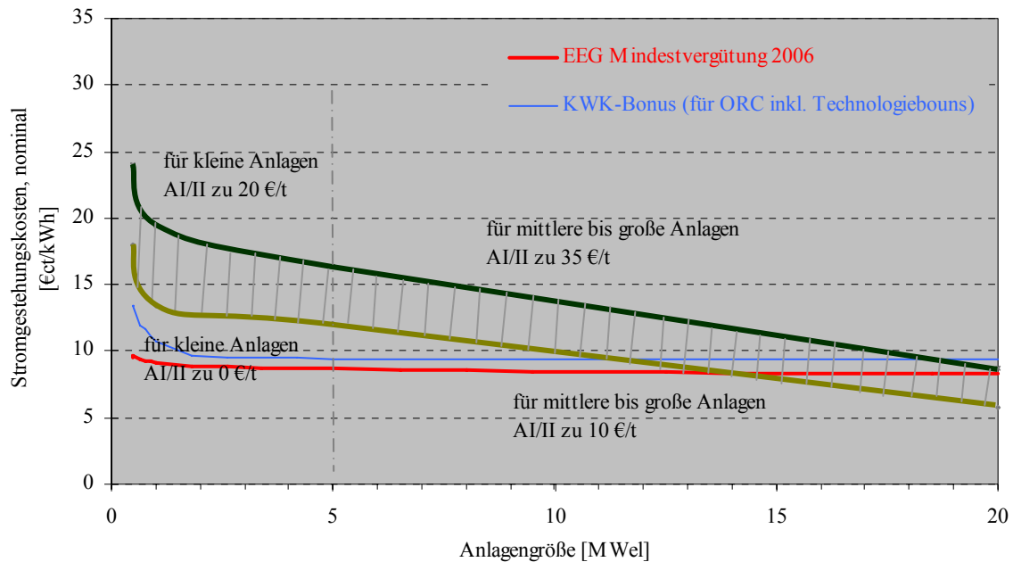
Abbildung 3-3: nominale Stromgestehungskosten für Altholz in Biomasse(heiz)kraftwerken in Abhängigkeit von der Anlagengröße; Annahme Brennstoffpreis: 0 bis 35 €/t für Altholz A I/II
