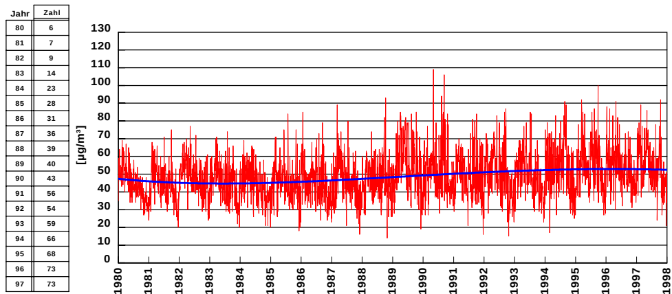
Abb. 3d: Validierte, wetterbereinigte und renormierte 6° GMT Ozonwerte als Mittel über alle "la" Stationen, Sommerhalbjahre 1980 bis 1997
