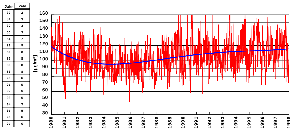
Abb. 2e: Validierte, wetterbereinigte und renormierte Tagesmaxima der Ozonkonzentration als Mittel über alle 'bg' Stationen, Sommerhalbjahre 1980 bis 1997
