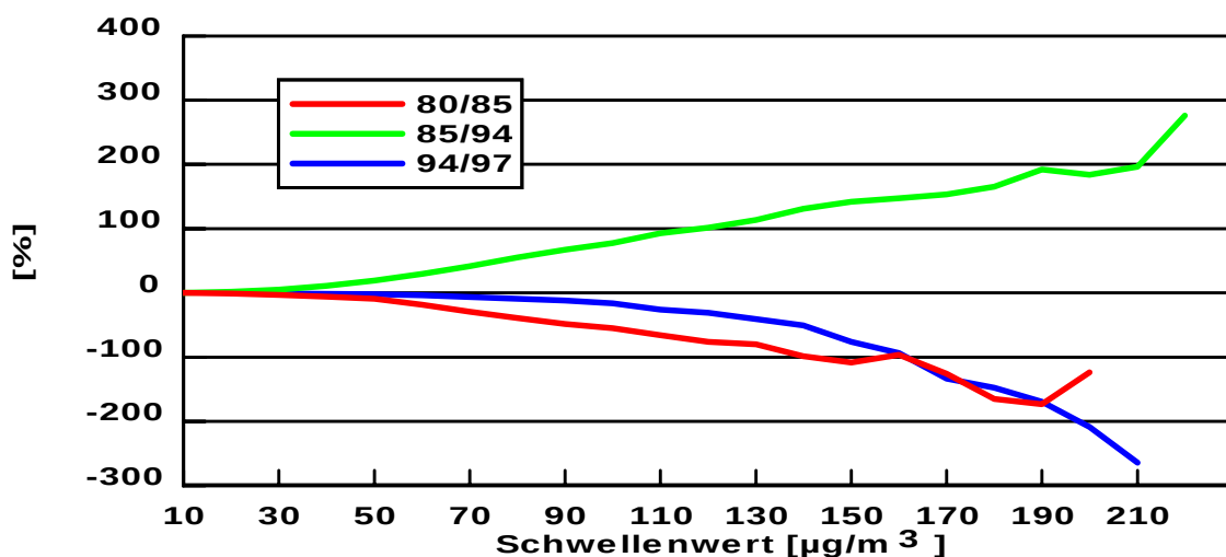
Abb.4: Prozentuale Änderung der Überschreitungshäufigkeiten vorgegebener Schwellenwerte der Tagesmaxima der Ozonkonzentration zwischen Beginn und Ende der untersuchten drei Zeiträume, im Vergleich zur mittleren Überschreitungshäufigkeit im entsprechenden Zeitraum. Validierte, wetterbereinigte und renormierte tägliche Ozonmaxima, alle Stationen, Sommerhalbjahre 1980 bis 1997
