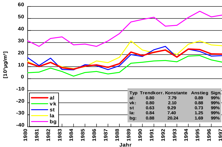
Abb.5: AOT40 Werte als Mittel über alle im entsprechenden Jahr zur Verfügung stehenden Stationen, getrennt nach Stationstypen und über alle Stationen
