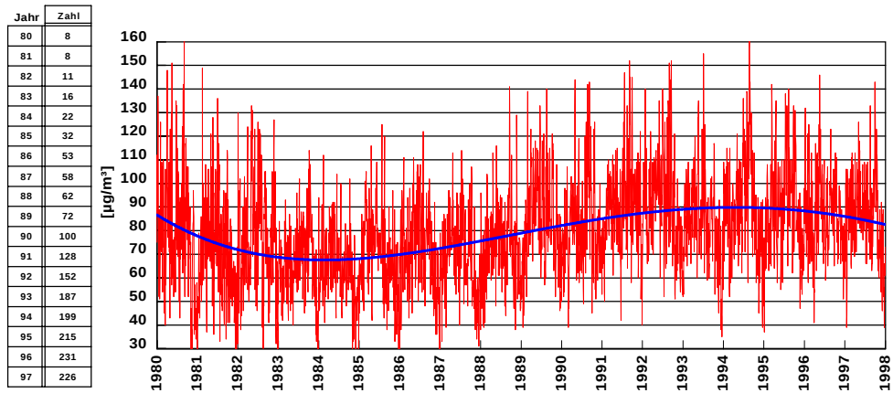
Abb. 2c: Validierte, wetterbereinigte und renormierte Tagesmaxima der Ozonkonzentration als Mittel über alle 'st' Stationen, Sommerhalbjahre 1980 bis 1997
