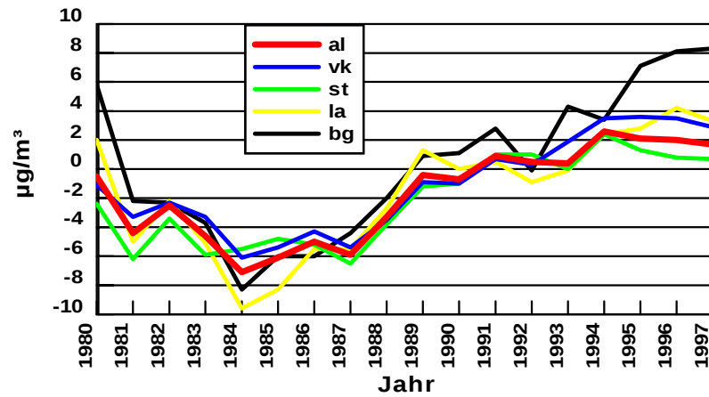
Abb.6: Jahresmittelwerte der Bodenozonekonzentration als Abweichung vom stationsspezifischen Stichprobenklima und als Mittel über alle im betreffenden Jahr vorhandenen Stationen
