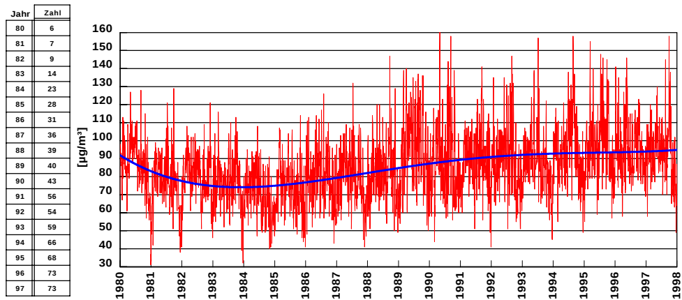
Abb. 2d: Validierte, wetterbereinigte und renormierte Tagesmaxima der Ozonkonzentration als Mittel über alle 'la' Stationen, Sommerhalbjahre 1980 bis 1997
