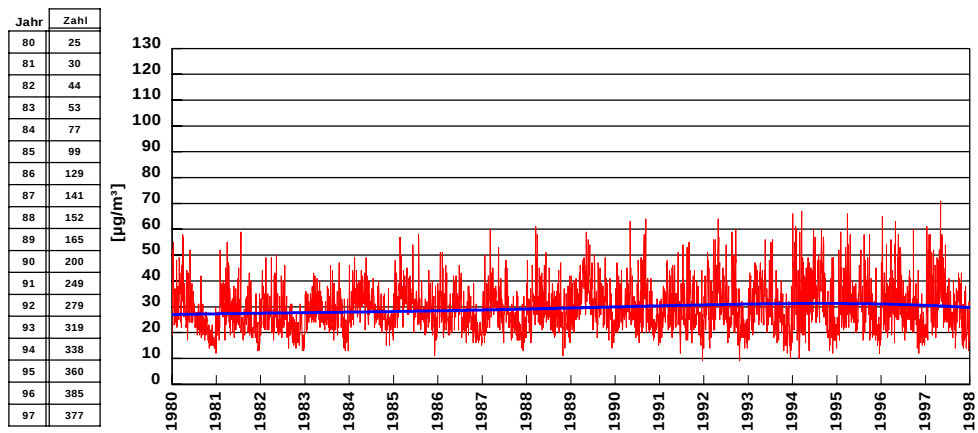
Abb. 3a: Validierte, wetterbereinigte und renormierte 6° GMT Ozonwerte als Mittel über alle Stationen, Sommerhalbjahre 1980 bis 1997
