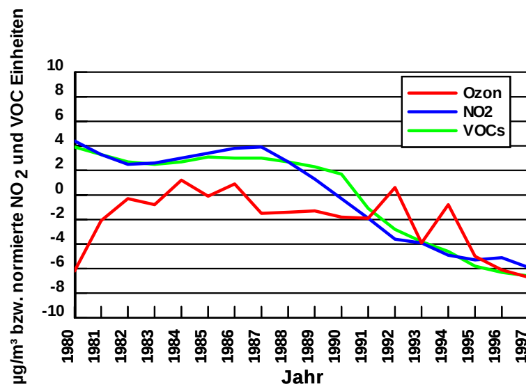
Abb. 11: Abweichungen der Jahresmittelwerte der Bodenozonekonzentration von den Jahresmittelwerten der Bergstationen (mittlere regionale Komponente der Ozonkonzentration) im Vergleich zum normierten jährlichen NO 2 und VOC Ausstoß
