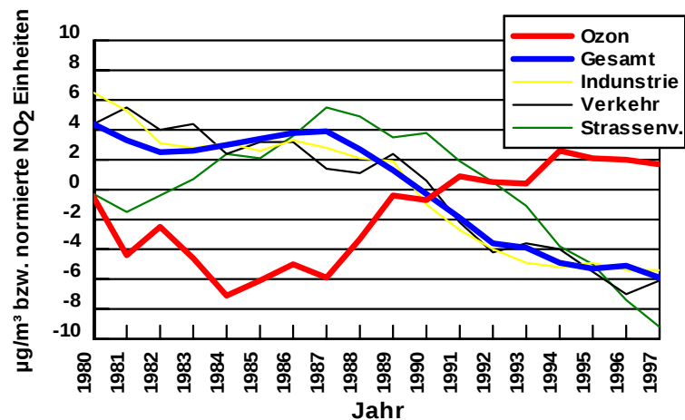
Abb. 10a: Jahresmittelwerte der Bodenozonekonzentration im Vergleich zum normierten jährlichen \text{NO}_2 Ausstoß
