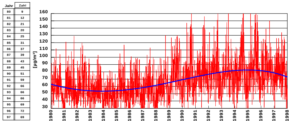
Abb. 2b: Validierte, wetterbereinigte und renormierte Tagesmaxima der Ozonkonzentration als Mittel über alle 'vk' Stationen, Sommerhalbjahre 1980 bis 1997
