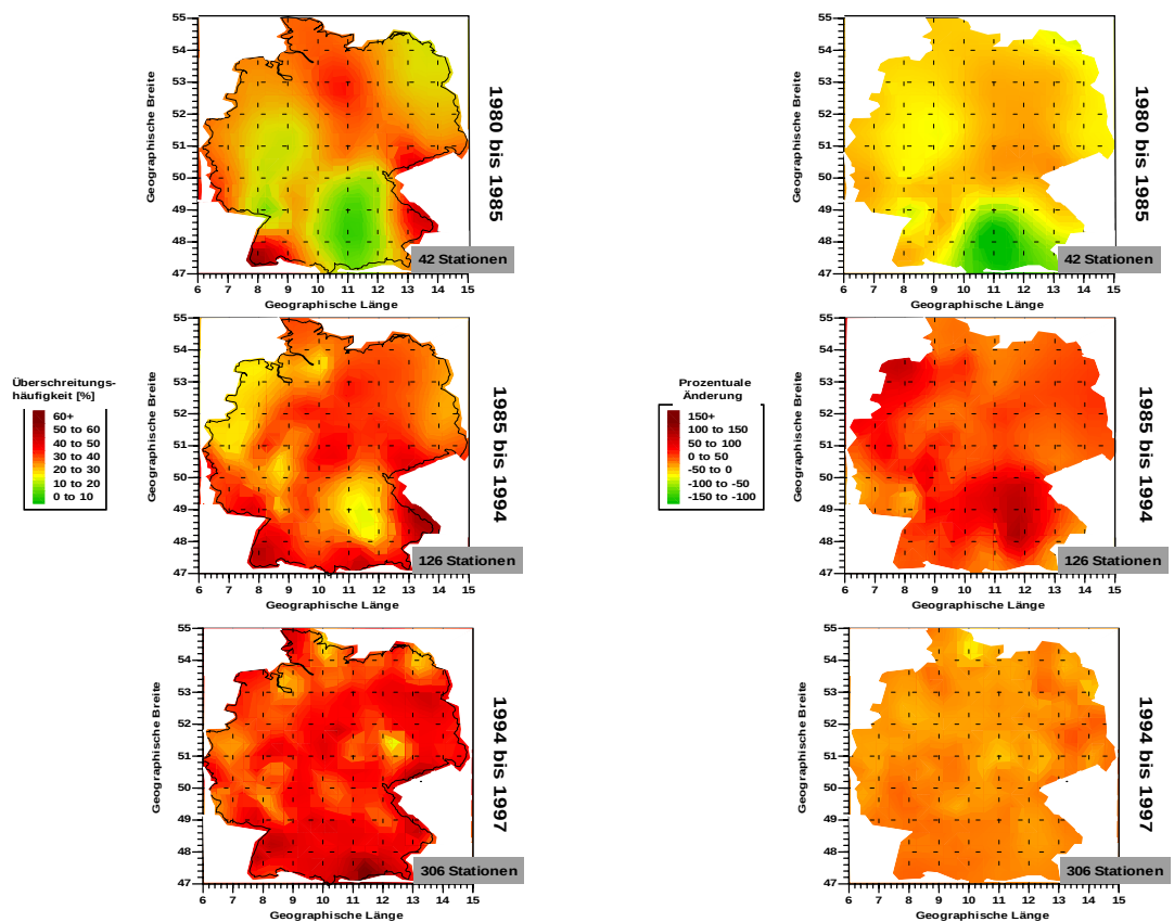
Abb. 7a: Mittlere Überschreitungshäufigkeit der Ozontagesmaxima > 80 \mu\text{g}/\text{m}^3
