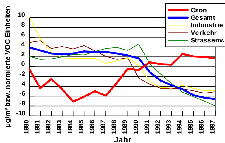
Abb. 10b: Jahresmittelwerte der Bodenozonekonzentration im Vergleich zum normierten jährlichen VOC Ausstoß
