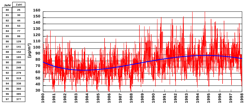
Abb. 2a: Validierte, wetterbereinigte und renormierte Tagesmaxima der Ozonkonzentration als Mittel über alle Stationen, Sommerhalbjahre 1980 bis 1997
