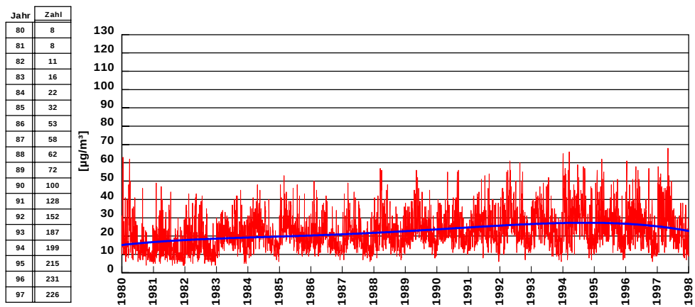
Abb. 3c: Validierte, wetterbereinigte und renormierte 6° GMT Ozonwerte als Mittel über alle "st" Stationen, Sommerhalbjahre 1980 bis 1997
