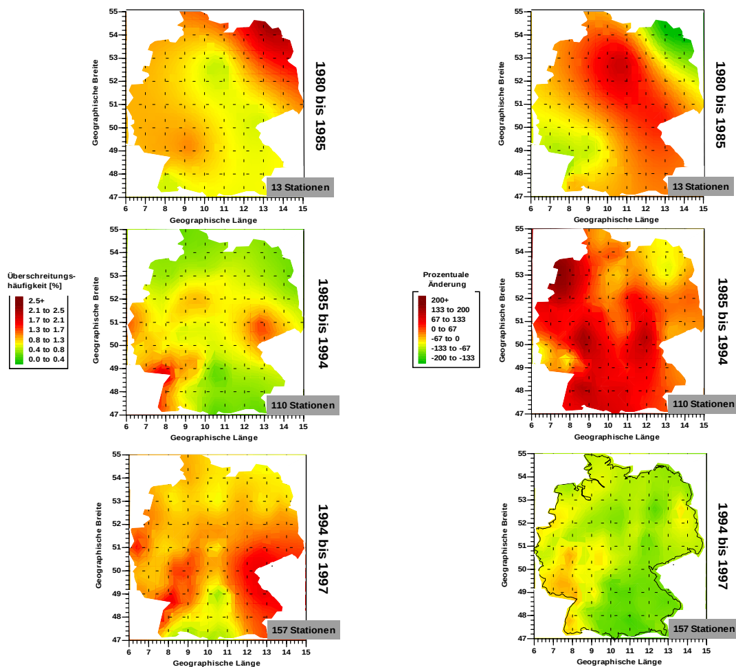
Abb. 8b: Prozentuale Änderung der Überschreitungshäufigkeit der mittleren Überschreitungshäufigkeit des entspr. Zeitintervalls - Ozontagesmaxima > 180 \mu\text{g}/\text{m}^3
