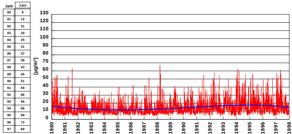
Abb. 3b: Validierte, wetterbereinigte und renormierte 6° GMT Ozonwerte als Mittel über alle "vk" Stationen, Sommerhalbjahre 1980 bis 1997
