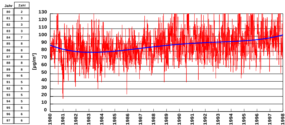
Abb. 3e: Validierte, wette bereinigte und renormierte 6° GMT Ozonwerte als Mittel über alle "bg" Stationen, Sommerhalbjahre 1980 bis 1997
