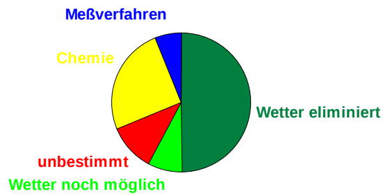
Abb. 1: Relativer Beitrag zur Variabilität der täglichen Ozonmaxima
