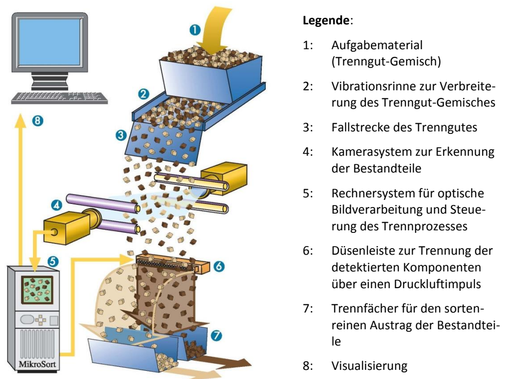
Bild 2.7c: Funktionsprinzip MikroSorter (Quelle: Fa. Mogensen)
