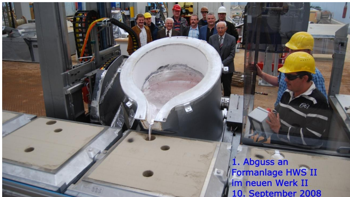
Bild 4.1: Erster Abguss im neuen Werk, deutlich ist die zunächst helle Färbung des Formstoffs zu erkennen.
