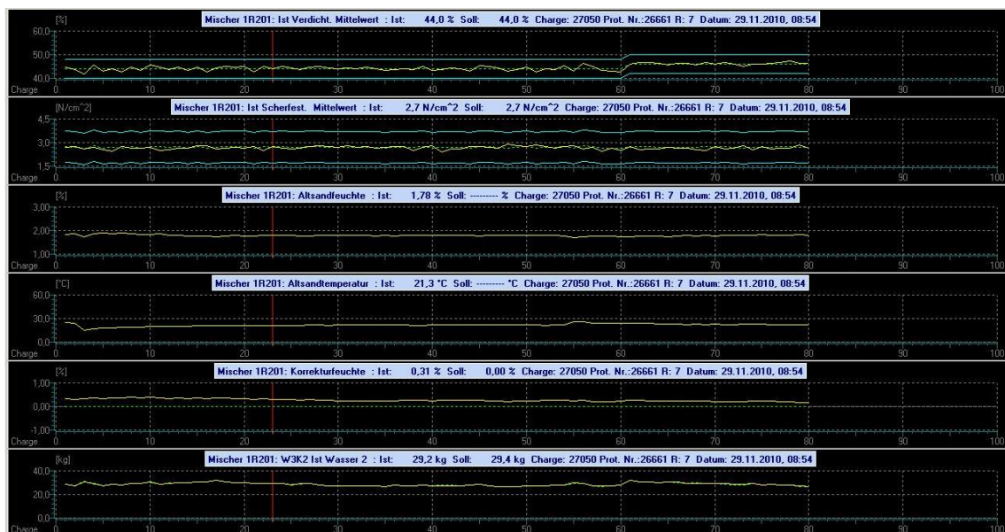
Bild 2.14: Online-Messauswertung der technologischen Eigenschaften der Sandmischungen mit dem Eirich-SandExpert
