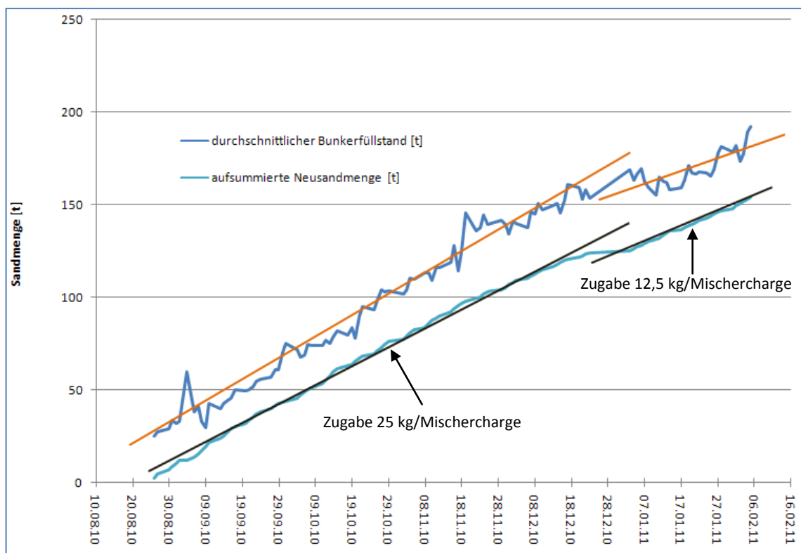
Bild 3.8: Auswirkung der Neusandzugabe auf die Bunkerfüllstände
