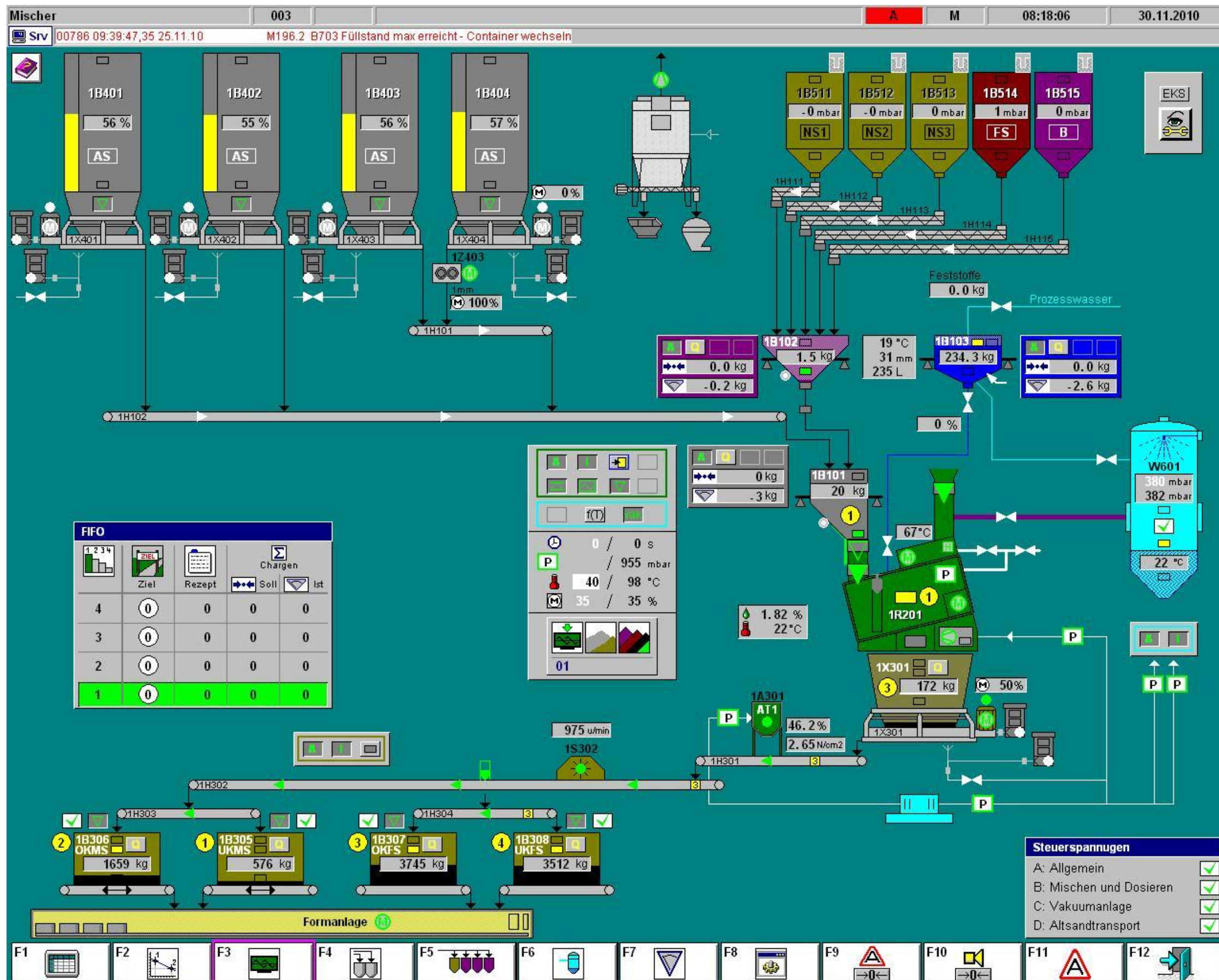
Bild 2.3: Leitstandsgraphik der Frischsandstrecke der EIRICH-Sandaufbereitung: Jedes Aggregat ist mit einer entsprechenden Kennzeichnung versehen.
