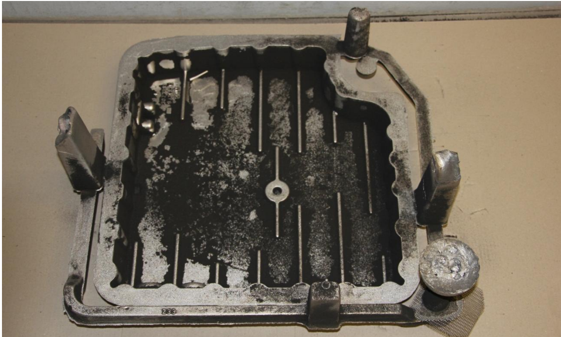
Bild 3.6: Gusstraube mit anhaftendem Restformstoff
