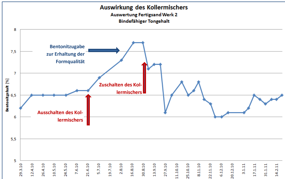
Bild 3.4: Erprobung der Auswirkung des Kollermischers
