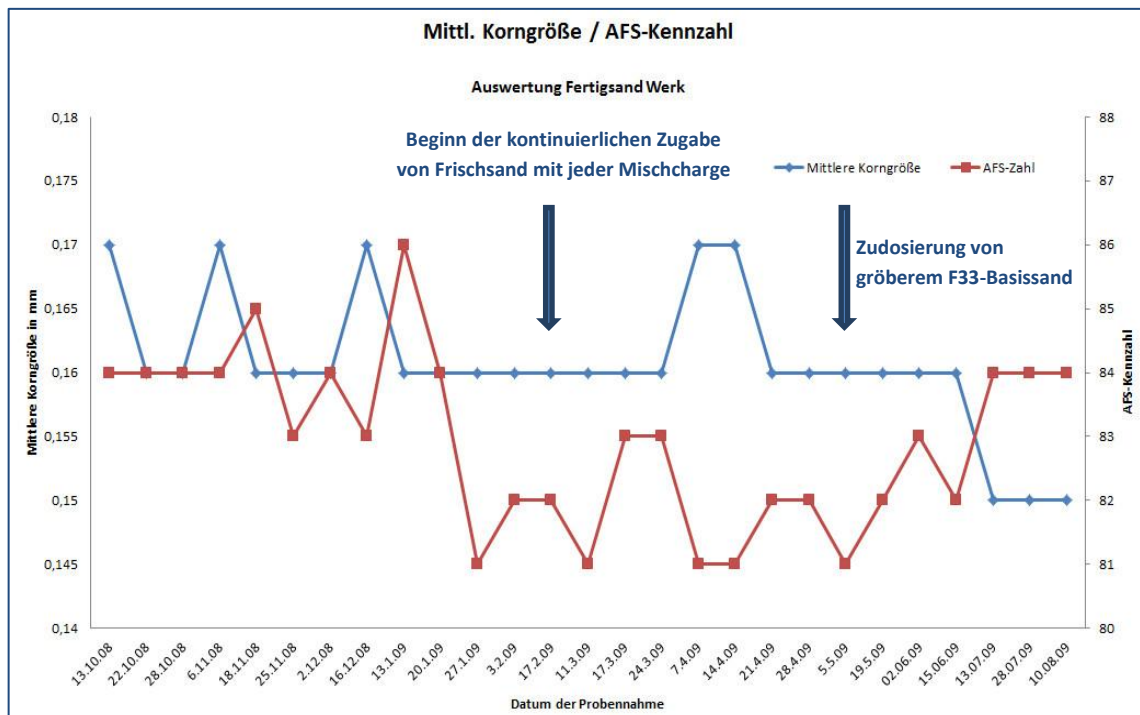
Bild 3.2: Korngröße und AFS-Kennzahl
