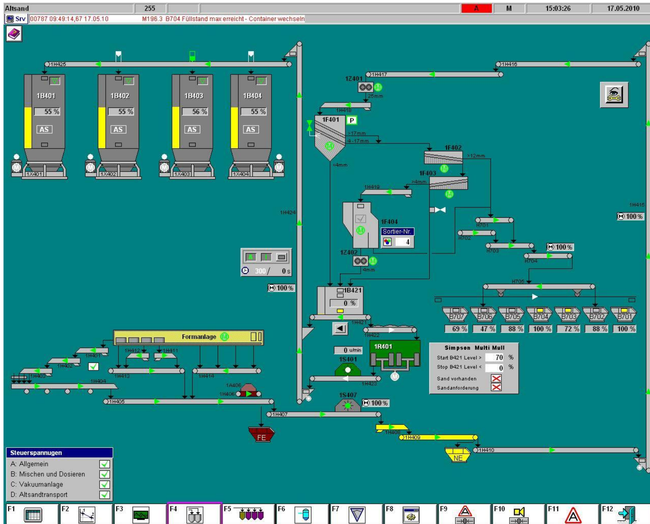
Bild 2.2: Leitstandsgraphik der Altsandstrecke der EIRICH-Sandaufbereitung: Jedes Aggregat ist mit einer entsprechenden Kennzeichnung versehen.
