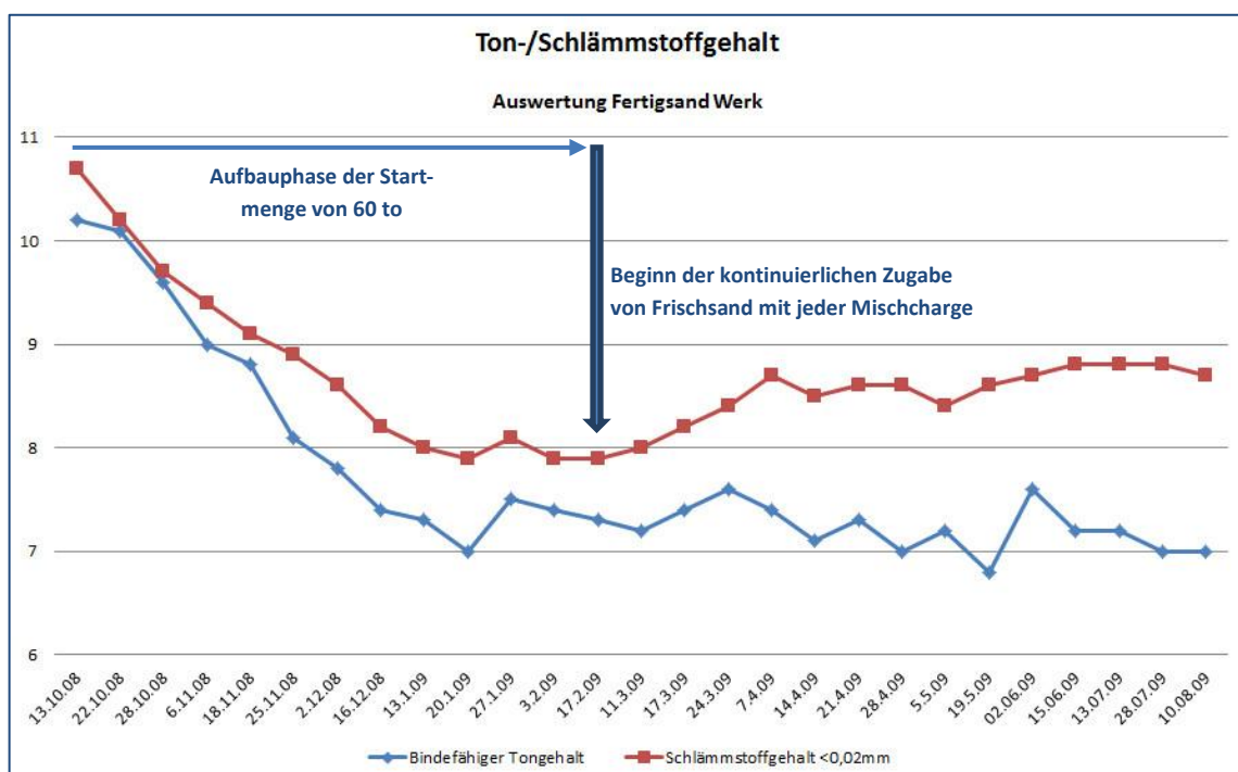
Bild 3.1: Verlauf des Bentonit und Schlammstoffgehaltes in der Aufbauphase des Sandsystems
