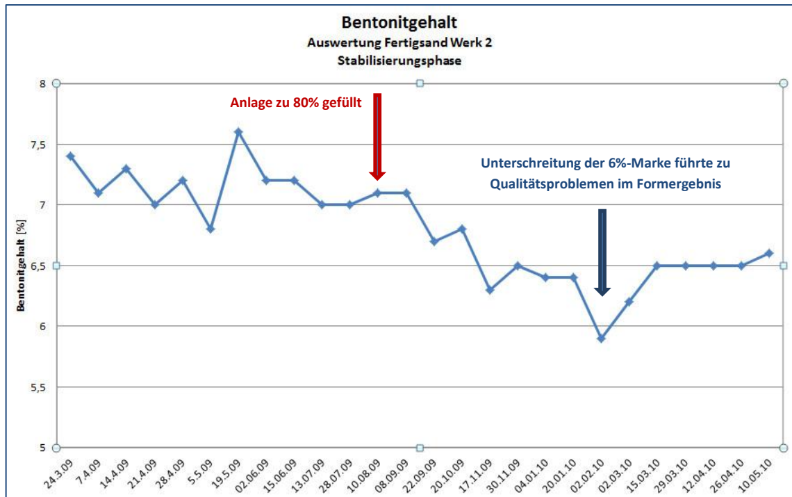
Bild 3.3: Bindefähiger Tongehalt (Bentonitgehalt) in der Stabilisierungsphase
