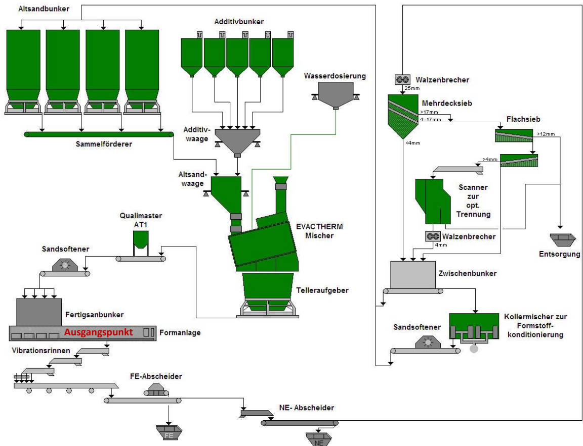
Bild 2.1: Prinzipskizze der neuen Sandaufbereitungsanlage mit Kennzeichnung der innovativen Anlagenelemente (grün gekennzeichnete Anlagenteile)
