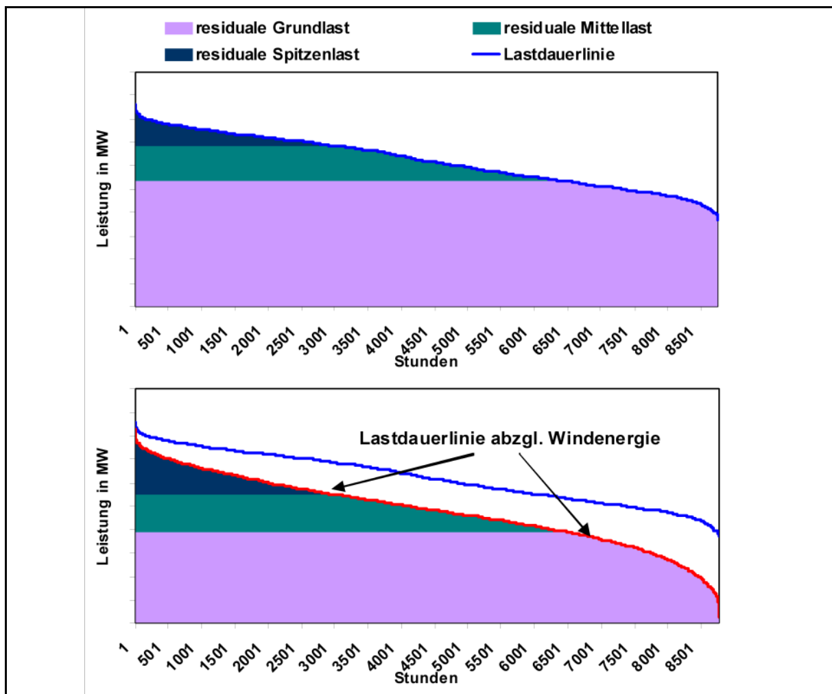
Abbildung 5-7: Veränderung der Lastdauerlinie durch Windenergieeinspeisung (BET [2008])
