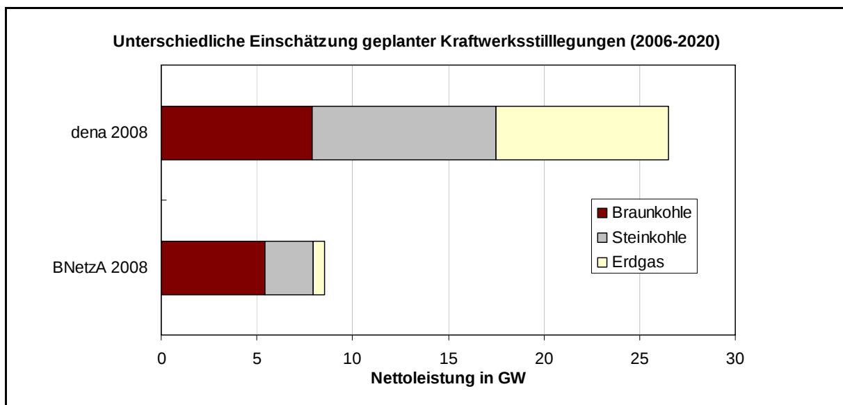
Abbildung 4-1: Vergleich der Stilllegungen nach der dena-Kurzanalyse mit den geplanten Stilllegungen der Kraftwerksbetreiber nach dem Monitoringbericht der Bundesnetzagentur zwischen 2006 und 2020 132 (eigene Darstellung)
