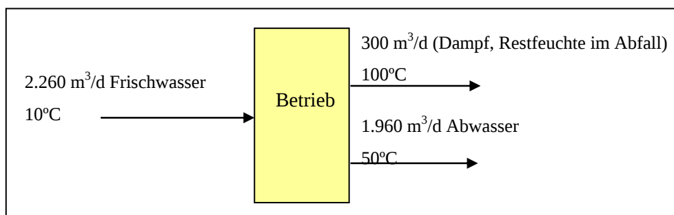
Abbildung 10: Vereinfachte Wasserbilanz einer Papierfabrik
