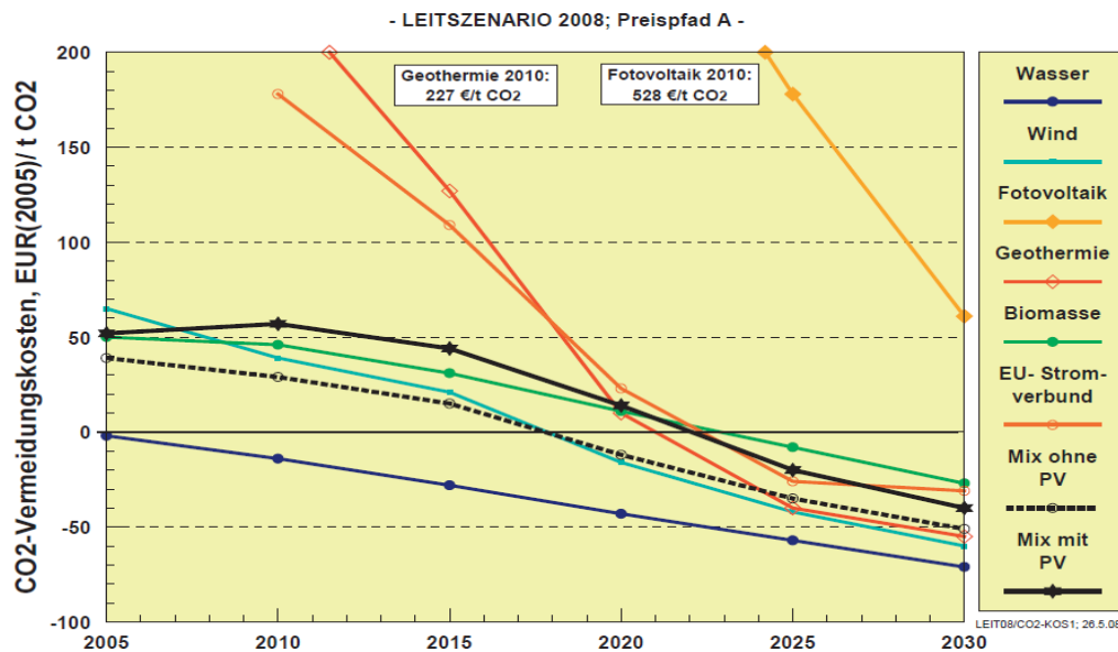
Abbildung 6: CO 2 -Vermeidungskosten erneuerbarer Energien 197
