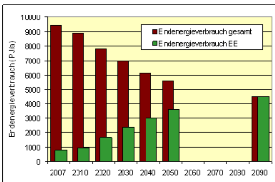
Abbildung 12: Notwendige Entwicklungen des Endenergieverbrauchs und der Anteil erneuerbarer Energien am Endenergieverbrauch bis zum Jahr 2090 242
