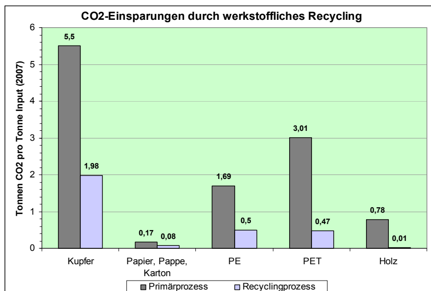
Abbildung 11: CO 2 -Einsparungen durch werkstoffliches Recycling
