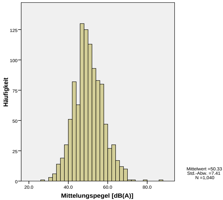
Abbildung 10.3-2: Verteilung der Mittelungspegel der Schallpegelmessung
