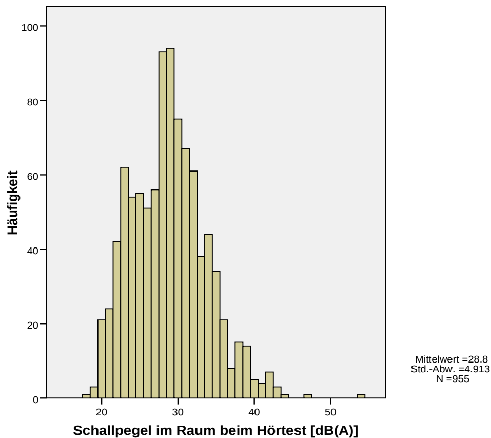
Abbildung 6.3-1: Verteilung der vorherrschenden Umgebungsschallpegel ( L_{AS} ) beim Hörtest (ungewichtet)
