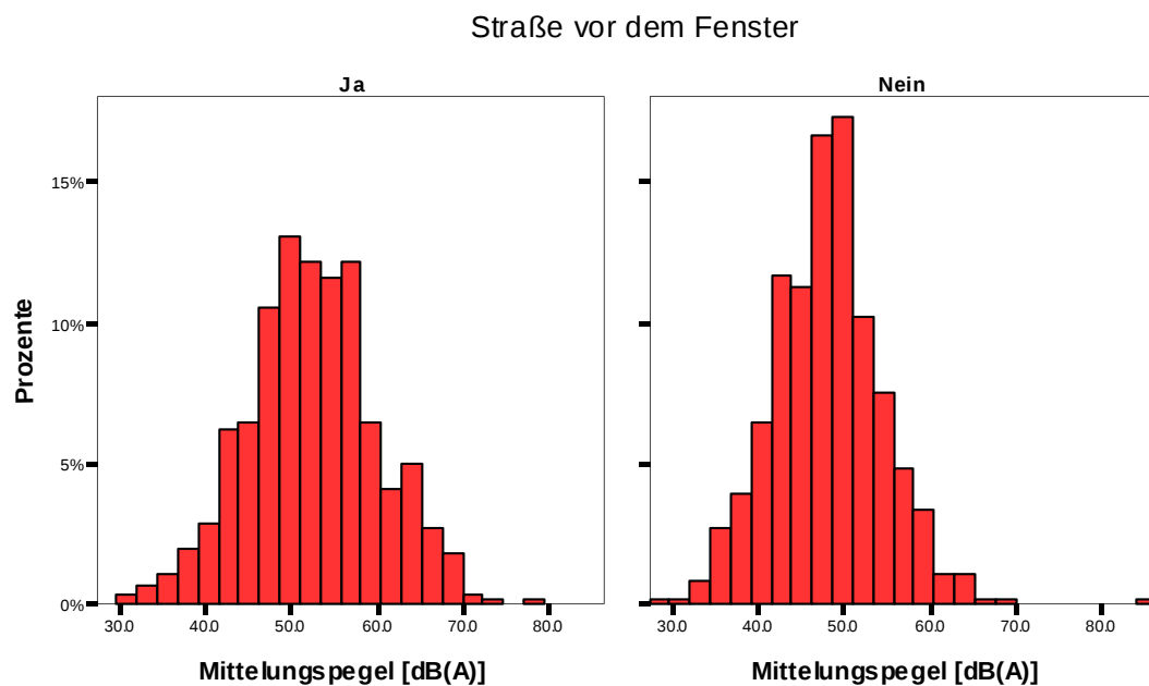
Abbildung 10.3-5: Verteilungen der Schalldruck-Mittelungspegel der Schallpegelmessung für Wohnungen mit (linkes Bild) und ohne (rechtes Bild) einer Straße vor dem Fenster (ungewichtete Daten)
