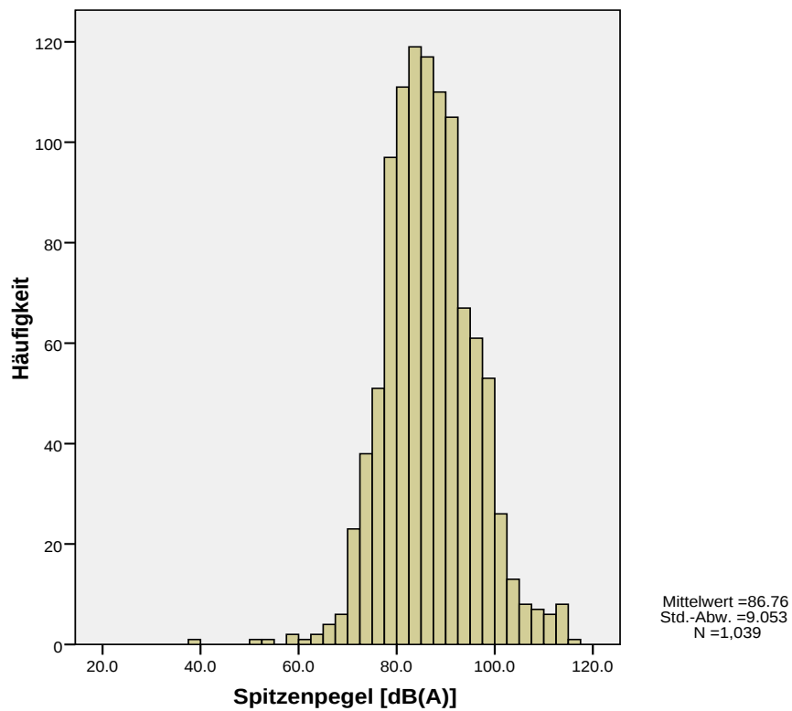
Abbildung 10.3-4: Verteilung der Spitzenpegel der Schallpegelmessung
