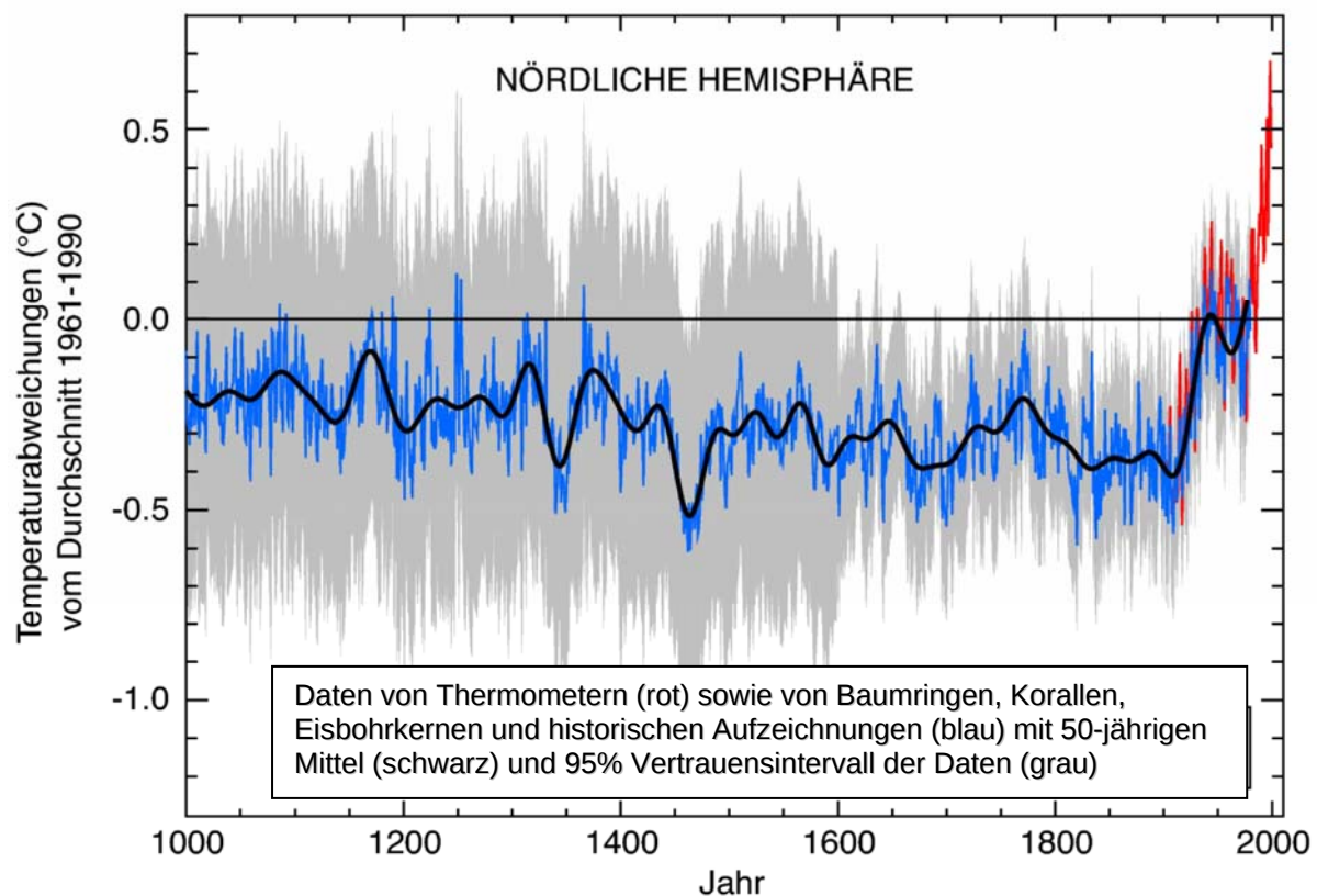
Abbildung: Historische Temperaturerhöhung der Nördlichen Hemisphäre in Form eines „Hockeyschlägers“. Quelle: IPCC, Klimaänderung 2001, Synthesebericht
