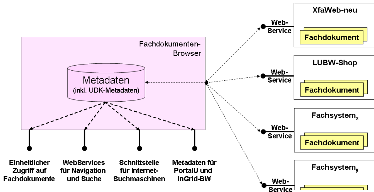
Abbildung 1: Der Fachdokumenten-Browser (FDB) als zentrale Zugangscomponente für Fachdokumente im UIS BW (XfaWeb-neu und LUBW-Shop stehen beispielhaft als Fachsysteme, die Fachdokumente enthalten).
