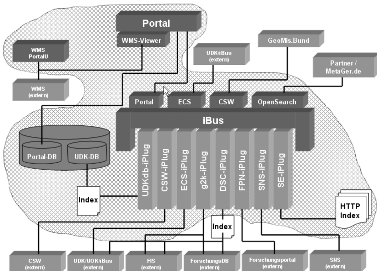
Abbildung 1: PortalU®/InGrid®-Softwarearchitektur.
