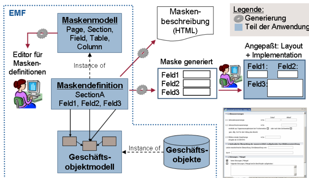
Abbildung 7: Modellbasierte Masken
