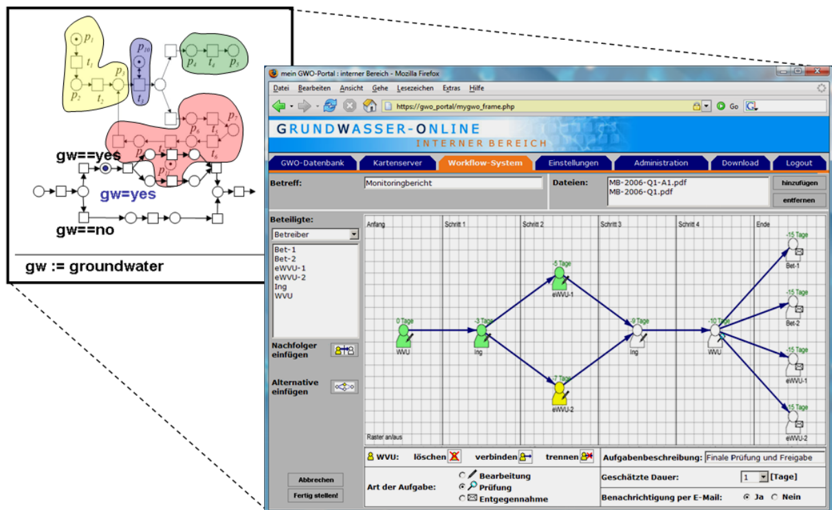
Abb. 7: Prozessbasiertes Notifikationsmanagement
