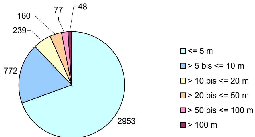
Abbildung 5.25: Ausbaufallhöhen der Wasserkraftanlagen in Bayern
