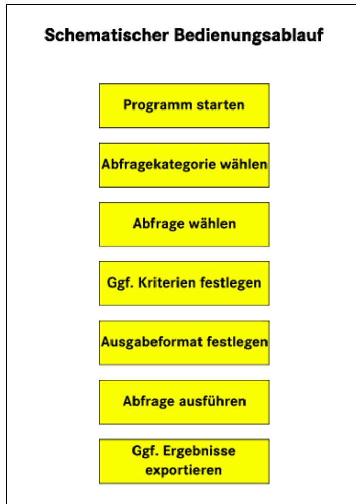
Abbildung 4.1: Typischer Programmablauf
