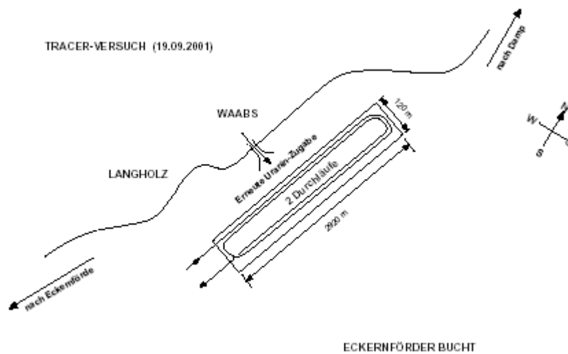
Abb. 8 Beprobungsschema vom 19.09.2001
