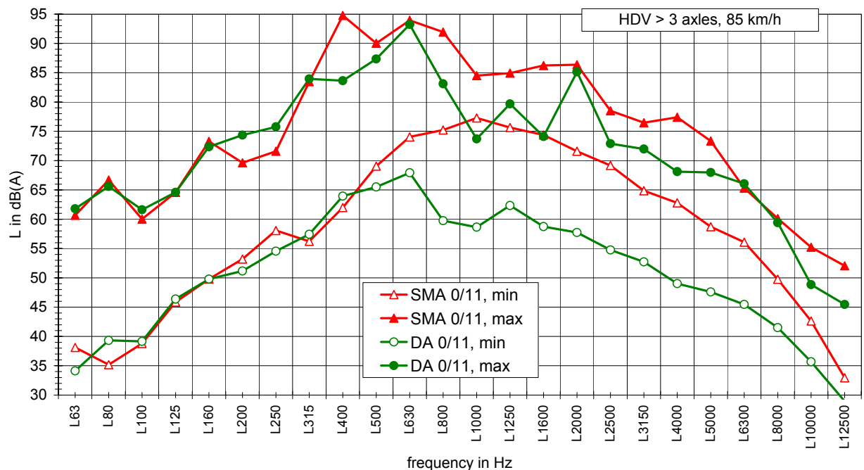
Bild 73: untere und obere Begrenzung der Frequenzspektren von sNfz an Autobahn-messstellen mit Splittmastixasphalt und Drainasphalt Belag (beide mit 11 mm maximale Korngröße)
