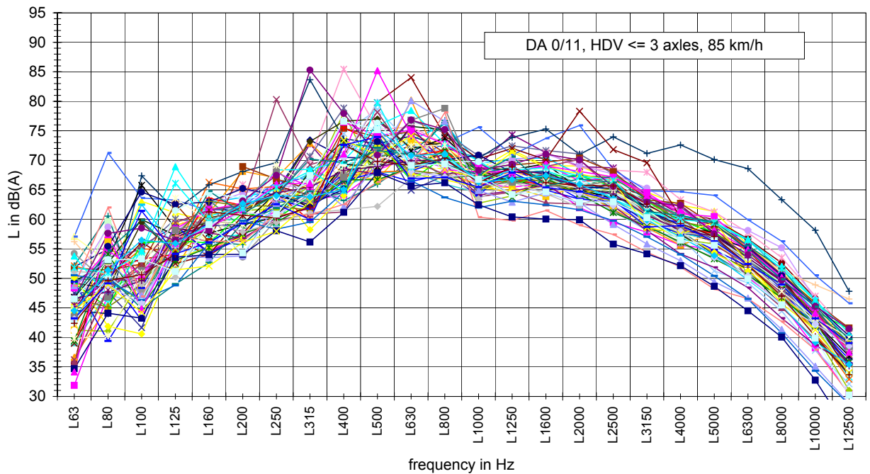
Bild 69: Frequenzspektren von sNfz mit mehr als 3 Achsen auf einer Autobahnmessstelle mit Drinasphalt (mit 11 mm maximale Korngröße)
