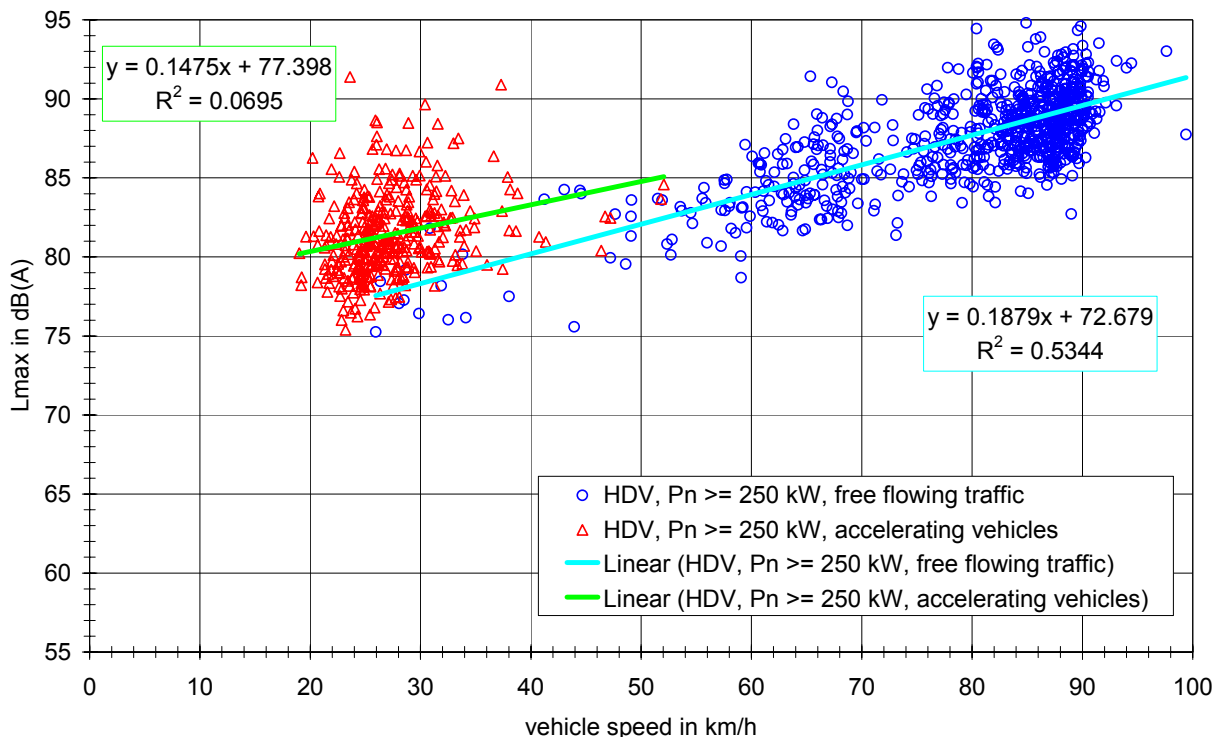
Bild 11: L_{max} Werte für sNfz mit Nennleistungen von 250 kW oder mehr gegen Fahrzeuggeschwindigkeit auf Asphaltbeton 0/11 oder Splittmastix 0/11 für frei fließenden Verkehr und für beschleunigende Fahrzeuge.
