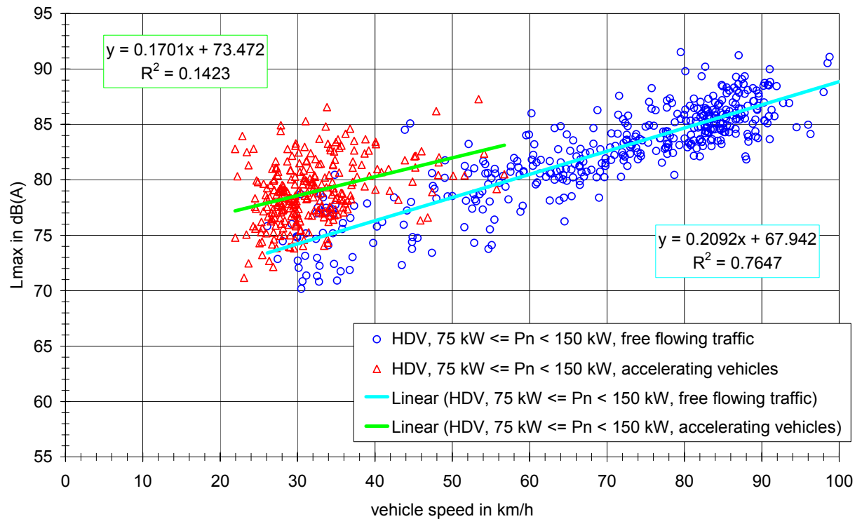
Bild 9: L_{max} Werte für sNfz mit Nennleistungen von 75 kW oder mehr, jedoch unter 150 kW gegen Fahrzeuggeschwindigkeit auf Asphaltbeton 0/11 oder Splittmastix 0/11 für frei fließenden Verkehr und für beschleunigende Fahrzeuge.
