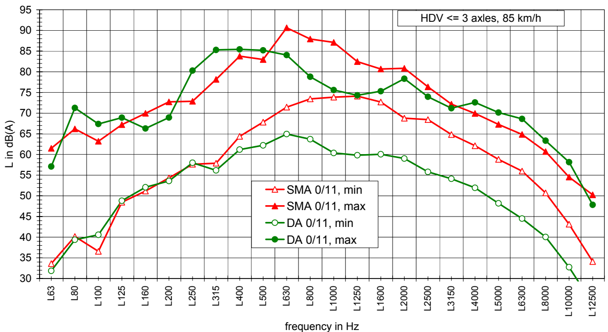
Bild 70: untere und obere Begrenzung der Frequenzspektren von sNfz mit bis zu 3 Achsen an Autobahnmessstellen mit Splittmastixasphalt und Drinasphalt Belag (beide mit 11 mm maximale Korngröße)
