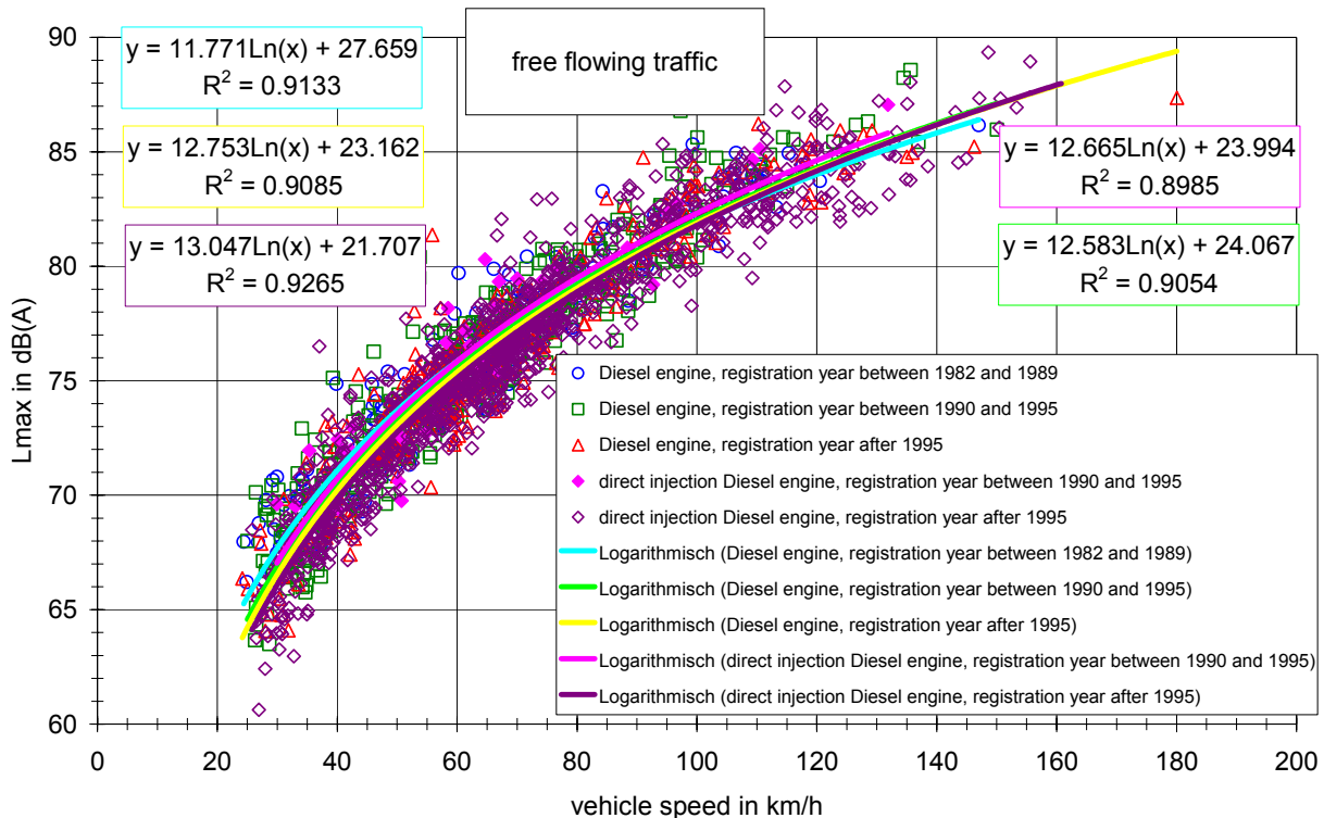
Bild 33: Vorbeifahrtpegel von Pkw im frei fließenden Verkehr mit Dieselmotoren und verschiedenen Zulassungsjahren
