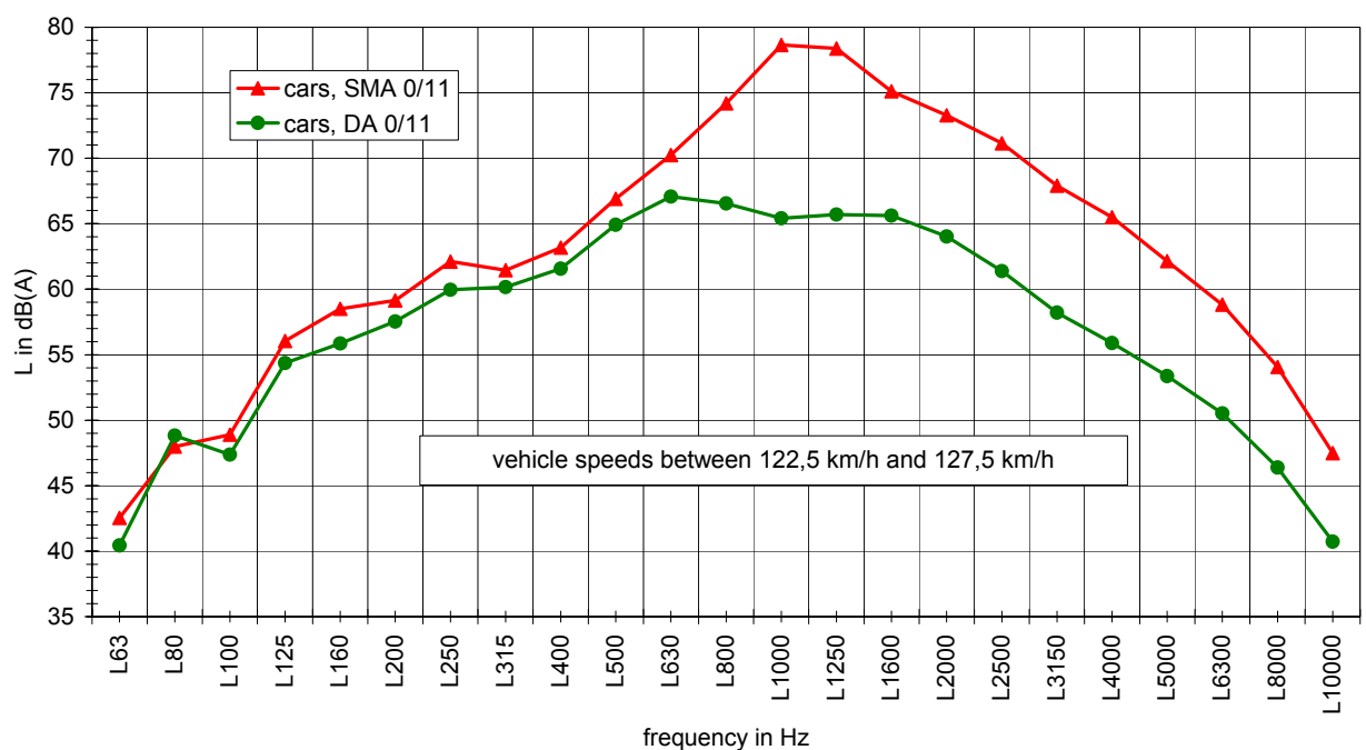
Bild 62: mittlere Frequenzspektren von Pkw auf Autobahnmessstellen mit Drainasphalt und Splittmastixasphalt (beide mit 11 mm maximale Korngröße)
