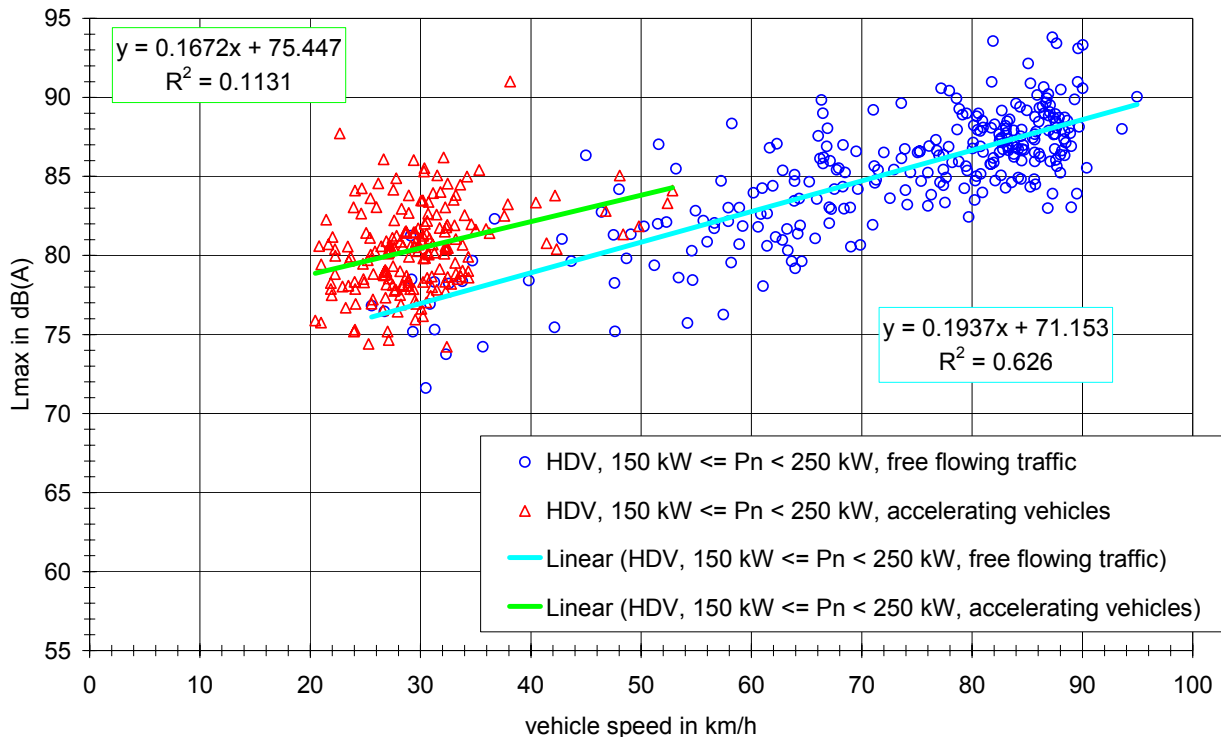
Bild 10: L_{max} Werte für sNfz mit Nennleistungen von 150 kW oder mehr, jedoch unter 250 kW gegen Fahrzeuggeschwindigkeit auf Asphaltbeton 0/11 oder Splittmastix 0/11 für frei fließenden Verkehr und für beschleunigende Fahrzeuge.
