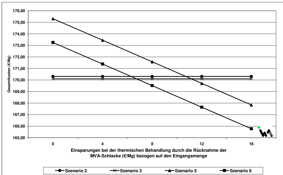
Bild 12-5: Gesamtkosten in Abhängigkeit von Einsparungen bei der thermischen Abfallbehandlung durch die Rücknahme der MVA-Schlacke
