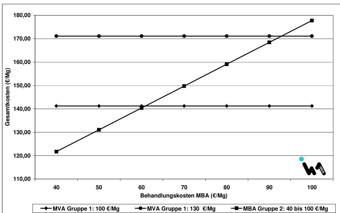
Bild 12-8: Gesamtkosten in Abhängigkeit der Kosten der mechanisch-biologischen Abfallbehandlung (MBA-Behandlungskosten bei Erzeugung einer heizwertreichen Fraktion, ohne Entsorgungskosten)
