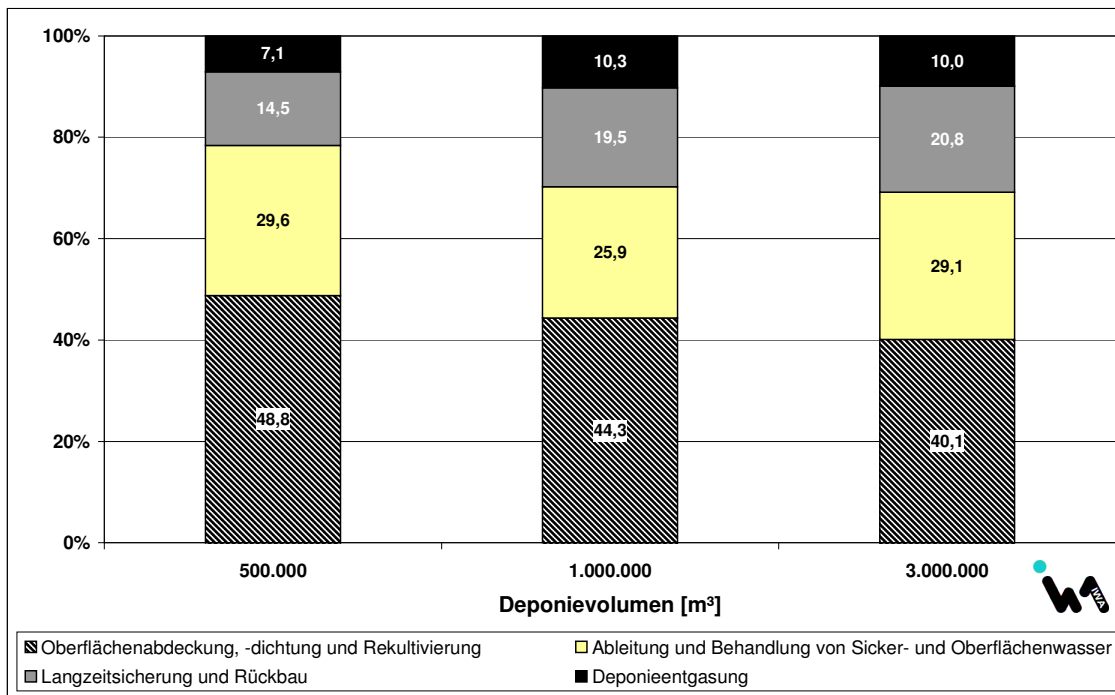
Bild 9-4: Prozentuale Verteilung der Nachsorgekosten
