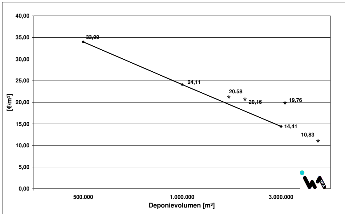
Bild 9-1 Spezifische Investitionskosten in Abhängigkeit vom Deponievolumen ([52], IWA, 2002; [53], Auksutat & Löffler, 1998), (Netto)
