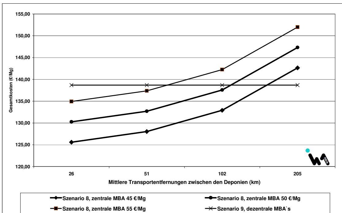
Bild 12-6: Gesamtkosten in Abhängigkeit der Transportentfernungen zwischen den Deponien
