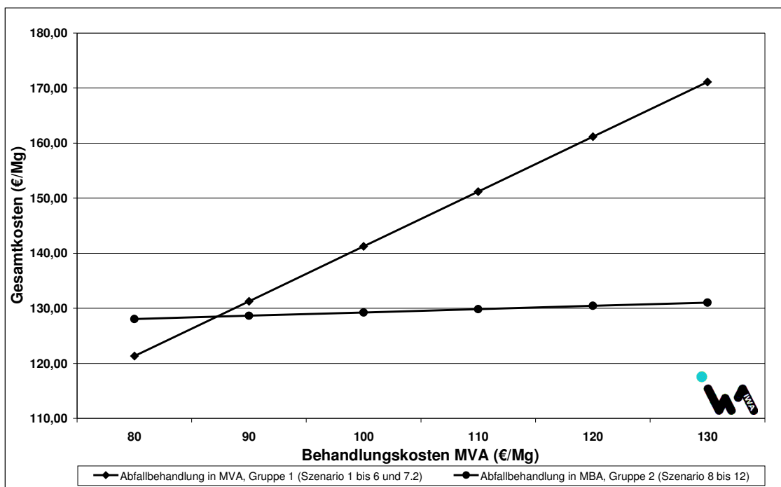
Bild 12-7: Gesamtkosten in Abhängigkeit der Kosten der thermischen Abfallbehandlung (MBA-Behandlungskosten bei Erzeugung einer heizwertreichen Siebfraktion)
