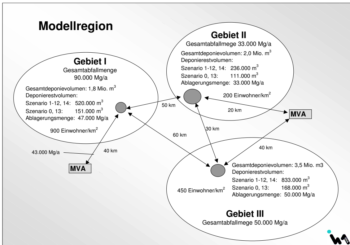
Bild 12-1: Darstellung der modifizierten Randbedingungen der Modellregion (Region B gemäß Kap. 11.2.2)
