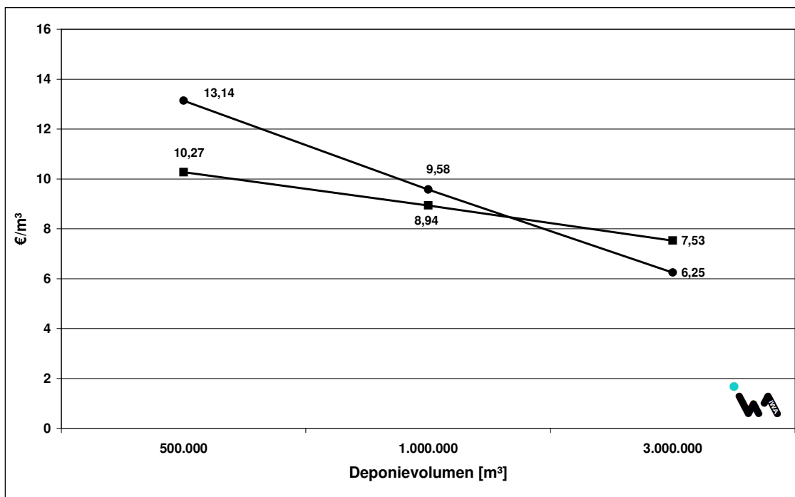
Bild 9-5: Nachsorgekosten in Abhängigkeit des Deponievolumens ([52], IWA, 2002; [53], Auksutat & Löffler, 1998)
