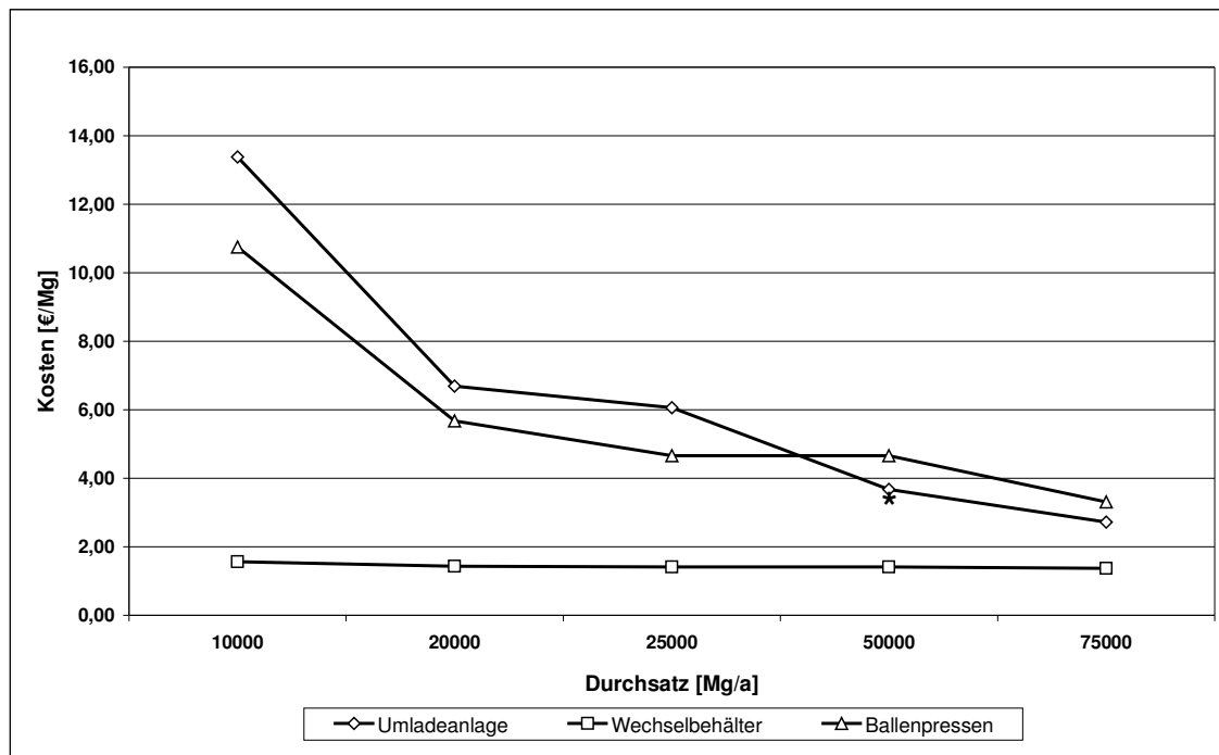
Bild 9-10 Umladekosten in Abhängigkeit der Durchsatzleistung und Umladeart ([57], Würz, 2000)
