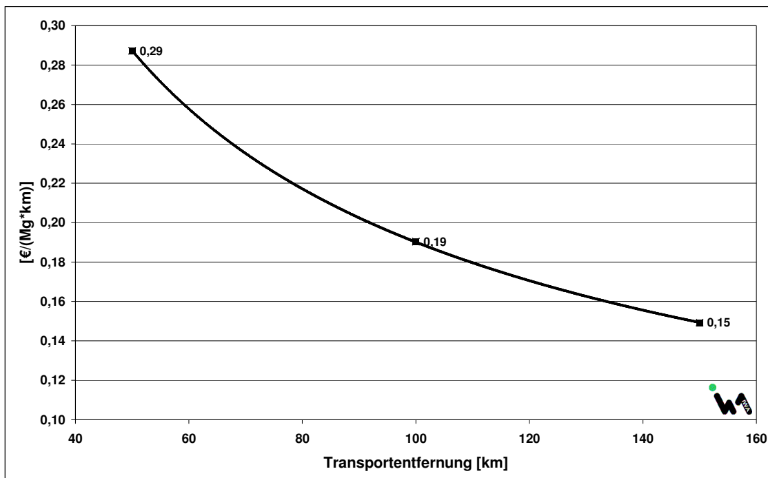
Bild 9-11: Spezifische Transport-/Umladekosten in Abhängigkeit der Transportentfernung, (Netto)
