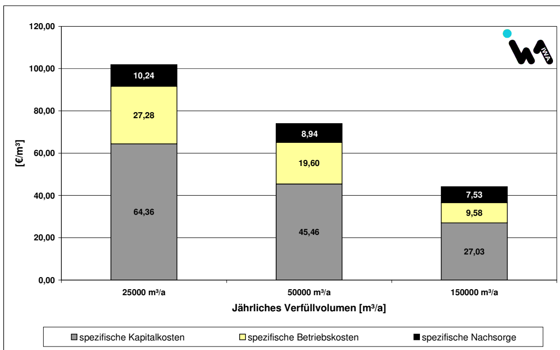
Bild 9-6: Darstellung der spezifischen Deponiekosten, (Netto)
