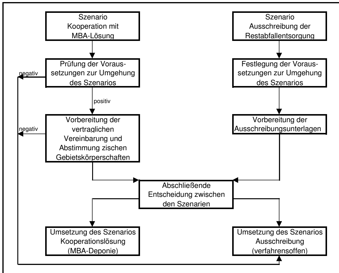
Bild 13-3: Ablaufschema zur Umsetzung eines Entsorgungskonzeptes zur Restabfallentsorgung
