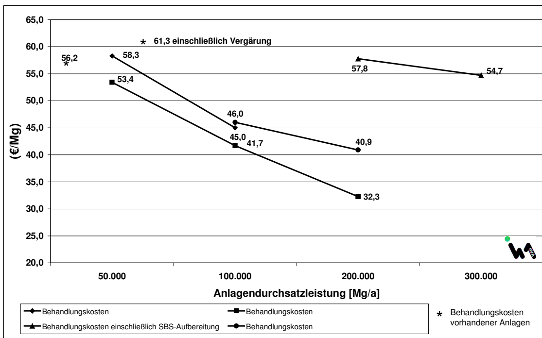
Bild 9-9: Darstellung spezifischer Behandlungskosten von mechanisch-biologischen Abfallbehandlungsanlagen ([41], Kost, 1998; [49], NN, 2000; [53], Auksutat & Löffler, 1998; [54], Dahm, Kollbach und Gebel, 1994), (Netto)
