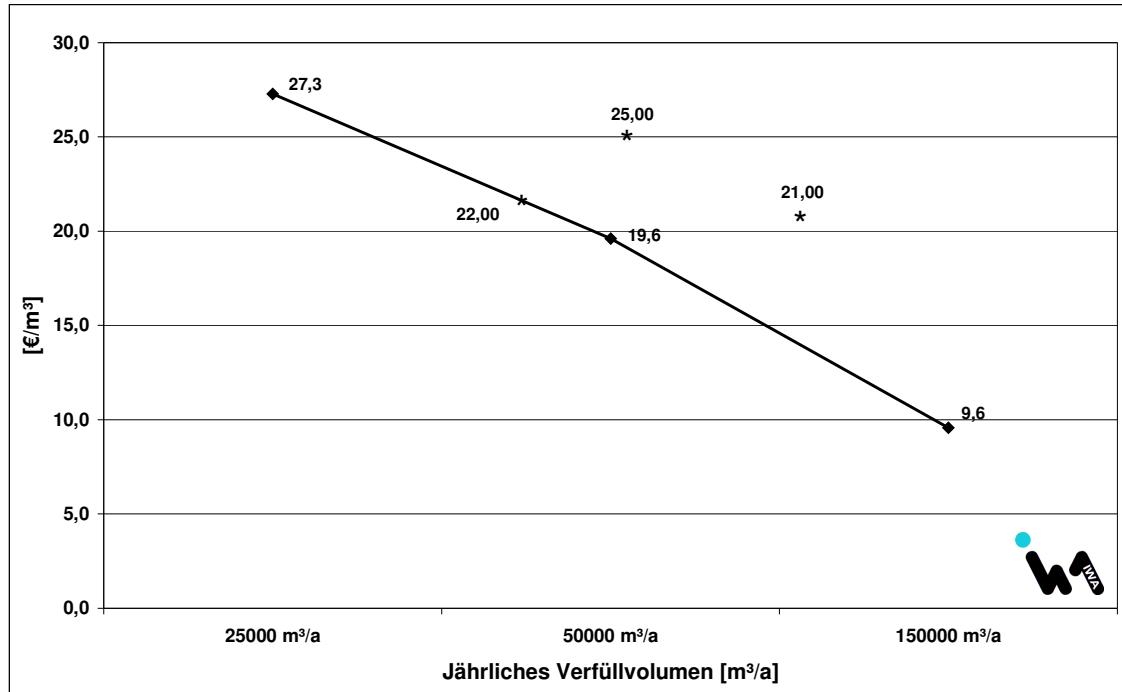
Bild 9-3: Darstellung der spezifische Betriebskosten in Abhängigkeit des jährlichen Verfüllvolumens einschließlich im Betrieb befindlicher Deponien (*[52], IWA, 2002)
