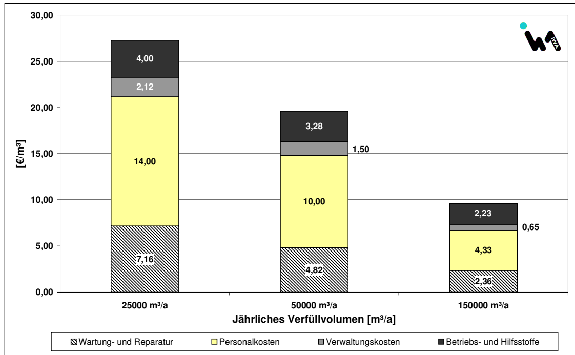
Bild 9-2: Darstellung der berechneten spez. Betriebskosten in Abhängigkeit des jährlichen Verfüllvolumens
