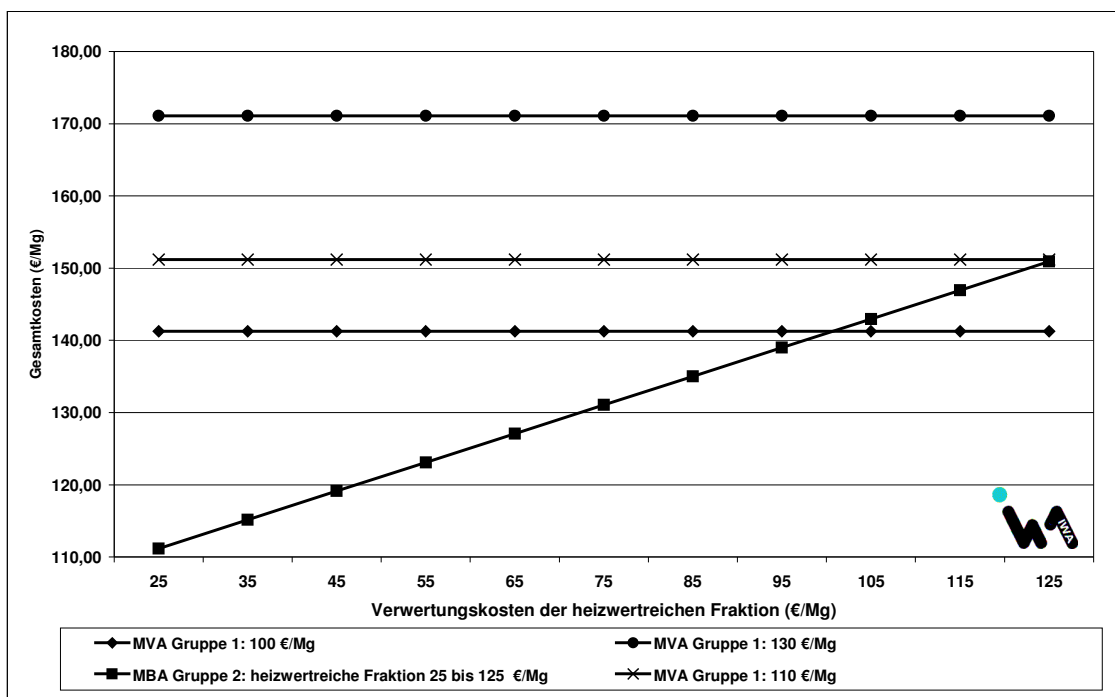
Bild 12-9: Gesamtkosten in Abhängigkeit der Kosten der Verwertung der heizwertreichen Fraktion der MBA (MBA-Behandlungskosten bei Erzeugung einer heizwertreichen Siebfraction)
