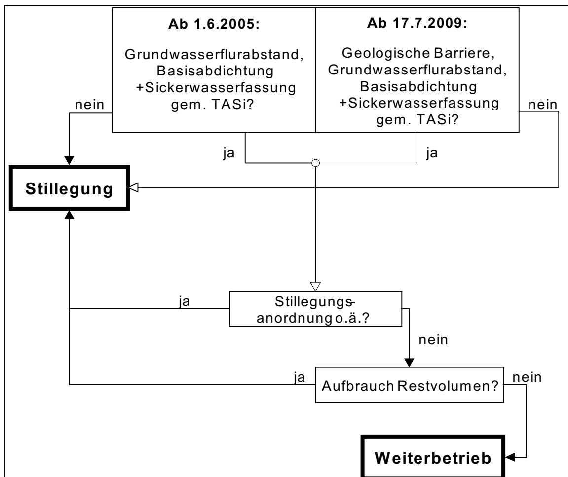
Bild 4-1: Auswahlschema Weiterbetrieb oder Stillegung
