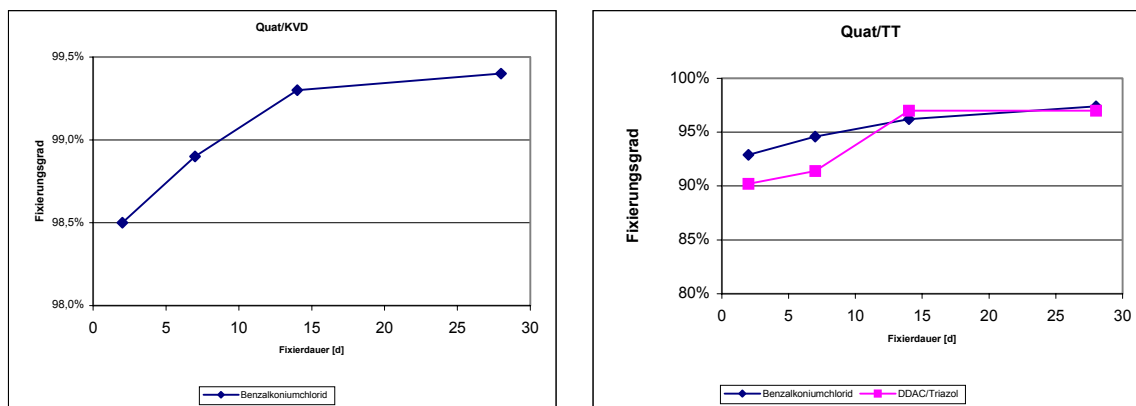
Abbildung 3: Fixierungsverlauf von quartären Ammoniumverbindungen aus einem Quat-Produkt und einem Quat/Triazol-Präparat nach Vakuum- bzw. Trogrückung (Daten zur Fixierung bei 20 °C)
