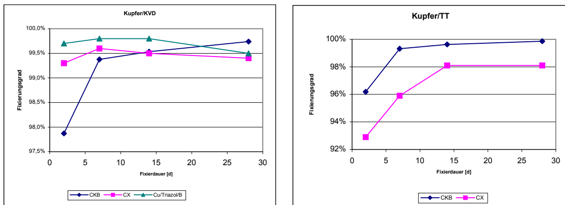
Abbildung 1: Fixierungsverlauf von Kupfer aus CKB-, Kupfer-HDO und Kupfer/Triazol/Bor-Präparaten nach Vakuum- bzw. Trogrtränkung (Daten zur Fixierung bei 20 °C)
