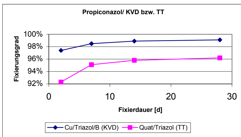
Abbildung 4: Fixierungsverlauf von Propiconazol aus einem Kupfer/Triazol/Bor- und einem Quat/Triazol-Präparat nach Vakuum- bzw. Trogrückung (Daten zur Fixierung bei 20 °C)
