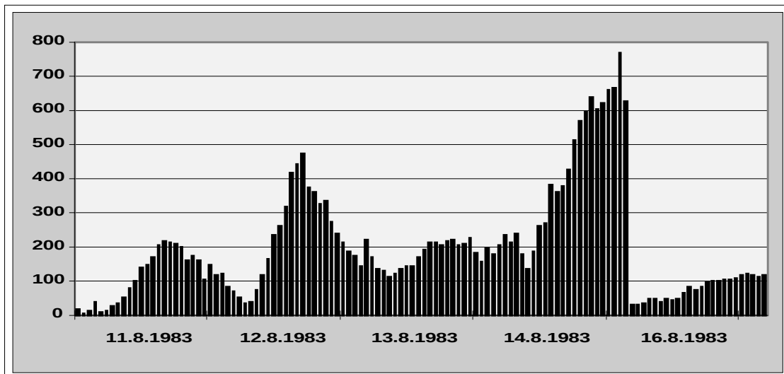
Abb. 09) Fehlerhaft berechnete Schätzwerte im Datenkollektiv der Station FICHTELBERG (SN053, Met. Dienst DDR)
