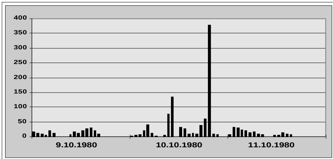
Abb. 13) Ausreißer im Datenkollektiv der Station KARLSRUHE-MITTE (BW001)
