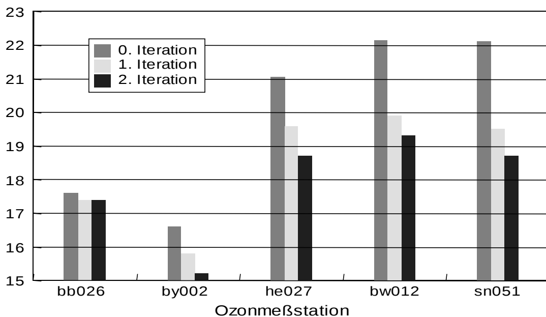
Abb. 103) Restreuung nach Wetterbereinigung als Mittel über 470 Stationen, 1990 bis 1997, April bis September, 5-stündiges Mittel (13 - 17 Uhr)
