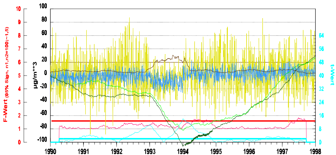
Abb. 84) Sensitivität um 30% reduziert und systematische Abweichung von -10 \mu\text{g}/\text{m}^3 im Jahr 1993 sowie ein Trend von +2 \mu\text{g}/\text{m}^3 pro Jahr
