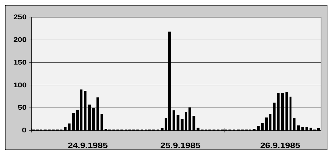
Abb. 43) Nicht plausible Werte an der Station KARLSRUHE-WEST (BW002)
