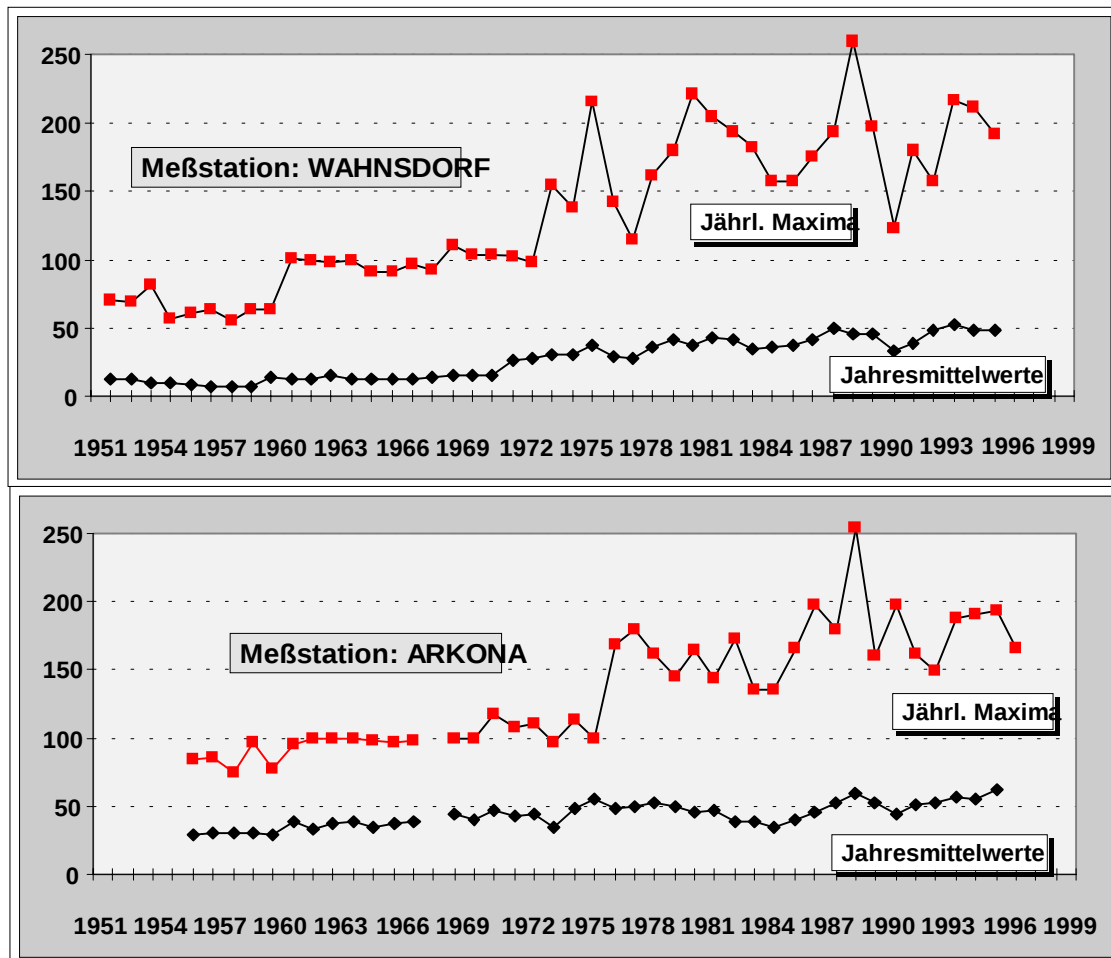
Abb. 11) Änderungen in der Messtechnik bewirken stufenförmige Interventionen in den Messreihen von ARKONA und WAHNSDORF (MV013 und SN051, Met. Dienst der DDR)
