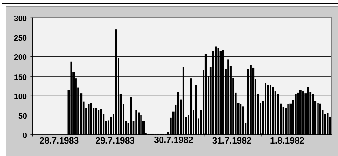
Abb. 28) Nicht plausible Messwerte an der Station MANNHEIM-SÜD (BW007)
