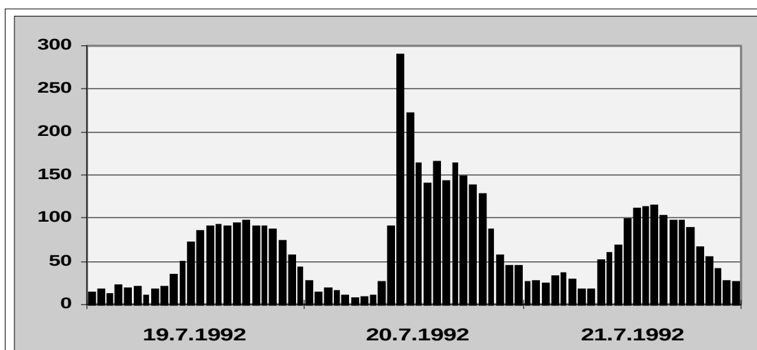
Abb. 73) Der HÜRTH-EFFEKT im Juli 1992 an der Messstation HÜRTH bei Köln (NW058)
