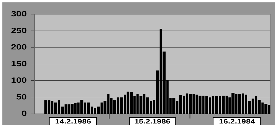
Abb. 50) Ausreißer oder Kalibrierwerte? Nicht plausible Werte an der Station ARZBERG (BY002), 15.2.1986
