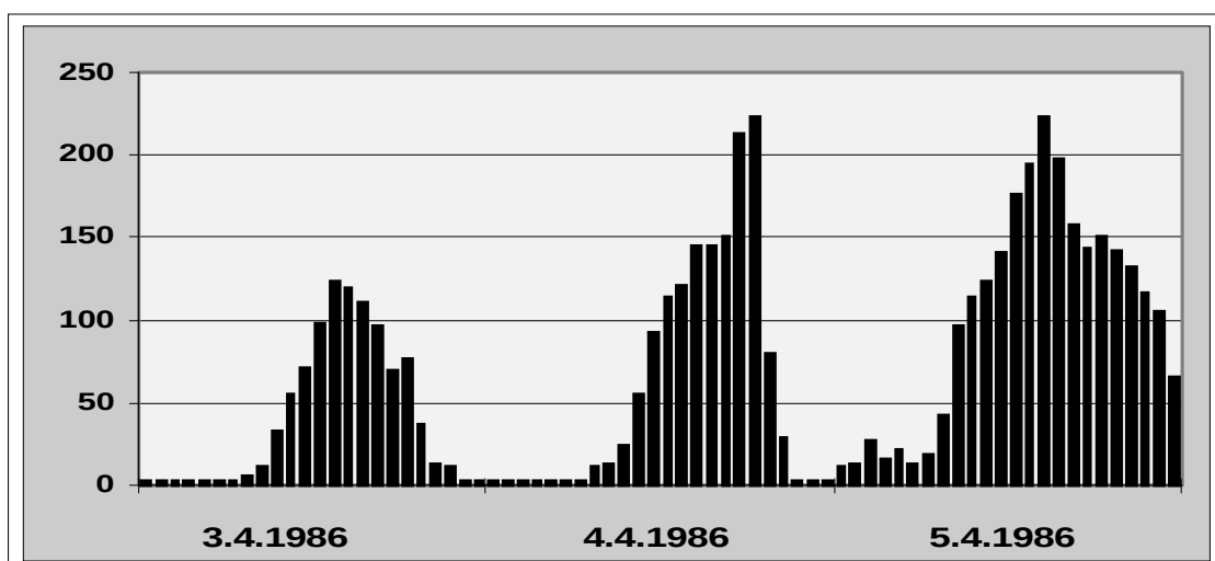
Abb. 52) HÜRTH-EFFEKT an der Station TRIER (RP020). Die Werte werden noch als plausibel angesehen
