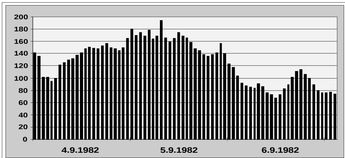
Abb. 27) Fragwürdige, aber nicht unplausible Werte an der Station SCHMÜCKE (UB029) im September 1982
