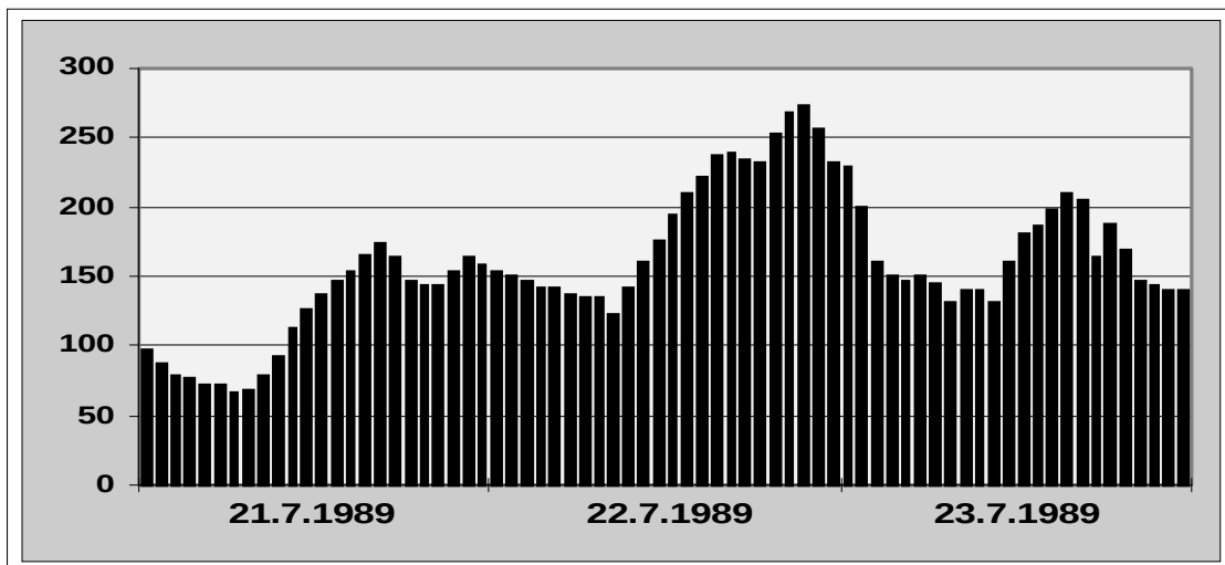
Abb. 65) Station WESTERWALD (RP016): Der kritisierte Messwert ist als plausibel einzustufen
