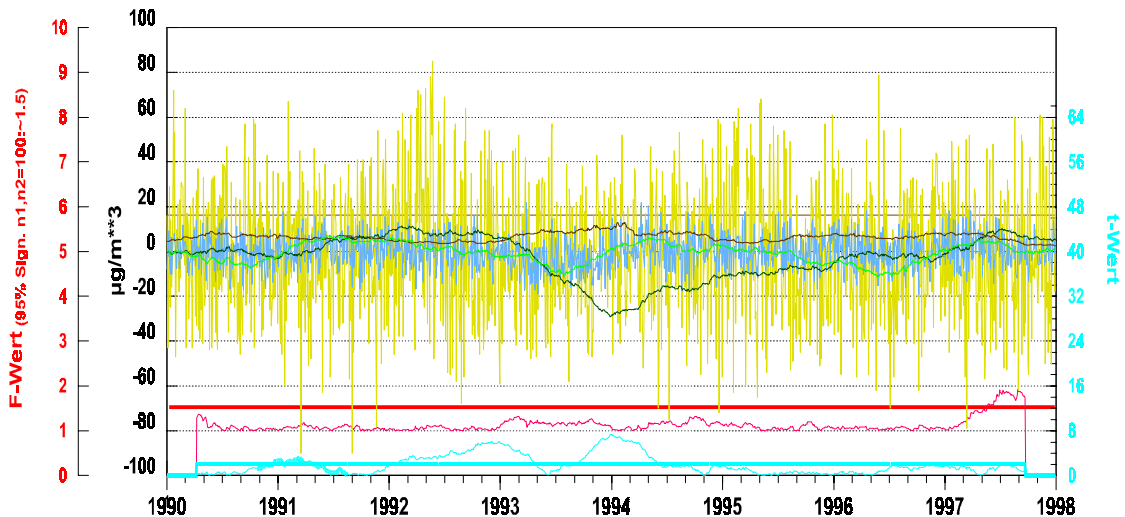
Abb. 85) Systematische Abweichung im stärksten Prediktor im Jahr 1993 (+10 \mu\text{g}/\text{m}^3 )
