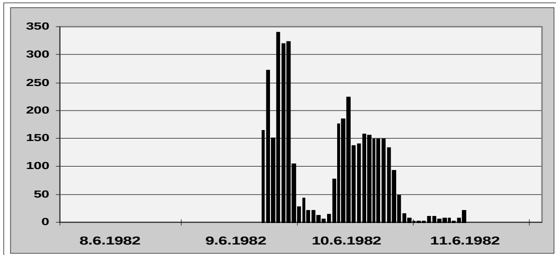
Abb. 23) Nicht plausible Messwerte an der Station ZUFFENHAUSEN (BW011)
