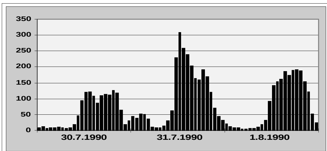
Abb. 70) Noch ein Beispiel für den HÜRTH-EFFEKT an der Messstation HÜRTH (NW058) ebenfalls im Juli 1990
