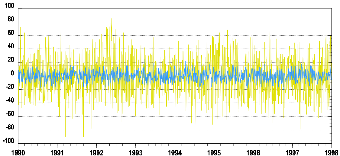
Abb. 74) Zeitreihe der Originalwerte (normal verteilte Zufallsfolge = gelbe Kurve) und der Differenz zwischen den Originalwerten und den Erwartungswerten (blaue Kurve)
