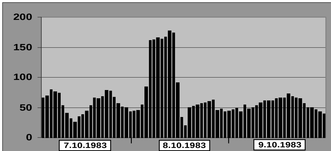
Abb. 34) Fehlerhaft geschätzte Messwerte an der Station NEUGLOBSOW (UB030)
