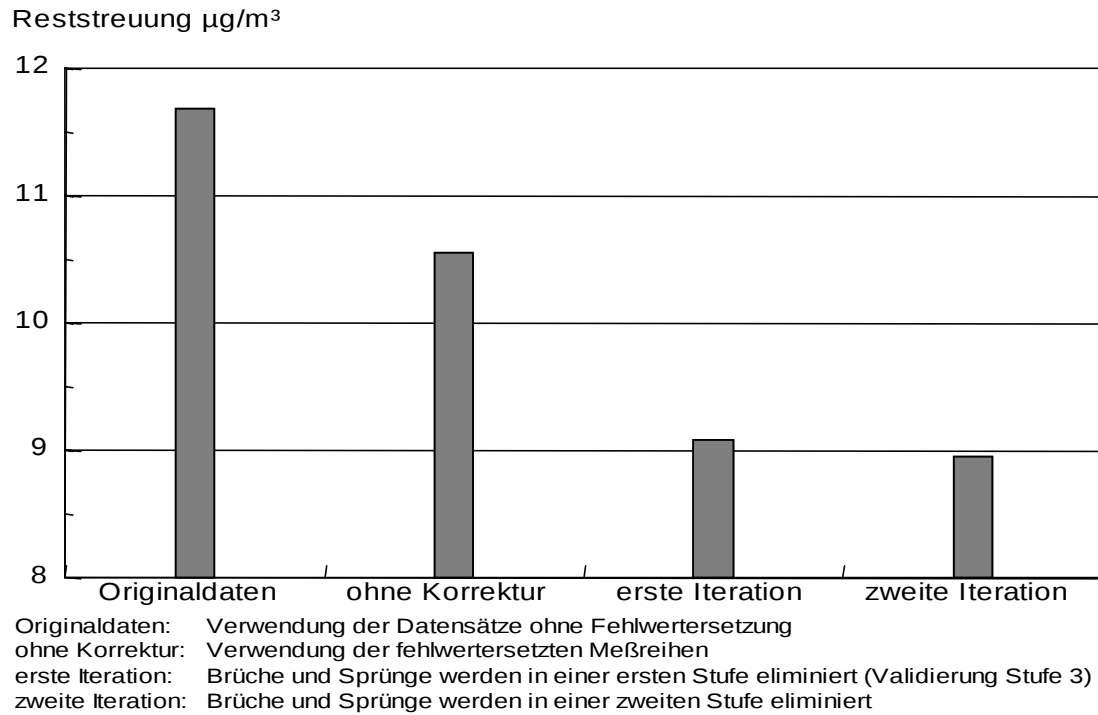
Abb. 101) Gewichtete mittlere Reststreuung bei kompletter Fehlwertersetzung als Mittel über 470 Stationen, 1990 bis 1997, April bis September, 5-stündiges Mittel (13 - 17 Uhr)
