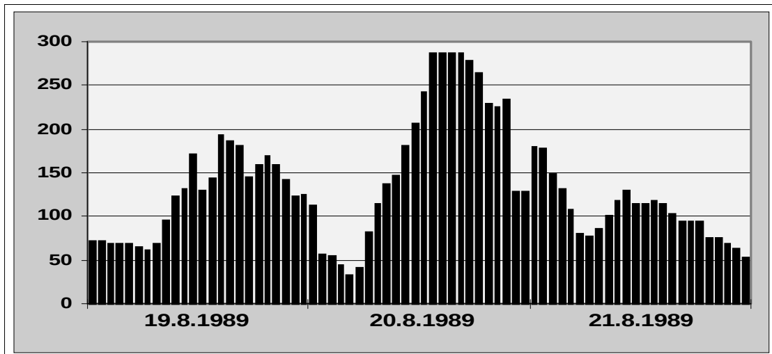
Abb. 67) Plausibel oder nicht plausibel? Fragwürdige Werte an der Station LINDENBERG (UB025)
