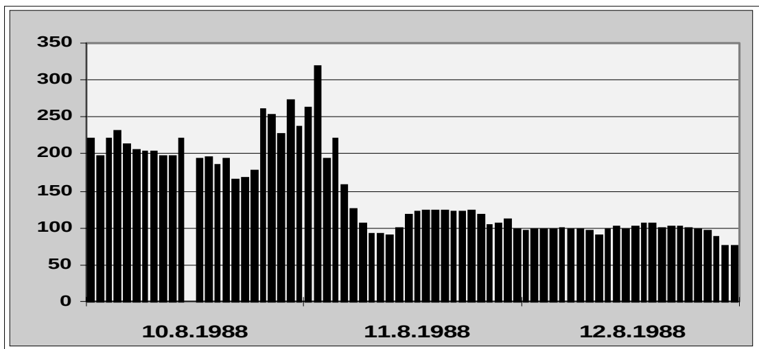
Abb. 59) Plausibel oder nicht plausibel? Fragwürdige Werte an der Station PFÄLZERWALD (RP017)
