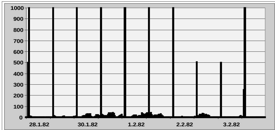
Abb. 01) Das Datenkollektiv der Station Nürnberg (BY053) enthält Kalibrierwerte
