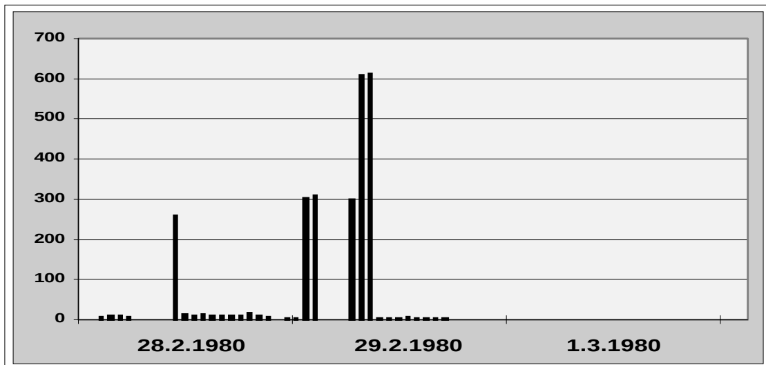
Abb. 05) Kalibrierwerte? Nicht plausible Messwerte an der Station HEILBRONN (BW015)
