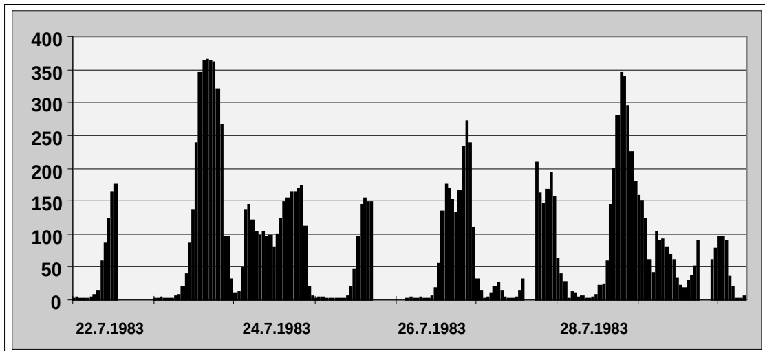
Abb. 29) Nicht plausible Messwerte in einem insgesamt nicht plausiblen Datenkollektiv der Station STUTTGART-HAFEN (BW014)
