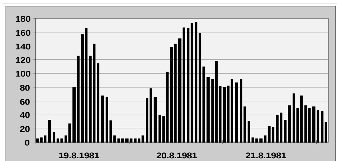
Abb. 18) Als fragwürdig bezeichnete Werte sind offensichtlich plausibel, Station MÜNCHEN-EFFNERPLATZ (BY038)
