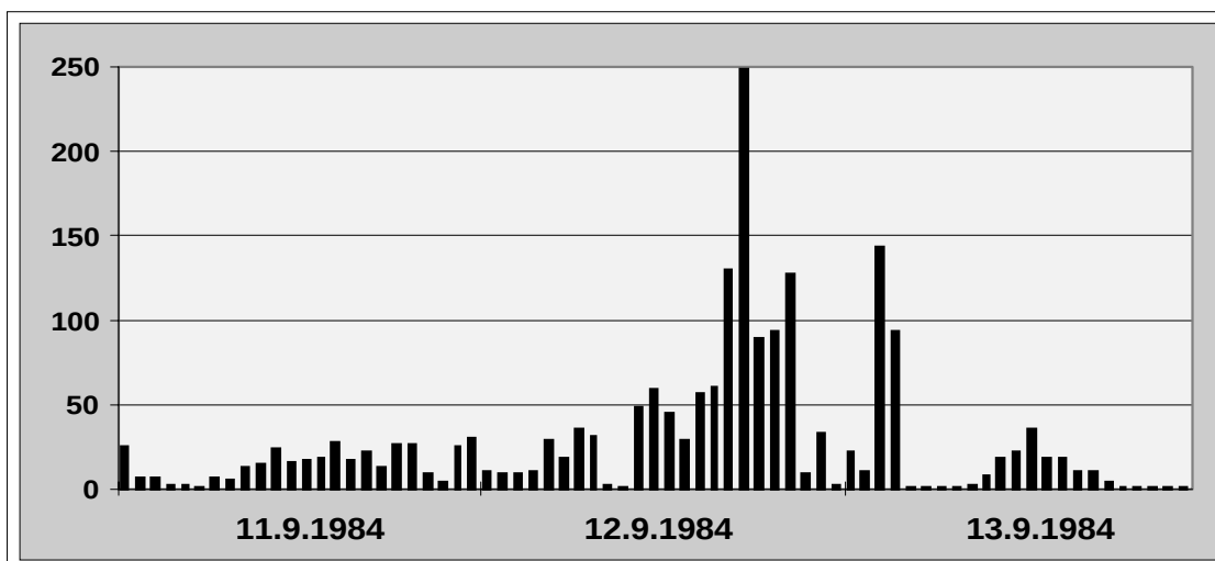
Abb. 40) Nicht plausible Ausreißer an der Station MANNHEIM-NORD (BW005) im Monat September 1984
