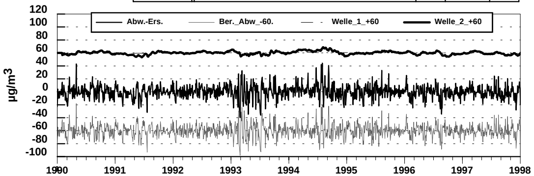
Abb. 99: Validierung der Ozon- Meßreihe BW048 - Stuttgart vor- und nach der Bereinigung von Strukturbrüchen, April bis September, 5-stündiges Mittel (13 bis 17 Uhr)
