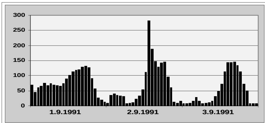
Abb. 71) Der HÜRTH-EFFEKT im September 1991 an der Messstation HÜRTH bei Köln (NW058)
