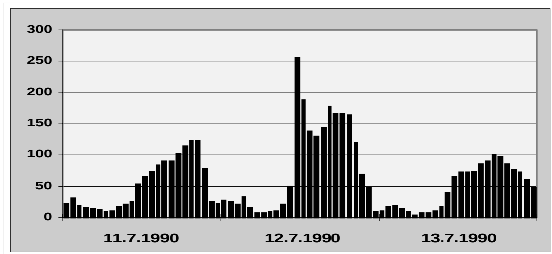
Abb. 69) Ein weiteres Beispiel für den HÜRTH-EFFEKT an der Messstation HÜRTH (NW058) im Juli 1990
