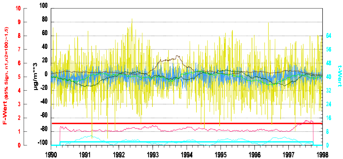
Abb. 82) Beispiel für das beschriebene “Sensitivitätsmaß der Varianz”
