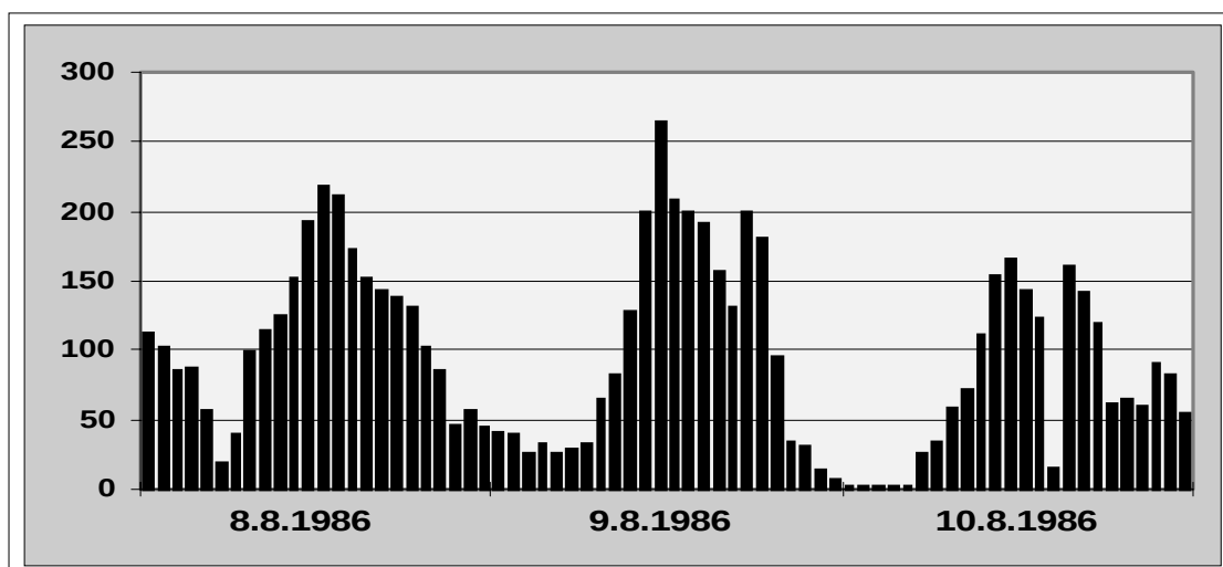
Abb. 48) Ausreißer oder HÜRTH-EFFEKT? Fragwürdige, aber noch plausible Werte in KEHL-HAFEN (BW022)
