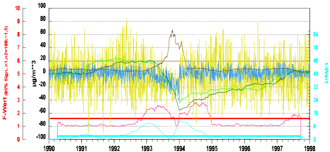
Abb. 86) Zunehmende systematische Abweichung bis - 18 \mu\text{g}/\text{m}^3 und Sensitivität abnehmend auf – 50%, beides im Jahr 1993
