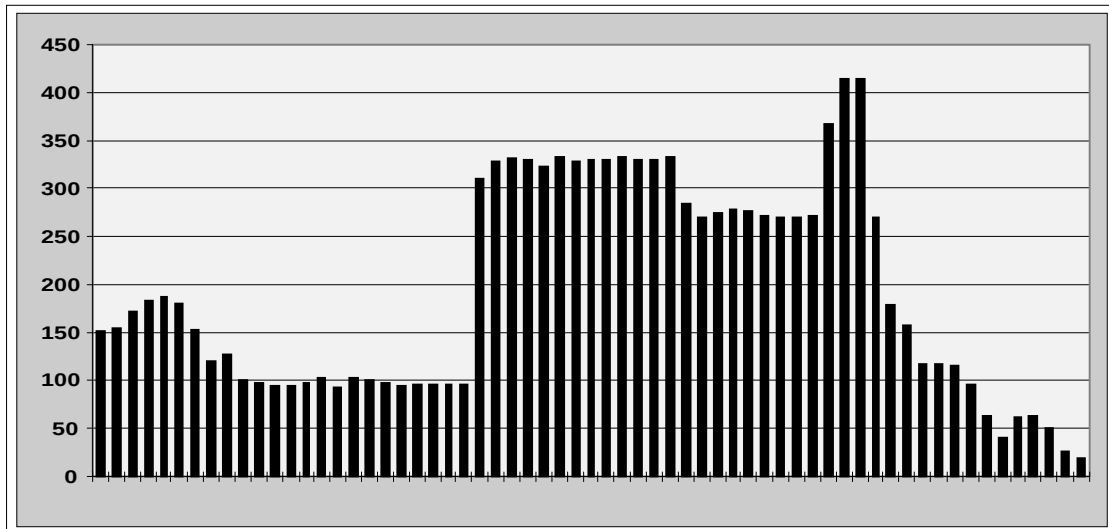
Abb. 02) Nicht plausible Messwerte im Datenkollektiv der Station MANNHEIM-NORD (BW005)
