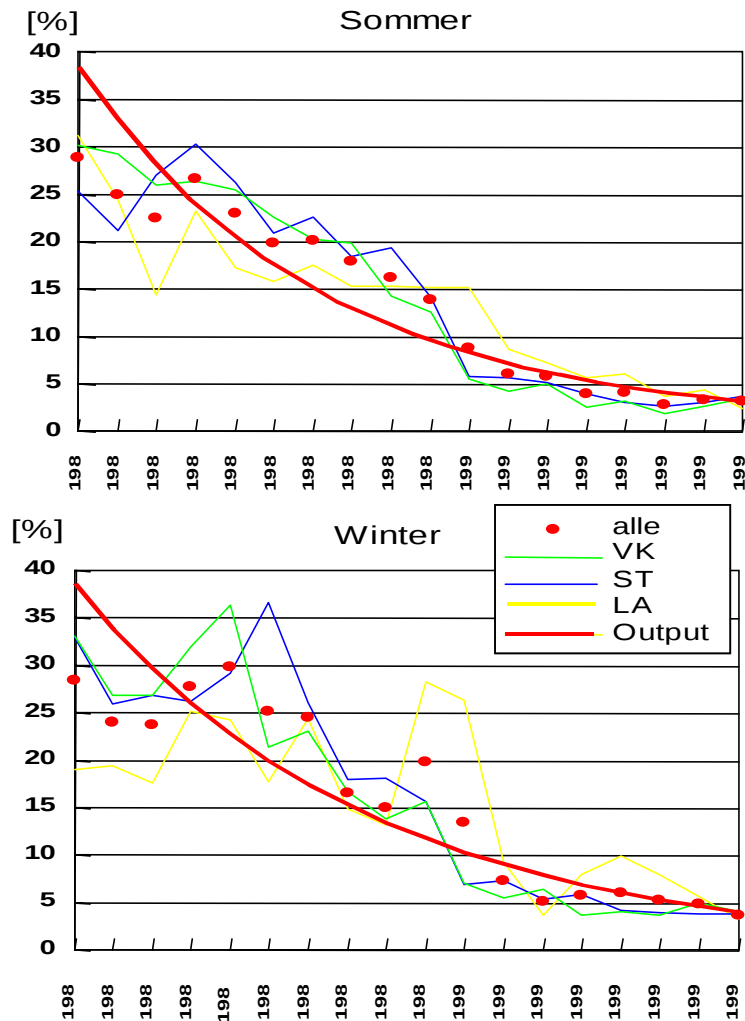
Abb. 104) Approximierter Messfehler, abgeschätzt aus dem Verhältnis der Streuung von LIMBA21 zu LIMBA26 im zeitlichen Verlauf als Mittel über alle Stunden
