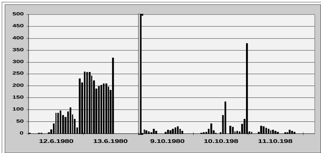
Abb. 04) Wie oben, zusätzlich eine einzelne nicht plausible Spitze im Oktober, KARLSRUHE-MITTE (BW001)
