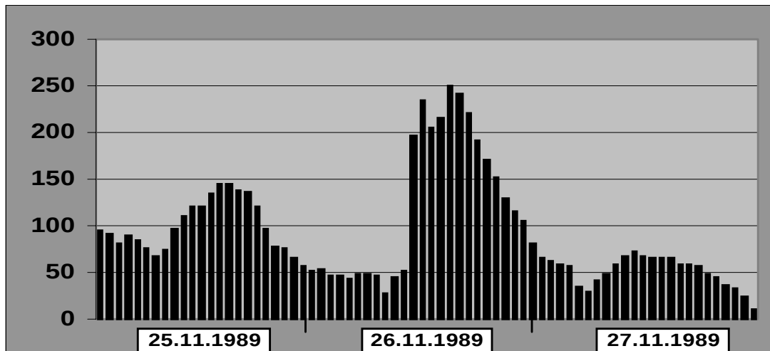
Abb. 63) Fehlerhaft berechnete Schätzwerte an der Station NEUGLOBSOW (UB030)
