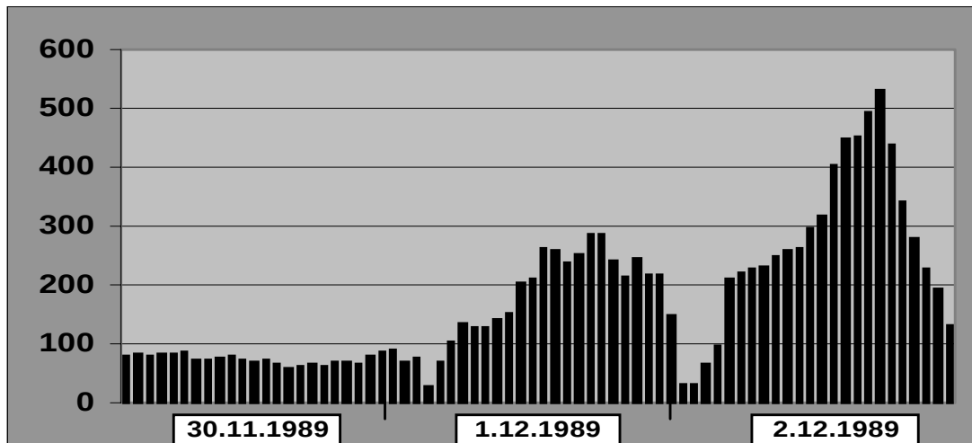
Abb. 62) Fehlerhaft berechnete Schätzwerte an der Station SCHMÜCKE (UB029)
