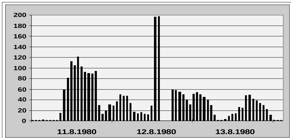
Abb. 12) Ausreißer oder Kalibrierwerte? Nicht plausible Werte an der Station KARLSRUHE-MITTE (BW001)
