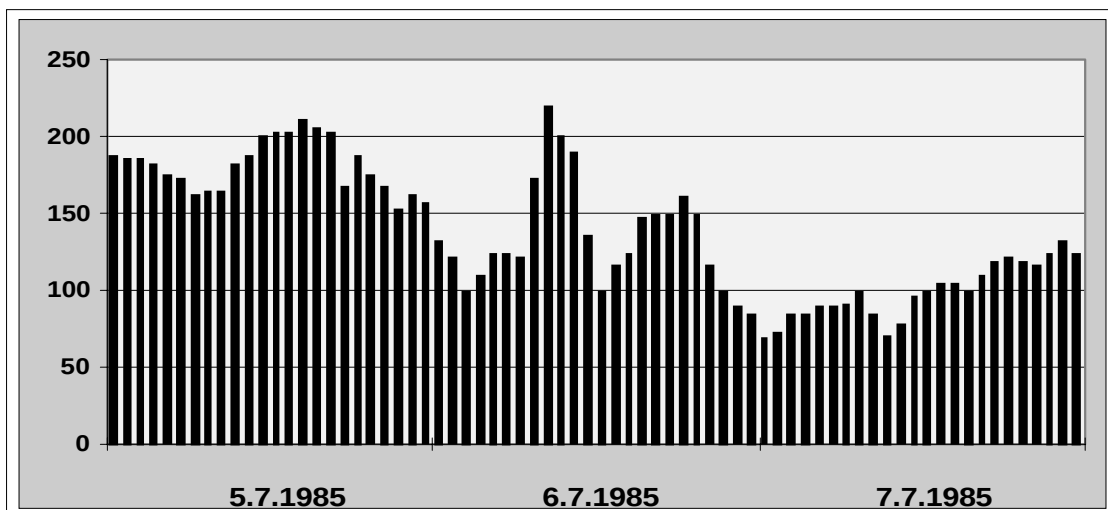
Abb. 45) Noch plausible Werte an der Station WESTEIFEL (RP015)
