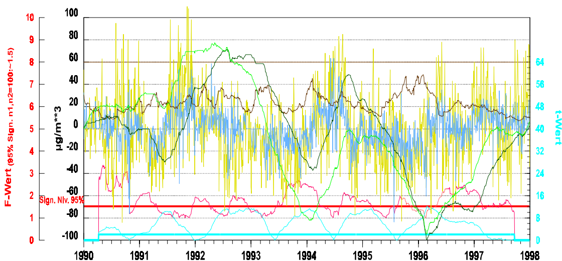
Abb. 91) Original-Ozonreihe der Station AALEN (BW029), Zeitraum 1990 – 1997 Messnetz Baden-Württemberg
