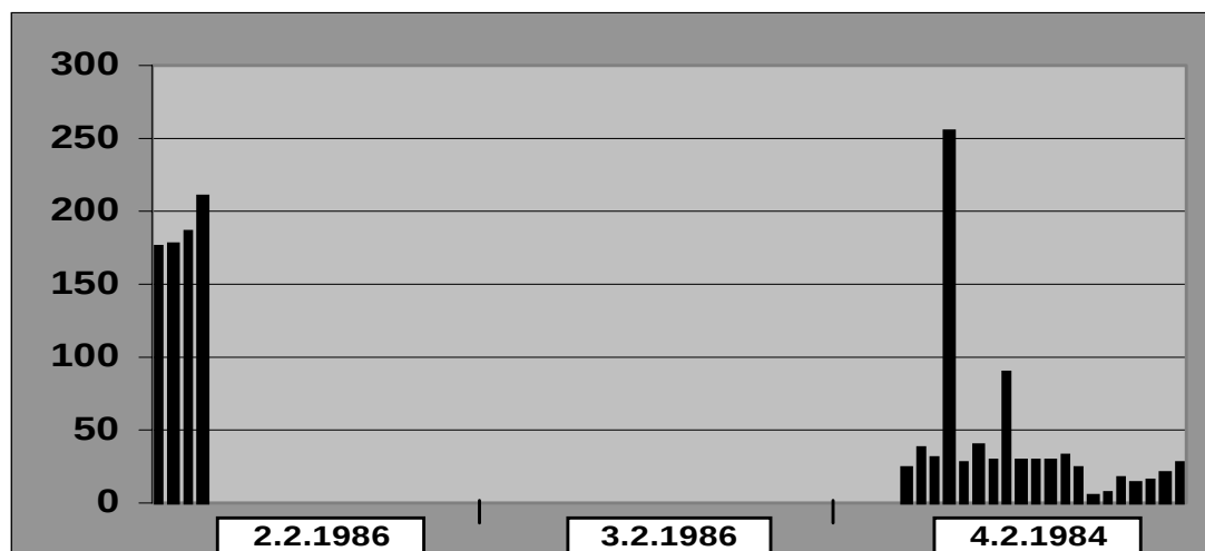
Abb. 49) Ausreißer oder Kalibrierwerte? Nicht plausible Werte an der Station ARZBERG (BY002), 2. und 4.2.1986
