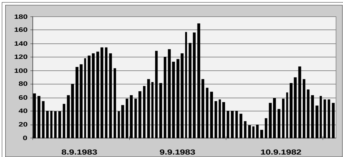
Abb. 30) Nicht plausible Messwerte an der Station WAHNSDORF (SN051), die Werte bleiben jedoch im Kollektiv
