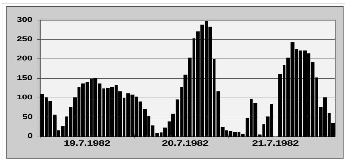
Abb. 21) Fragwürdige, aber plausible Werte an der Station EGGENSTEIN im Juli 1982 (BW004)
