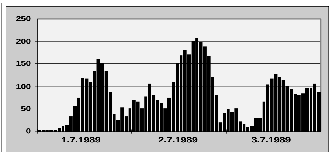
Abb. 64) Station LH-MUNDENHEIM (RP003): Der kritisierte Messwert ist als plausibel einzustufen
