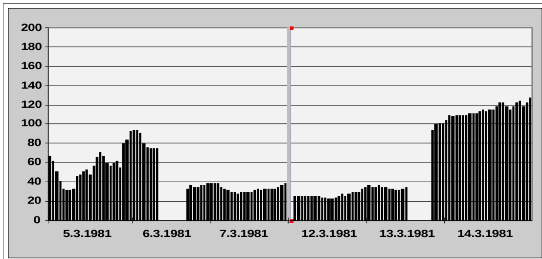
Abb. 10) Systematischer Messfehler im Datenkollektiv der Station SCHAUINSLAND (UB004)
