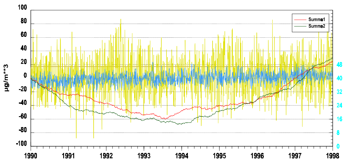
Abb. 77) Verlauf der Summenkurven I und II bei Anwesenheit eines Trends in der Originalreihe
