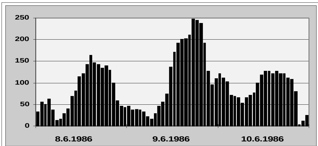
Abb. 54) HÜRTH-EFFEKT an der Station TRIER (RP020). Die Werte werden noch als plausibel angesehen
