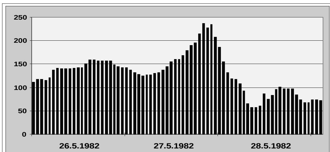
Abb. 25) Fragwürdige, aber nicht unplausible Werte an der Station SCHMÜCKE (UB029) im Mai 1982
