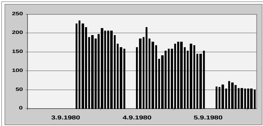
Abb. 06) Systematischer Messfehler, eingebettet in Ausfallperioden an der Station DEUSELBACH (UB002)
