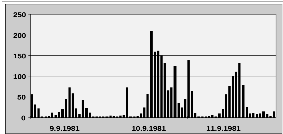
Abb. 16) Ausreißer oder HÜRTH-EFFEKT an der Station BAD CANNSTADT (BW013)
