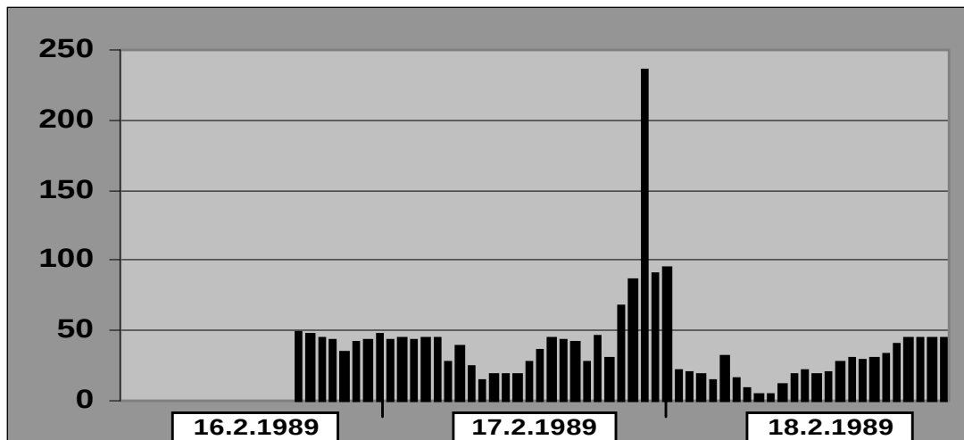
Abb. 61) Nicht plausibler Messwert an der Station NORDENHAM (NI036) im Wintermonat Februar
