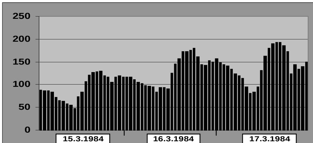
Abb. 41) Fragwürdige, aber als noch plausibel angesehene Messwerte an der Station KREUZECKBAHN (BY081)
