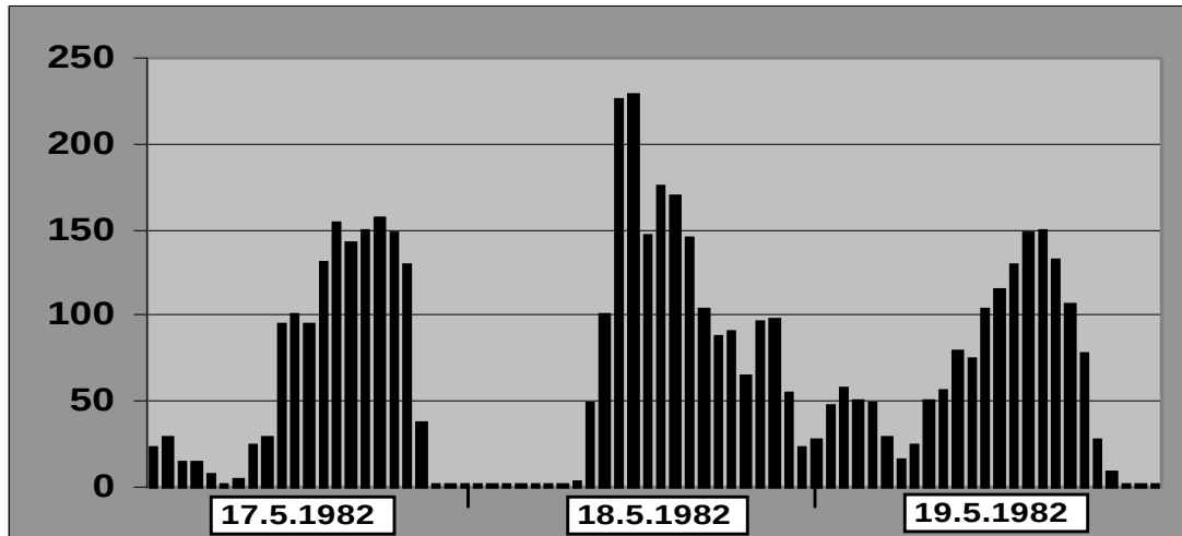
Abb. 19) Ausreißer oder HÜRTH-EFFEKT an der Station EGGENSTEIN im Mai 1982 (BW004)
