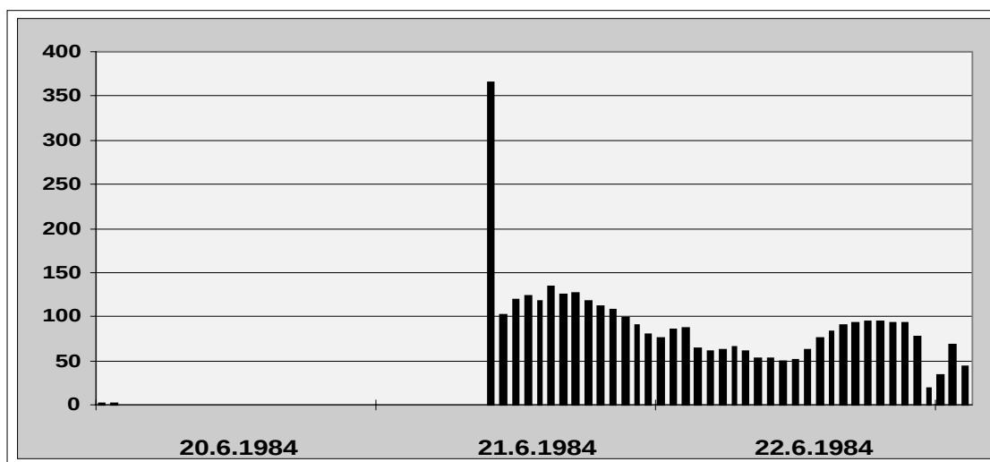
Abb. 37) Ein einzelner nicht plausibler Messwert (Kalibrierwert?) an der Station EGGENSTEIN (BW004)
