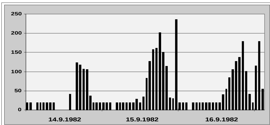
Abb. 24) Nicht plausible Messwerte und hohe “Sockelwerte” an der Station HÜRTH (NW058)
