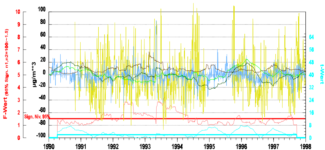
Abb. 87) Original-Ozonreihe der Station LÖRICK (NW071), Zeitraum 1990 – 1997 Messnetz Nordrhein-Westfalen (Raum Düsseldorf)
