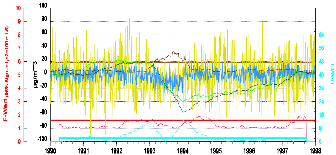
Abb. 83) Sensitivität um 30% reduziert und systematische Abweichung von -10 \mu\text{g}/\text{m}^3 im Jahr 1993
