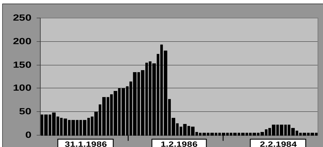
Abb. 51) Nicht plausible Werte an der Station HAUNSTETTEN (BY008) im Wintermonat Februar
