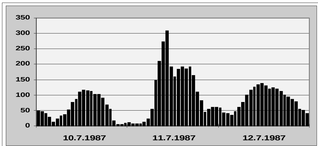
Abb. 58) HÜRTH-EFFEKT an der Station KARLSRUHE-NORDWEST (BW081) Die Werte gelten als plausibel
