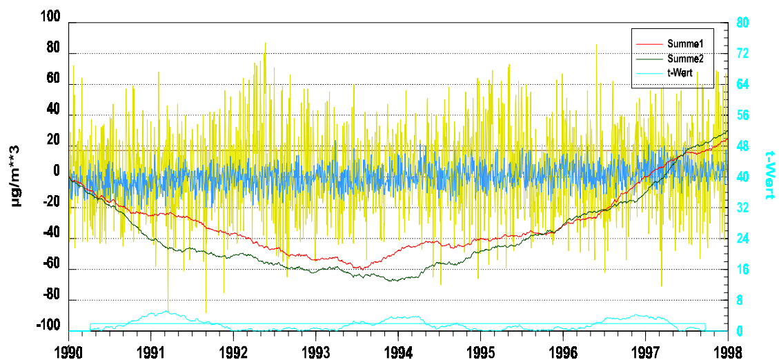
Abb. 79) Testgröße "Gleitender t-Wert (blaue Kurve) bei Anwesenheit eines Trends in der Originalreihe
