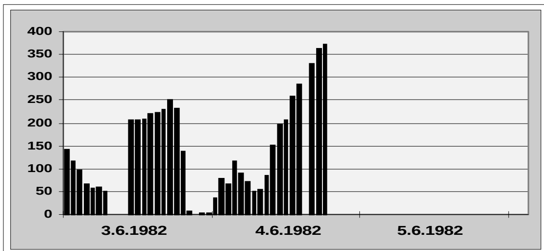
Abb. 20) Fragwürdige Messwerte an der Station EGGENSTEIN im Juni 1982 (BW004)
