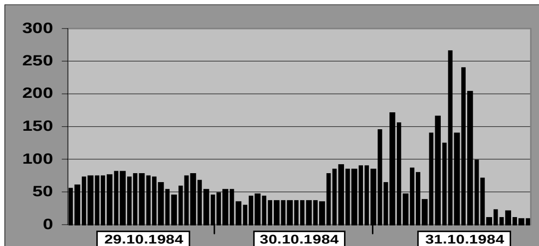
Abb. 42) Nicht plausible Werte (Schätzwerte) an der Station SCHMÜCKE (UB029)
