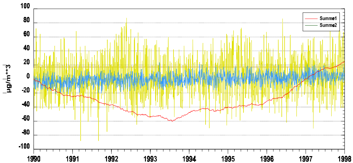
Abb. 76) Verlauf der Summenkurve I bei Anwesenheit eines Trends in der Originalreihe Trend in der Originalreihe = 2\mu\text{g}/\text{m}^3 pro Jahr
