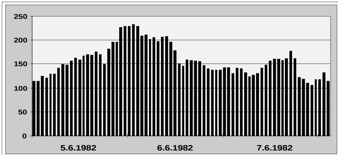
Abb. 26) Fragwürdige, aber nicht unplausible Werte an der Station SCHMÜCKE (UB029) im Juni 1982
