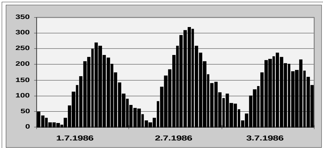
Abb. 55) Keine Auffälligkeiten sind bei den als fragwürdig eingestuften Werten der Station GEESTHACHT (SH003) zu erkennen
