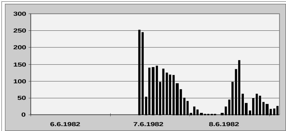
Abb. 22) Ausreißer oder Kalibrierwerte an der Station MANNHEIM-MITTE (BW006)
