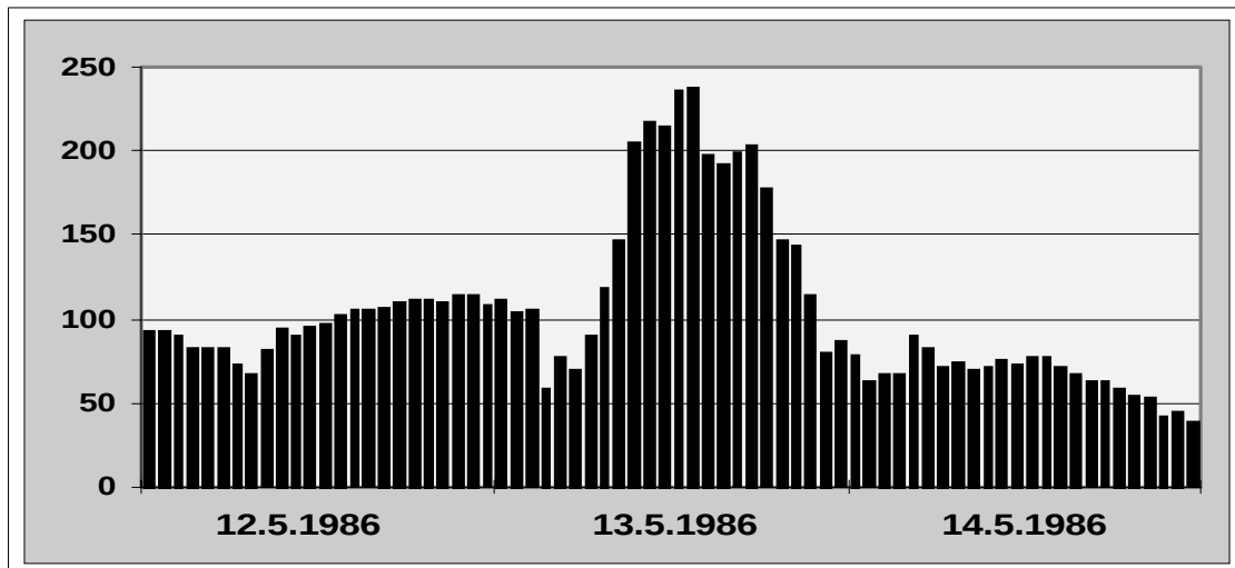
Abb. 56) Mehrere unplausible Werte an der Station SCHMÜCKE (UB029) im Mai 1986
