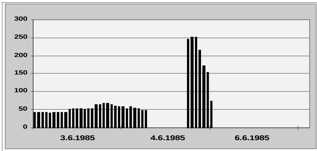
Abb. 07) Nicht plausible Messwerte, eingebettet in Ausfallperioden an der Station WESTEIFEL (RP015)
