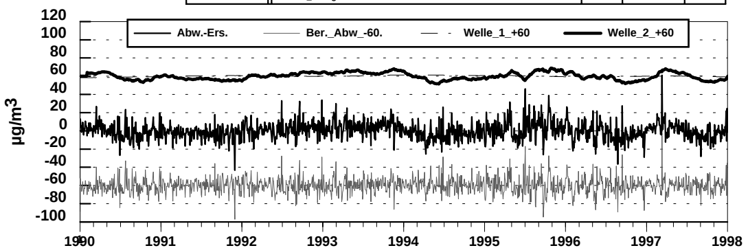
Abb. 98: Validierung der Ozon- Meßreihe HE027 - Frankenberg vor- und nach der Bereinigung von Strukturbrüchen, April bis September, 5-stündiges Mittel (13 bis 17 Uhr)
