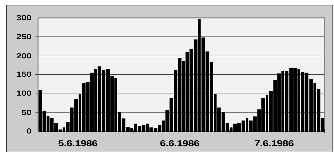
Abb. 53) HÜRTH-EFFEKT an der Station TRIER (RP020). Der Wert wird noch als plausibel angesehen
