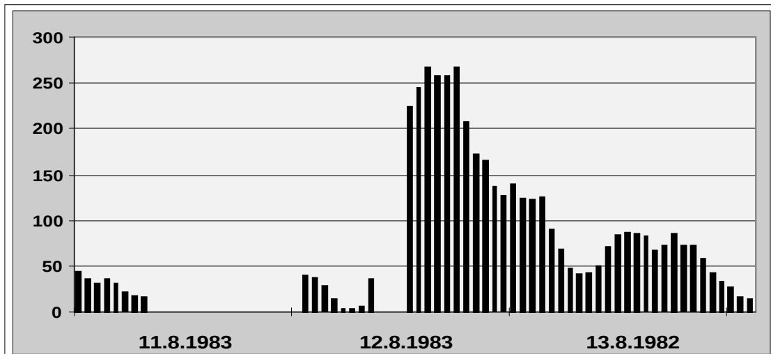
Abb. 27) Fragwürdige, aber nicht unplausible Werte an der Station MANNHEIM NORD (BW005)
