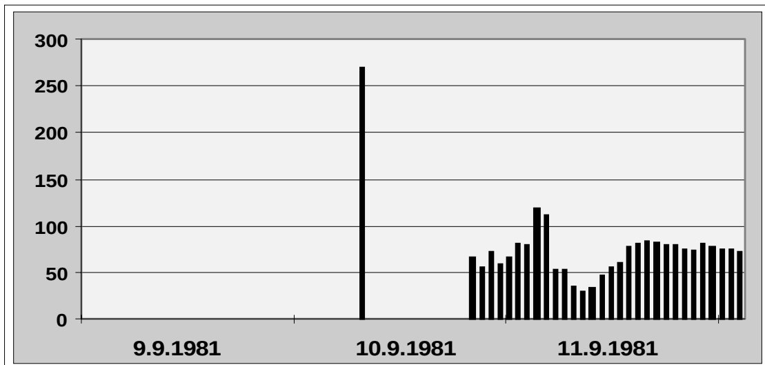
Abb. 17) Nicht plausibler Einzelwert in einer Ausfallperiode an der Station HEILBRONN (BW015)
