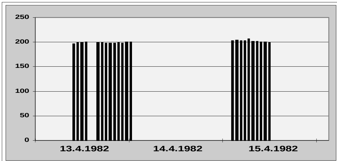
Abb. 08) Kalibrierwerte (?) im Datenkollektiv der Station LIS-ESSEN (NW028)
