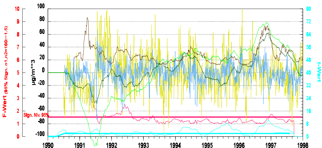
Abb. 89) Original-Ozonreihe der Station VILLINGEN (BW039), Zeitraum 1990 – 1997 Messnetz Baden-Württemberg
