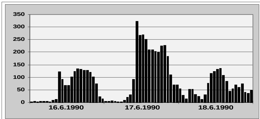
Abb. 68) Ein typisches Beispiel für den HÜRTH-EFFEKT an der Messstation HÜRTH (NW058) im Juni 1990
