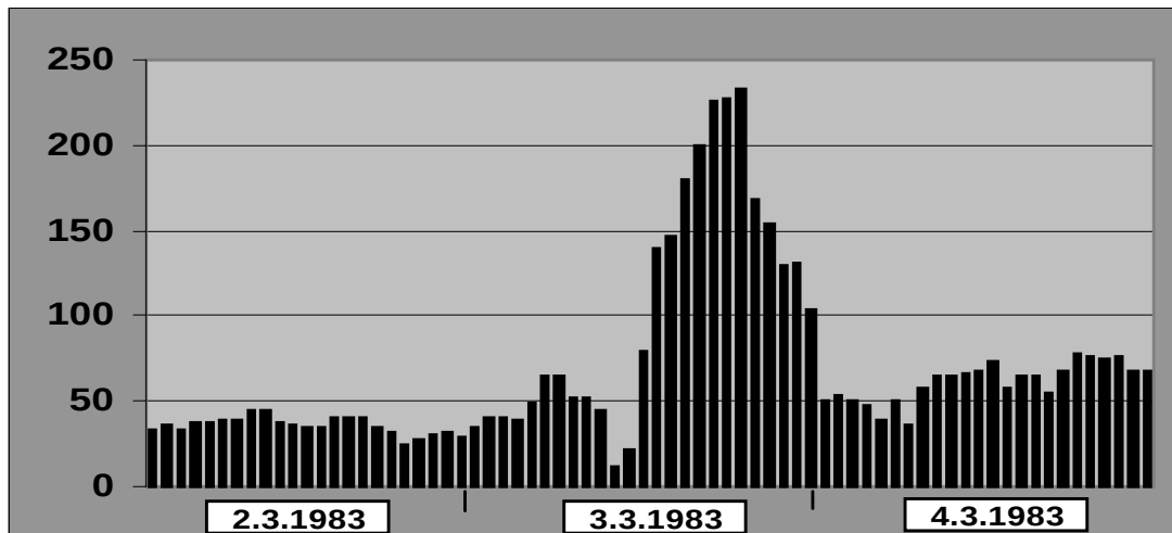
Abb. 31) Nicht plausible Werte (Schätzwerte) an der Station SCHMÜCKE (UB029) im März 1983
