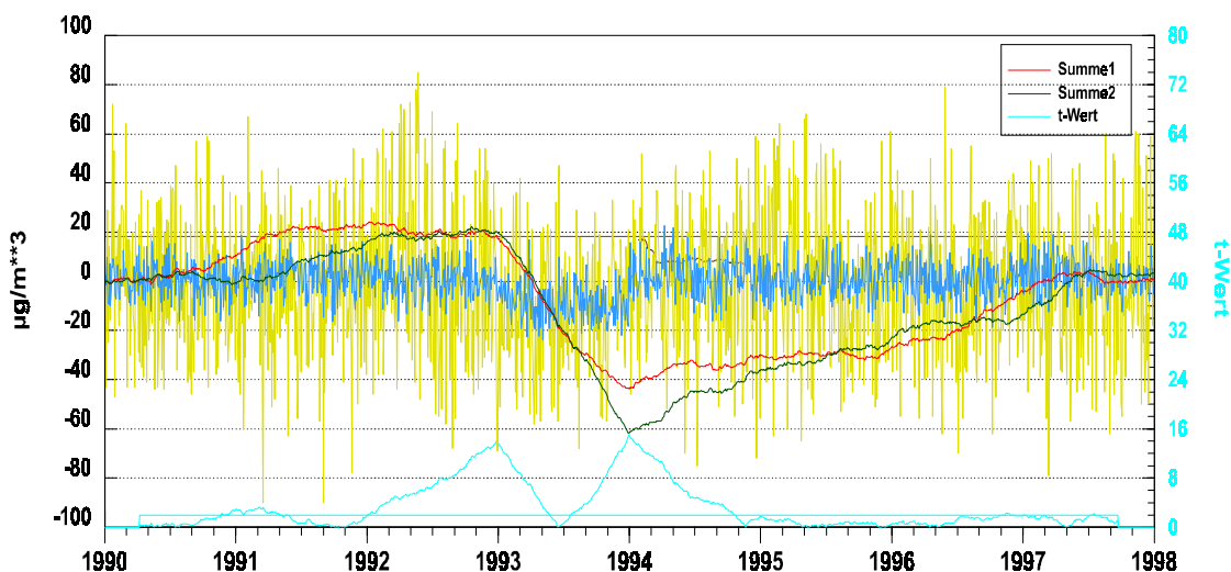
Abb. 80) Testgröße “Gleitender t-Wert” (blaue Kurve) bei Anwesenheit einer stufenförmigen Intervention in der Originalreihe
