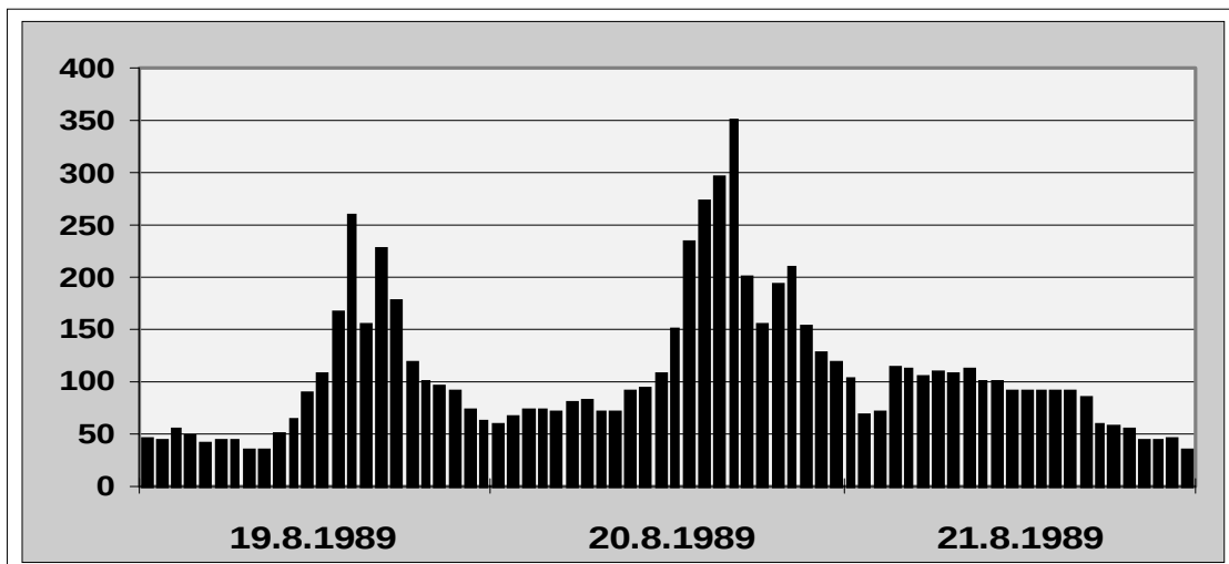
Abb. 66) Nicht plausible Messwerte an der Station HOHENWESTEDT (UB006) im August 1989
