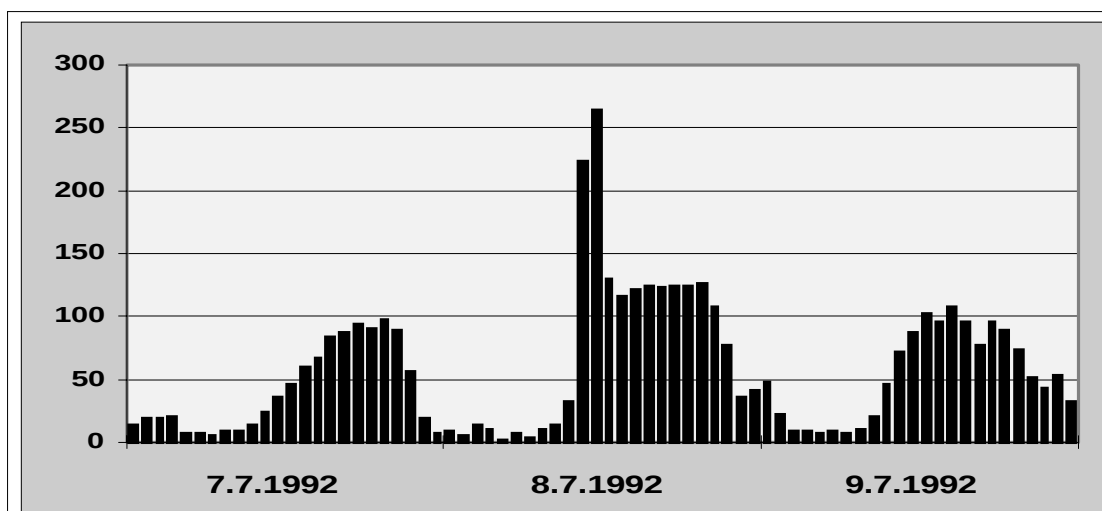
Abb. 72) Der HÜRTH-EFFEKT im Juli 1992 an der Messstation HÜRTH bei Köln (NW058)
