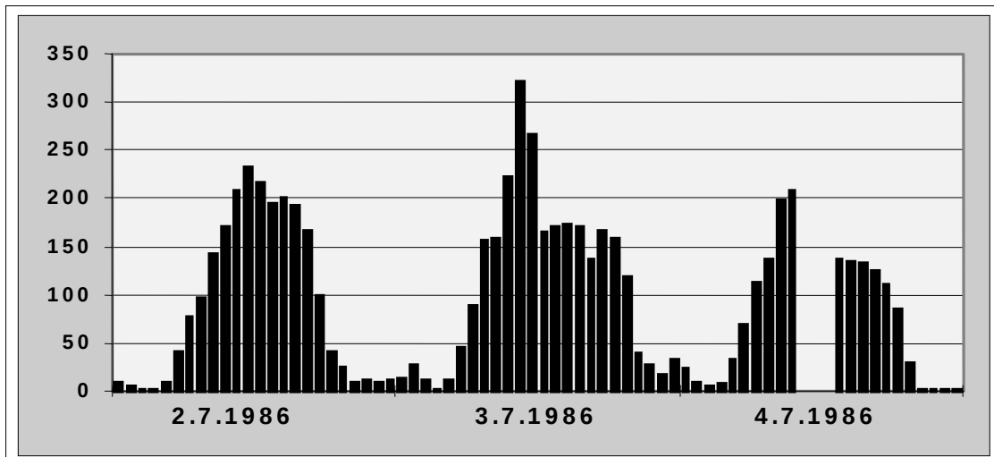
Abb. 46) Ausreißer oder HÜRTH-EFFEKT? Fragwürdige, aber noch plausible Werte in EGGENSTEIN (BW004)
