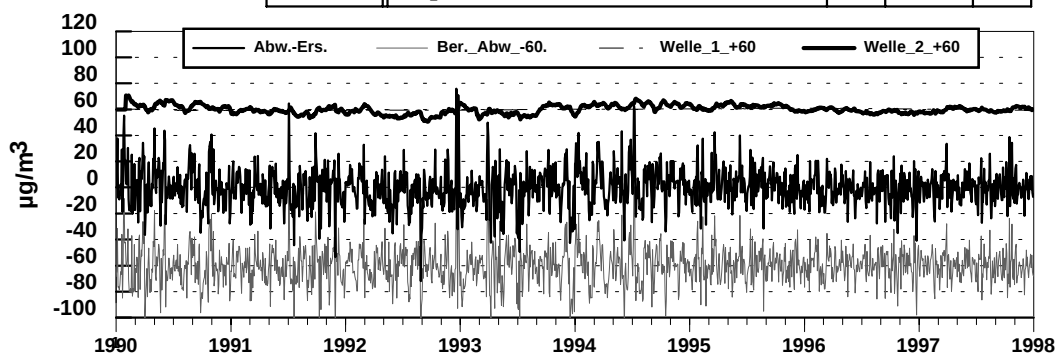
Abb.100: Validierung der Ozon- Meßreihe SN051 - Wahnsdorf vor- und nach der Bereinigung von Strukturbrüchen, April bis September, 5-stündiges Mittel (13 bis 17 Uhr)
