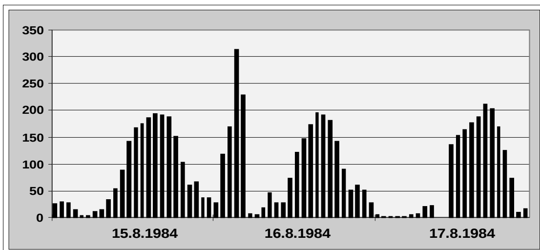
Abb. 39) Nicht plausible Ausreißer an der Station MANNHEIM-NORD (BW005) im Monat August 1984
