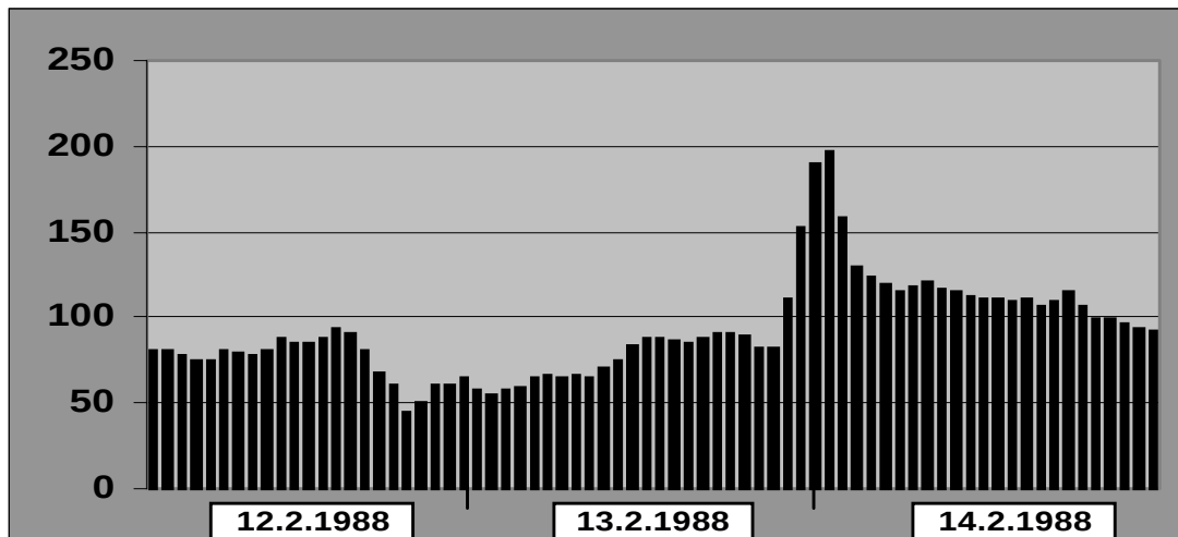
Abb. 60) Nicht plausible Messwerte an der Station ZUGSPITZE (BY083) im Wintermonat Februar
