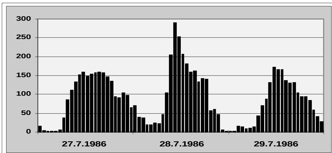
Abb. 47) Ausreißer oder HÜRTH-EFFEKT? Fragwürdige, aber noch plausible Werte in KEHL-HAFEN (BW022)
