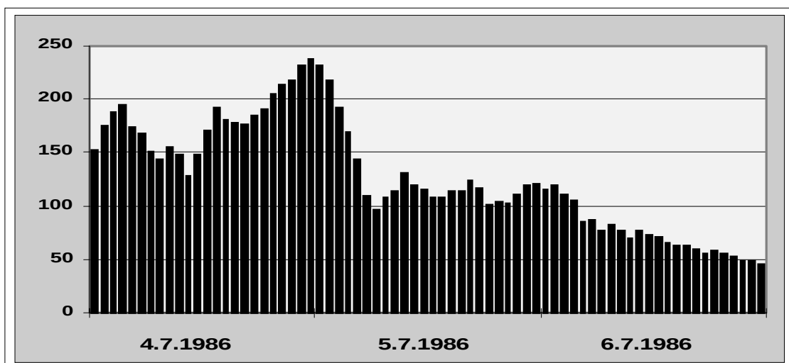
Abb. 57) Weitere unplausible Werte an der Station SCHMÜCKE (UB029)
