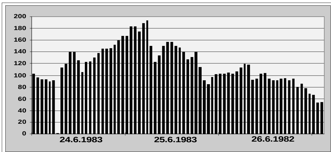
Abb. 32) Fragwürdige Messwerte an der Station SCHMÜCKE (UB029) im Monat Juni 1983
