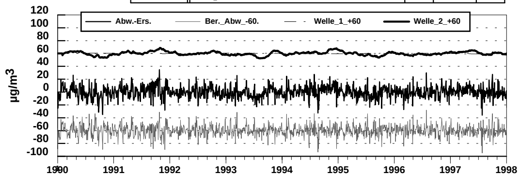
Abb. 97: Validierung der Ozon- Meßreihe BY002 - Arzberg vor- und nach der Bereinigung von Strukturbrüchen, April bis September, 5-stündiges Mittel (13 bis 17 Uhr)
