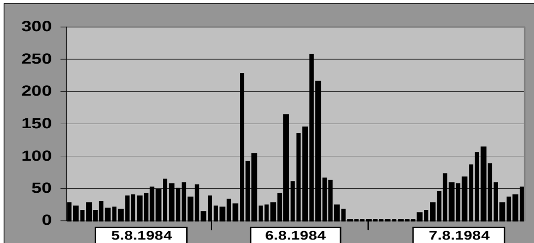
Abb. 38) Nicht plausible Messwerte im August 1984 an der Station MANNHEIM NORD (BW005)
