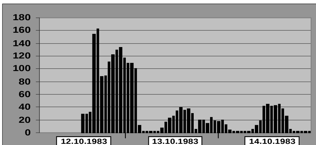
Abb. 35) Nicht plausible Messwerte an der Station KASSEL-NORD (HE014)
