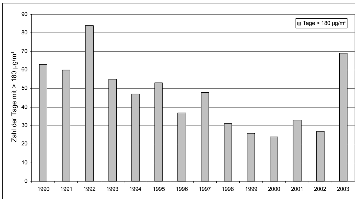
Abb. 3: Zahl der Tage mit Überschreitungen von 180 µg/m³
