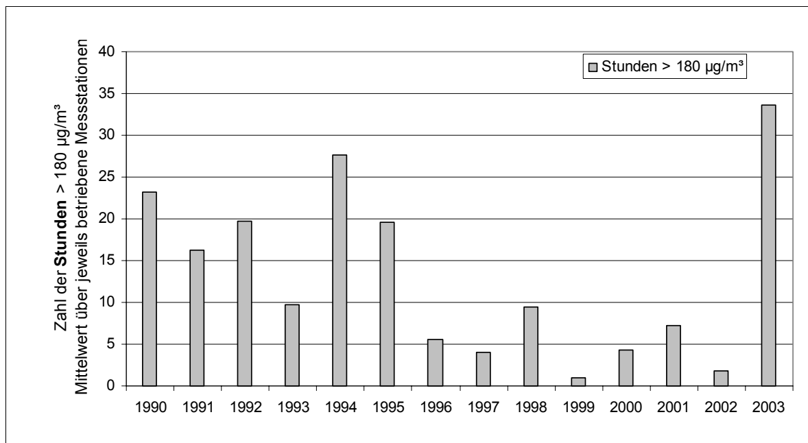
Abb. 2: Zahl der Stunden mit Überschreitungen von 180 µg/m³, im Mittel über die jeweils betriebenen Messstationen
