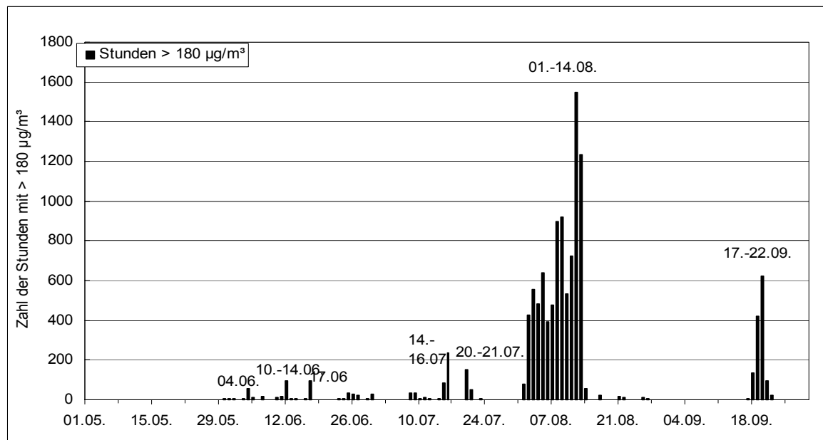
Abb. 1: Zeitliche Verteilung der Häufigkeit der Schwellenwertüberschreitungen (Stunden) von 180 \mu\text{g}/\text{m}^3
