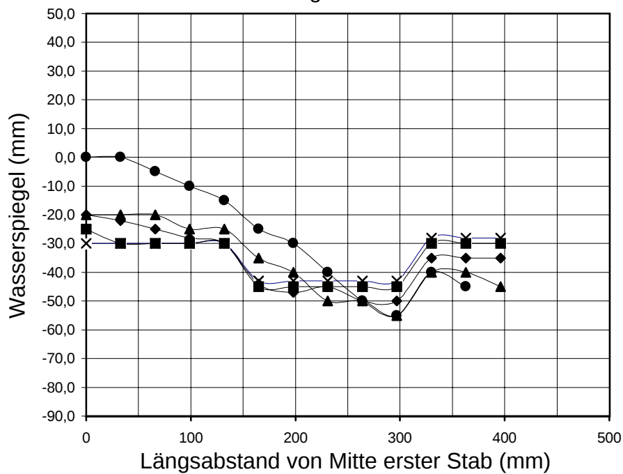
Wasserspiegel Längsprofile Messung am Matrixblock
