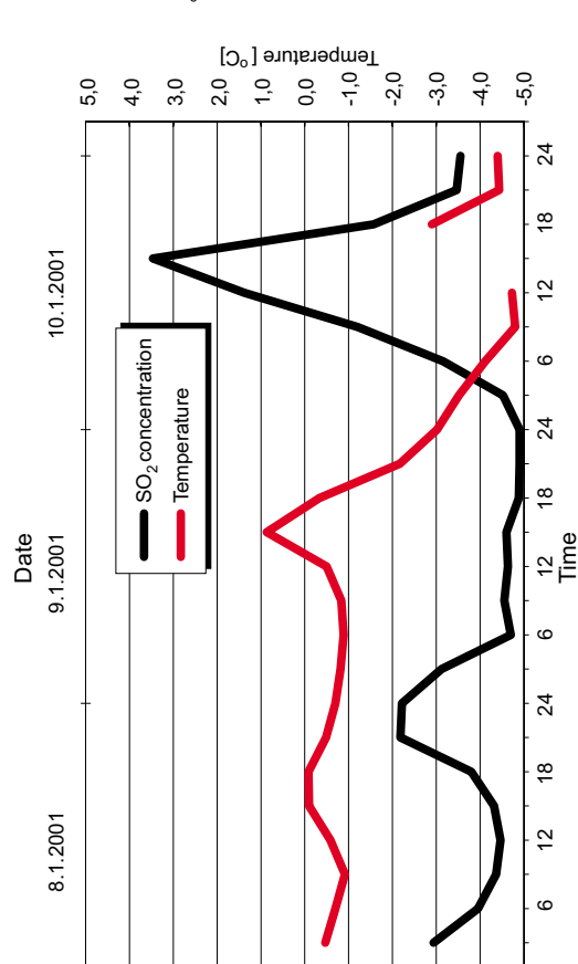
Figure 30. Maximum concentration in wintertime: Jeleniów – lowland station Obrázek 30. Maximální zimní koncentrace: stanice Jeleniów v nížko položené oblasti Abbildung 30. Winterepisode für die tiefer gelegene Station Jeleniów Rysunek 30. Maksymalne stężenie w okresie zimowym: Jeleniów – stacja nizinna
