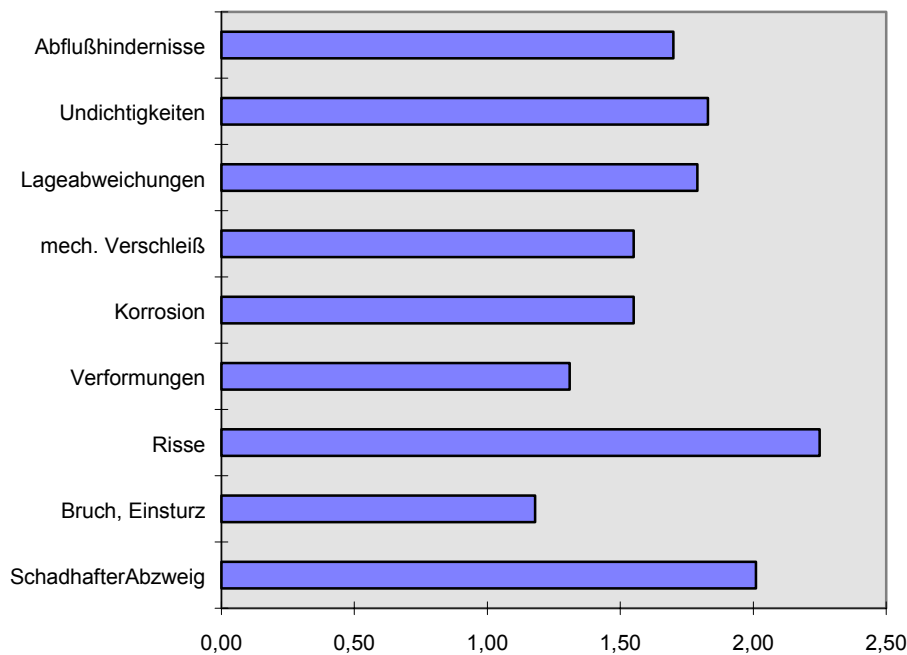
Abbildung 7.1: Häufigkeitsverteilung der Kanalschadensbilder [DY-98]
