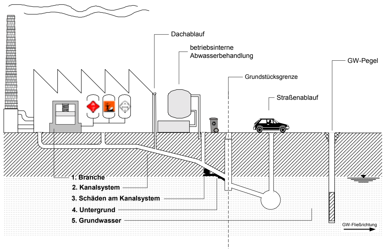
Abbildung 3.1: Randbedingungen bei undichten industriellen und gewerblichen Grundstücksentwässerungsleitungen
