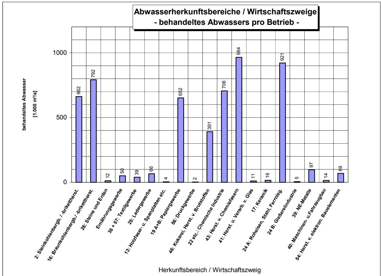
Abbildung 4.2: Abwasserherkunftsbereiche / Wirtschaftszweige - durchschnittliche behandelte Abwassermengen pro Betriebsstandort
