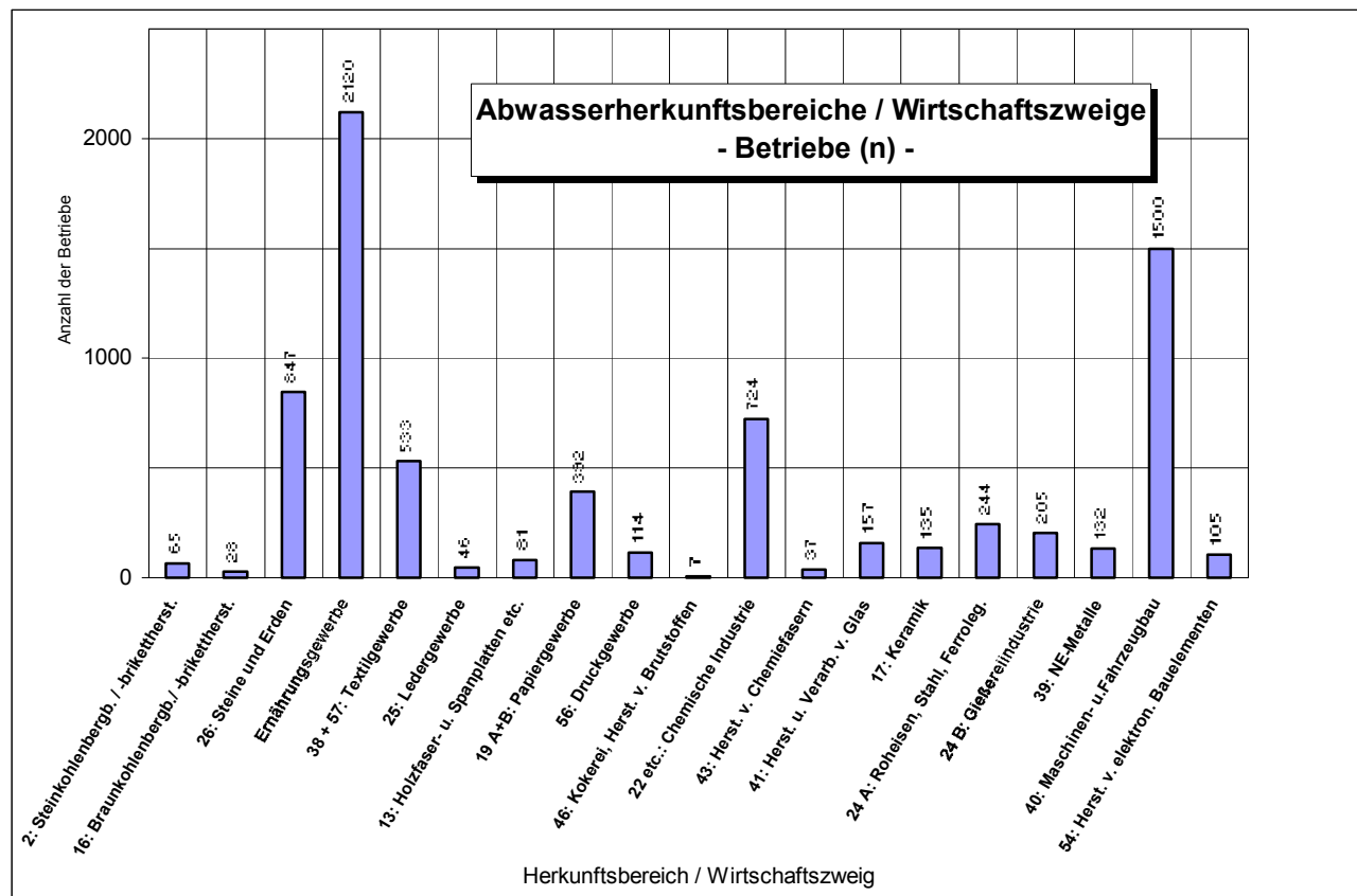
Abbildung 4.1: Abwasserherkunftsbereiche / Wirtschaftszweige - Anzahl der Betriebe mit einem Wasseraufkommen von > 10.000 m 3 /a
