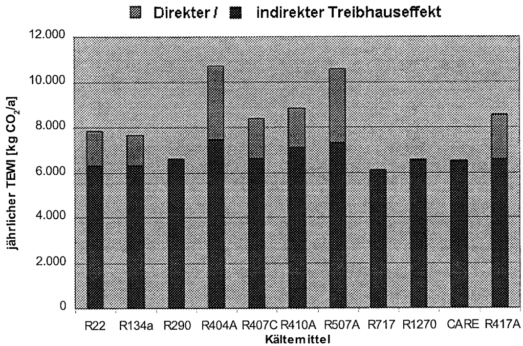
Bild 7.8: Jährlicher TEWI der Modell-Gebäudeklimaanlage
