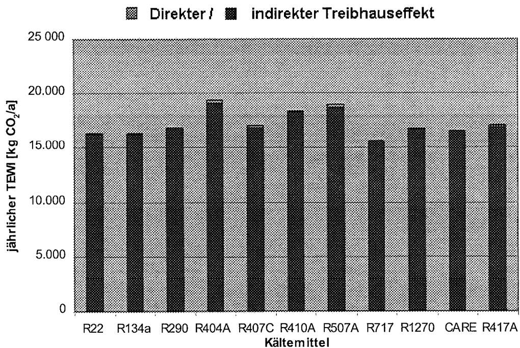
Bild 7.11: Jährlicher TEWI der Modell-Luft/Wasser-Wärmepumpe
