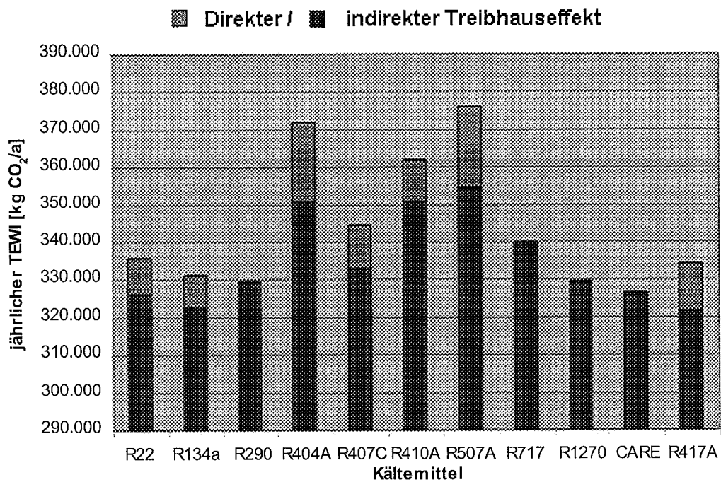
Bild 7.9: Jährlicher TEWI des Modell-Solesatzes
