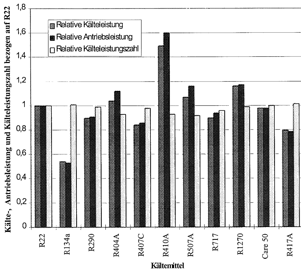
Bild 2.2: Relative Kälte- und Antriebsleistung sowie Kälteleistungszahl (bezogen auf R22) verschiedener Ersatzstoffe für das Beispiel Supermarktkälte / Tiefkühlung
