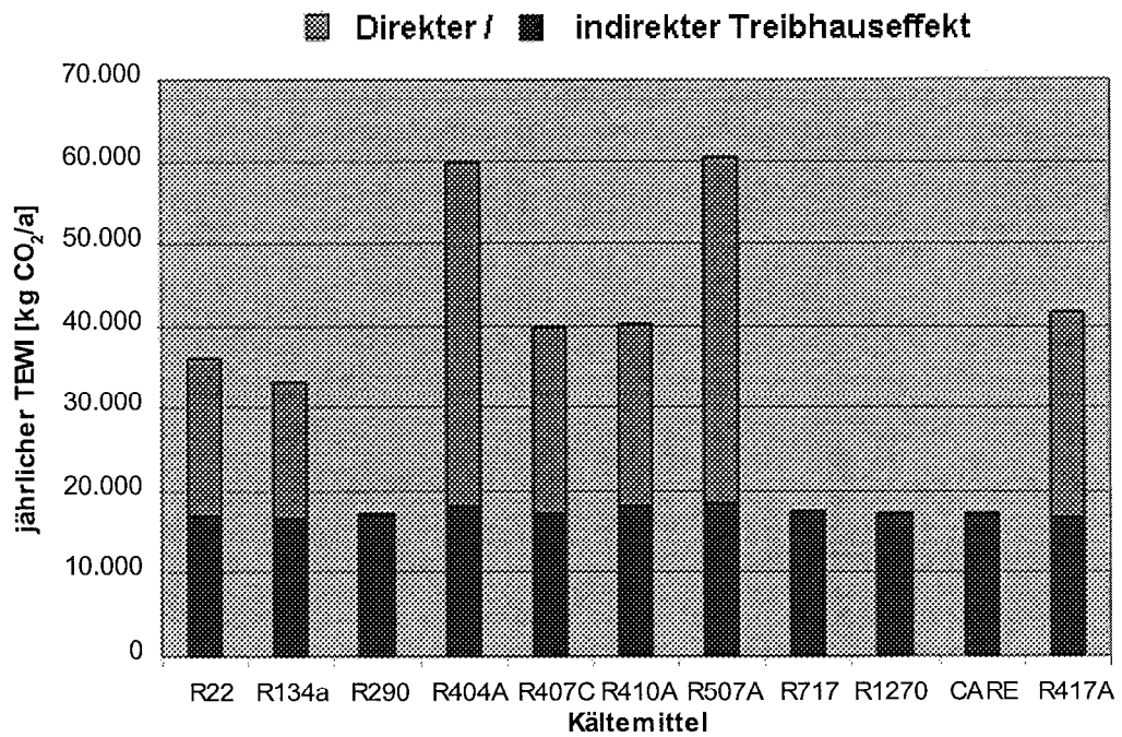
Bild 7.7: Jährlicher TEWI der Modell-Supermarktkälteanlage (Tiefkühlung)
