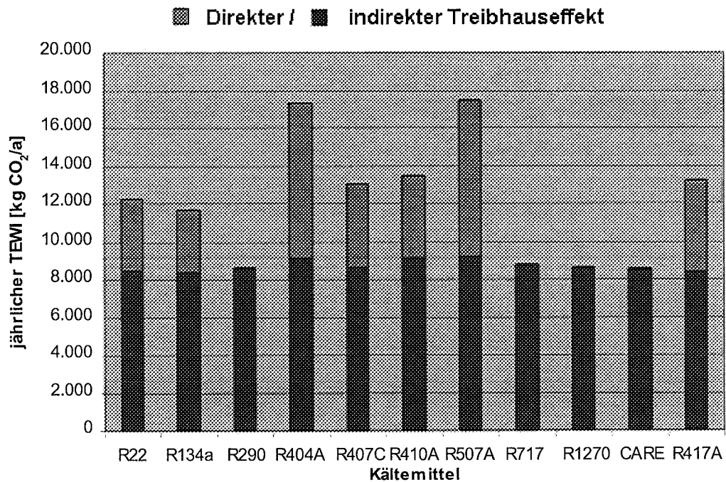
Bild 7.10: Jährlicher TEWI der Modell-Transportkälteanlage (Tiefkühlung)
