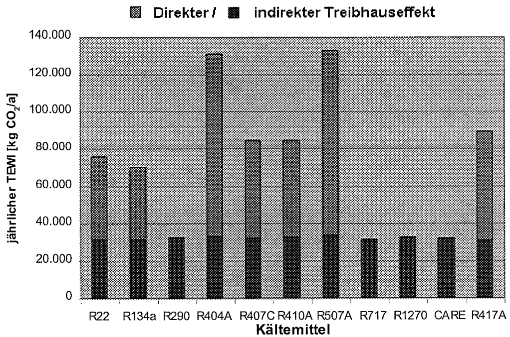
Bild 7.6: Jährlicher TEWI der Modell-Supermarktkälteanlage (Normalkühlung)
