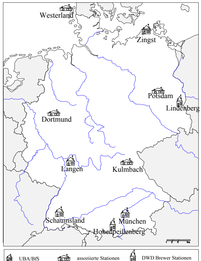
Abbildung: UV-Messstationen in Deutschland, die im Jahre 2000 die UV-Strahlung mittels Spektralradiometern gemessen haben
