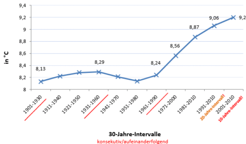
Abbildung 2: Zunahme der Mittleren Lufttemperatur in Deutschland
