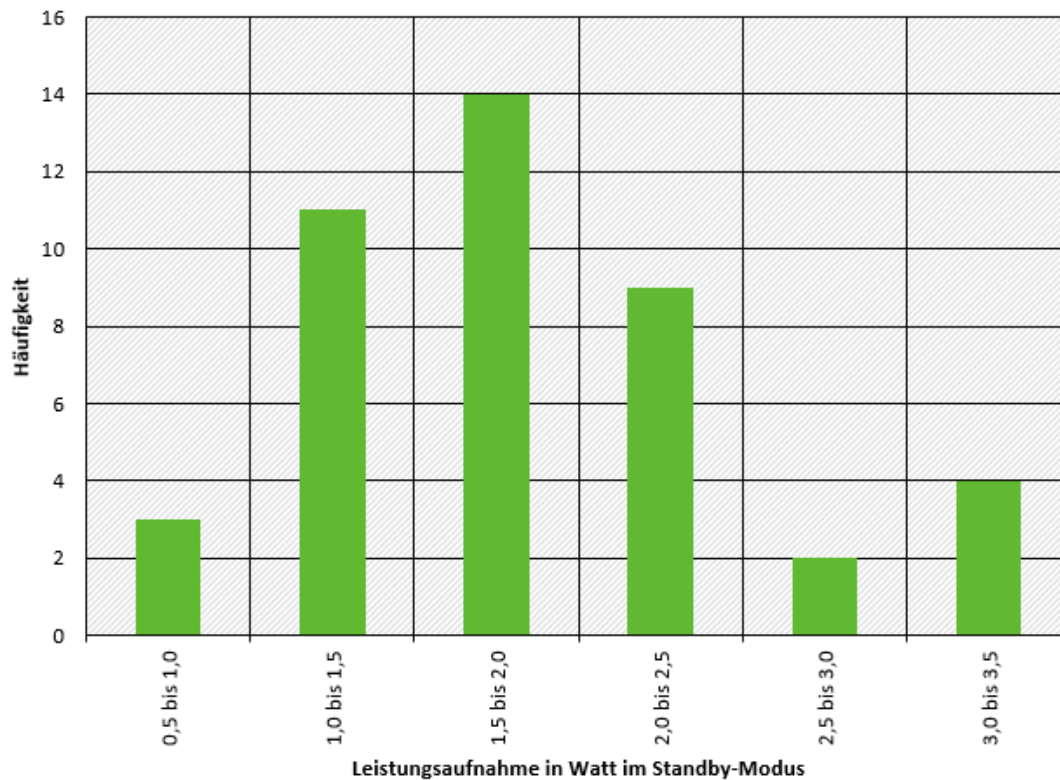
Abbildung 10: Leistungsaufnahme der mit dem Energy Star gekennzeichneten 43 schnurgebundenen Geräten im Idle Mode in Watt
