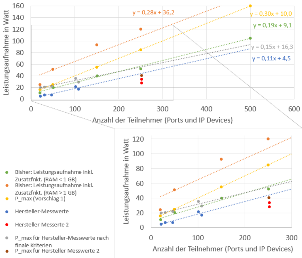
Abbildung 12: Herleitung des Grenzwerts für Telefonanlagen auf Basis bisheriger Grenzwerte
