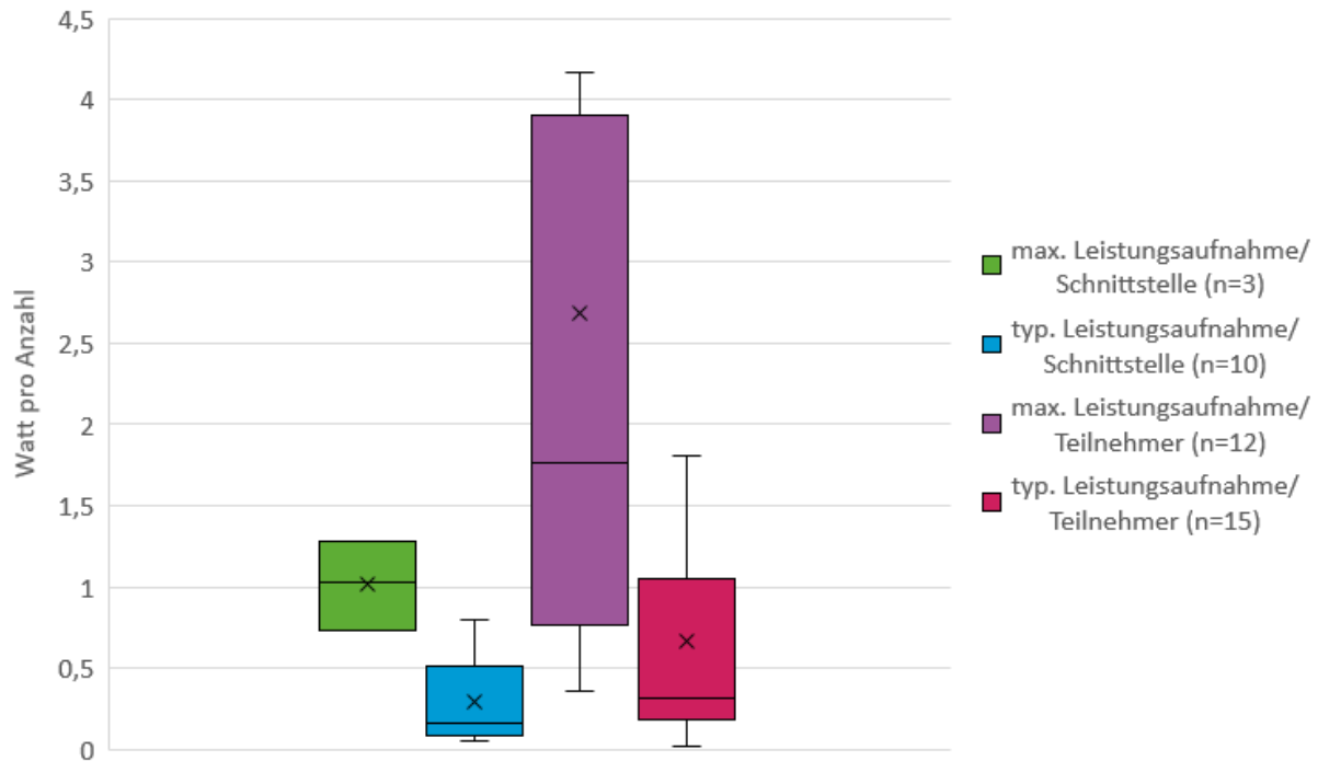
Abbildung 11: Statistische Auswertung von technischen Datenblättern von Telefonanlagen hinsichtlich Leistungsaufnahme pro Benutzer bzw. pro Gerät
