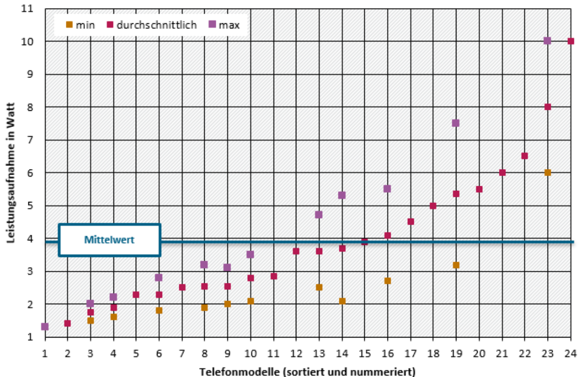
Abbildung 9: Exemplarische Leistungsaufnahme der VoIP-Telefone (Watt)
