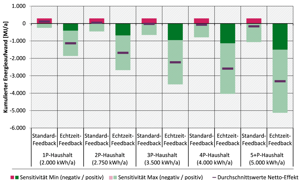
Abbildung 7: Gesamteffekte für Smart Meter bei unterschiedlichen jährlichen Stromverbräuchen
