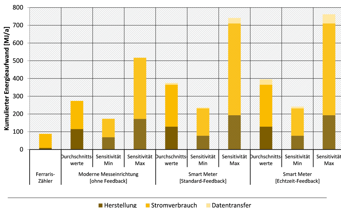
Abbildung 5: Direkte Effekte beim Einbau eines Smart Meters aufgeteilt nach Kategorien
