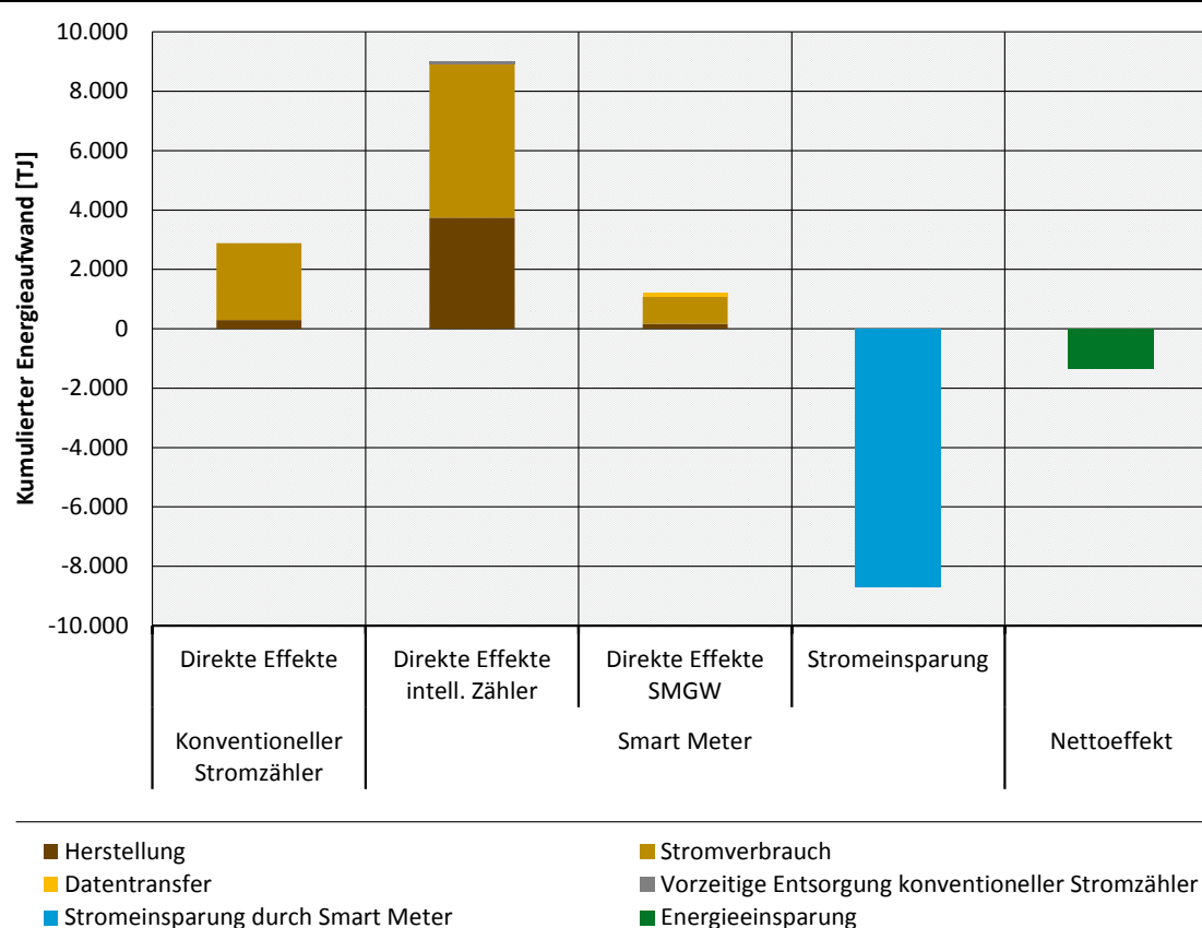
Abbildung 8: Kumulierter Energieaufwand für den Smart Meter Rollout im Base Case hochgerechnet auf das Jahr 2022
