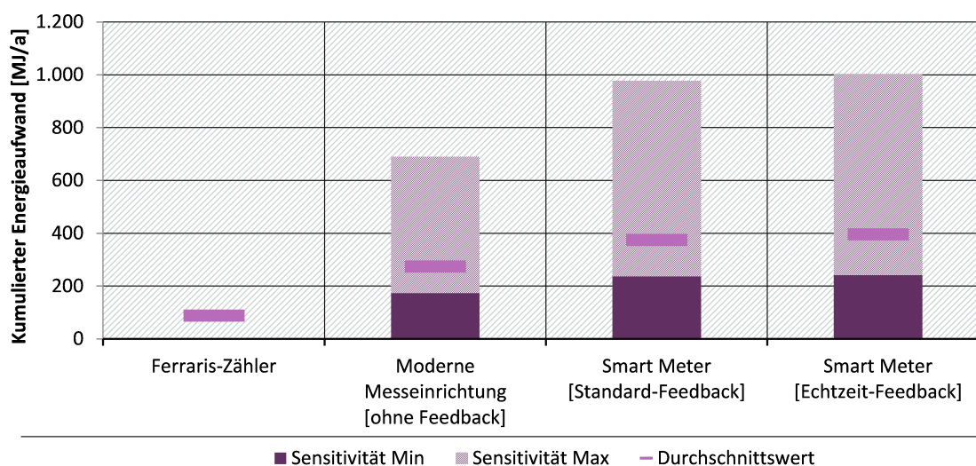
Abbildung 6: Bandbreiten der direkten Effekte beim Einbau eines Smart Meters
