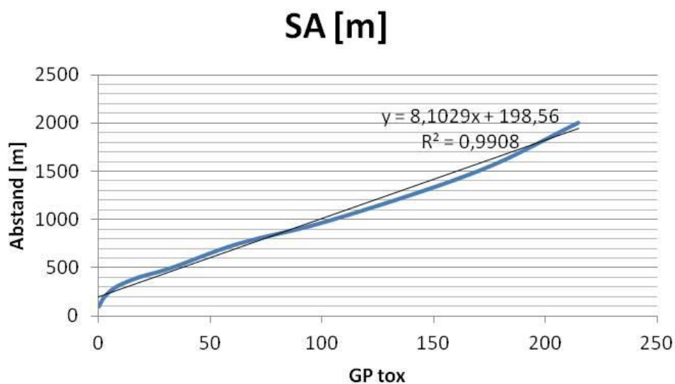
Abbildung 2: Zusammenhang zwischen dem Gefahrenpotential GP_{Tox} und dem angemessenen Sicherheitsabstand nach "Handlungsempfehlung 7 ...". Ausgleichsgrade: A = 8,1 \times GP_{Tox} + 198,56
