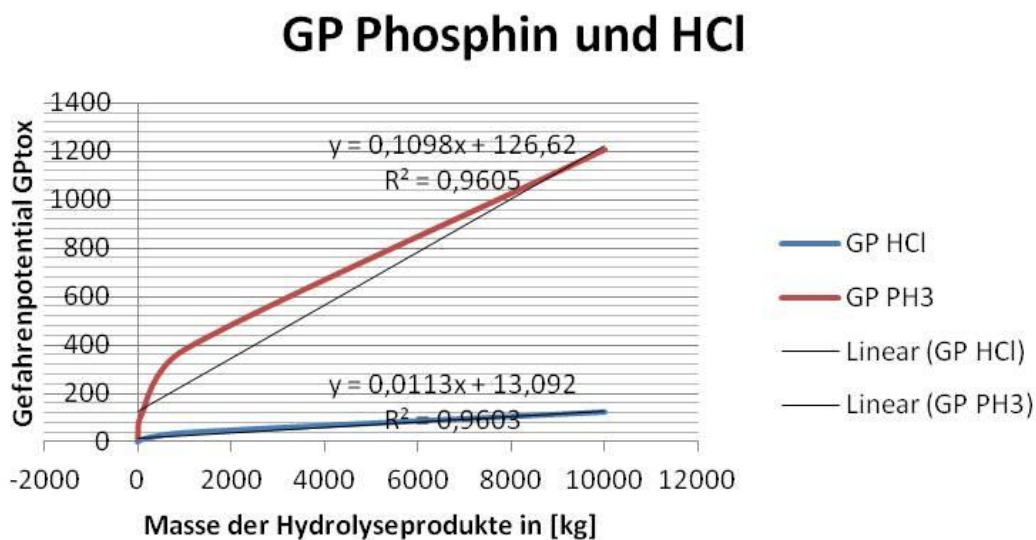
Abbildung 3: Entwicklung des GP für Phosphin und Chlorwasserstoff
