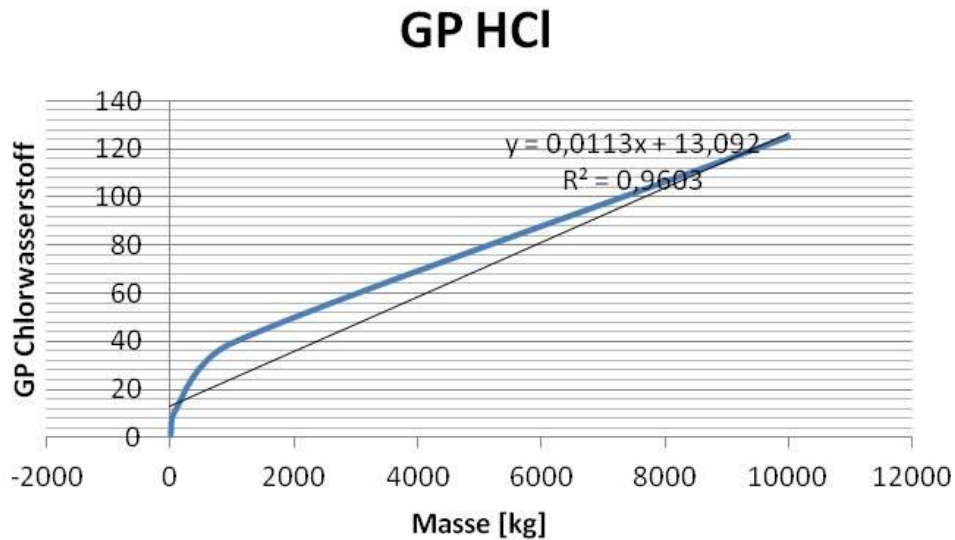
Abbildung 1: Entwicklung des GP_{HCl} in Abhängigkeit von der Masse. Ausgleichsgrade: GP_{HCl} = 0,01113 \times m + 13,1
