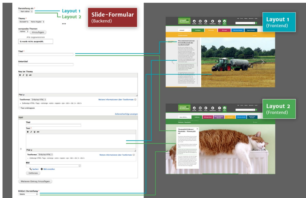
Abbildung 3: Zusammenhang von Backend und Frontend
