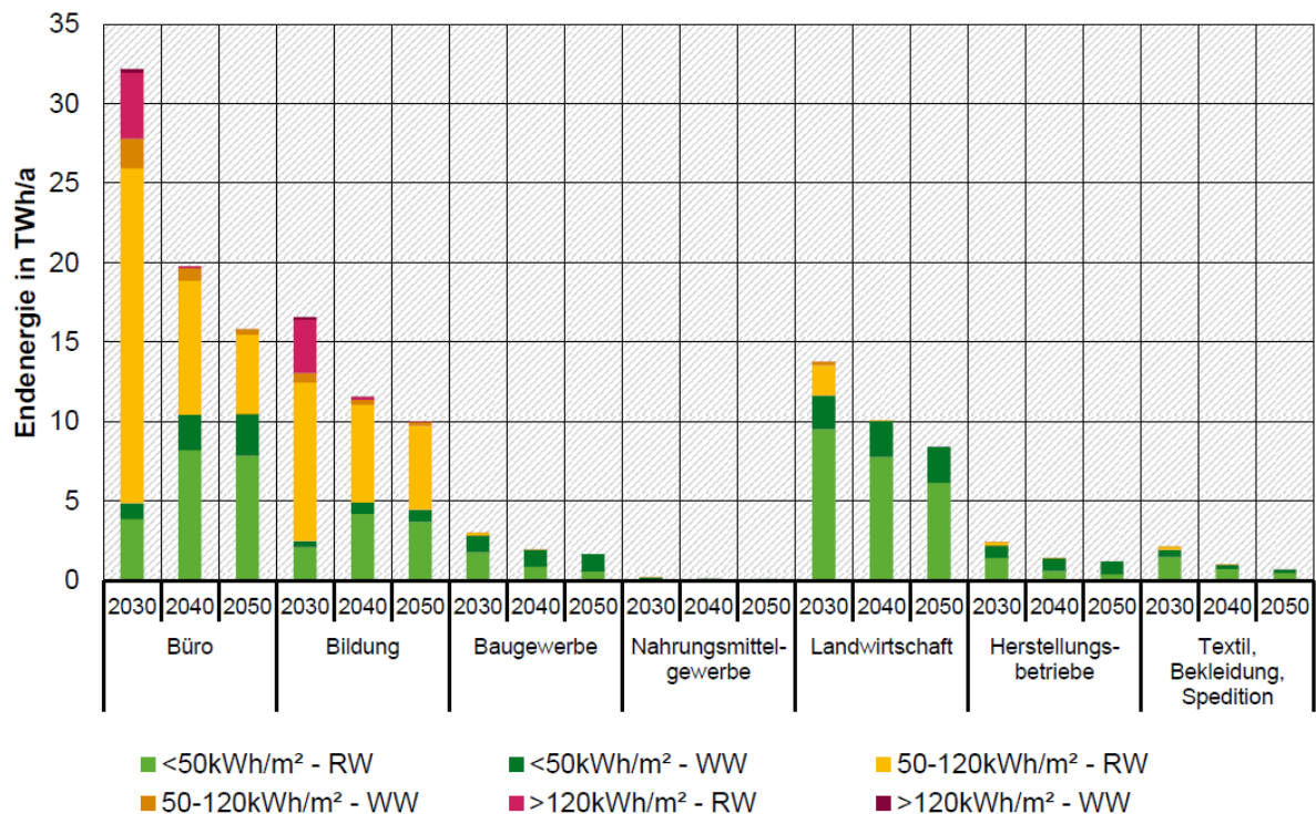
Abbildung 3: Unterteilung der Nichtwohngebäude 1 in Effizienzklassen in GreenLate – Endenergie
