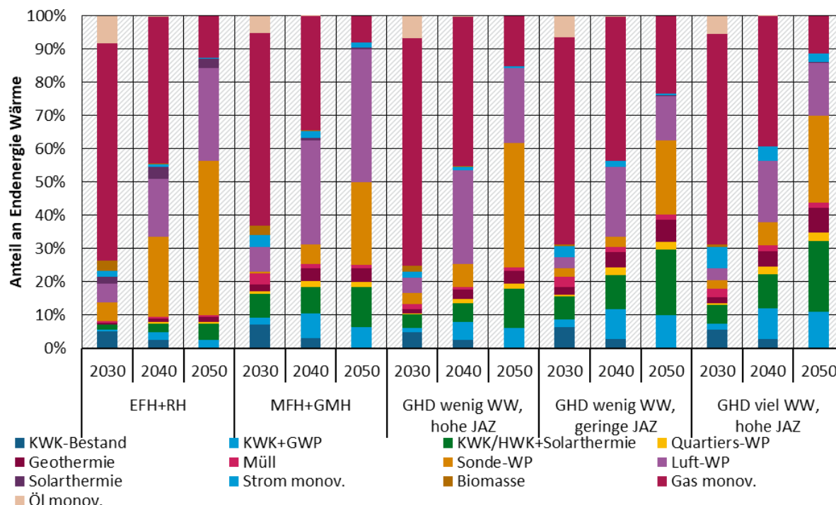
Abbildung 14: Deckung der Wärmenachfrage in GreenLate
