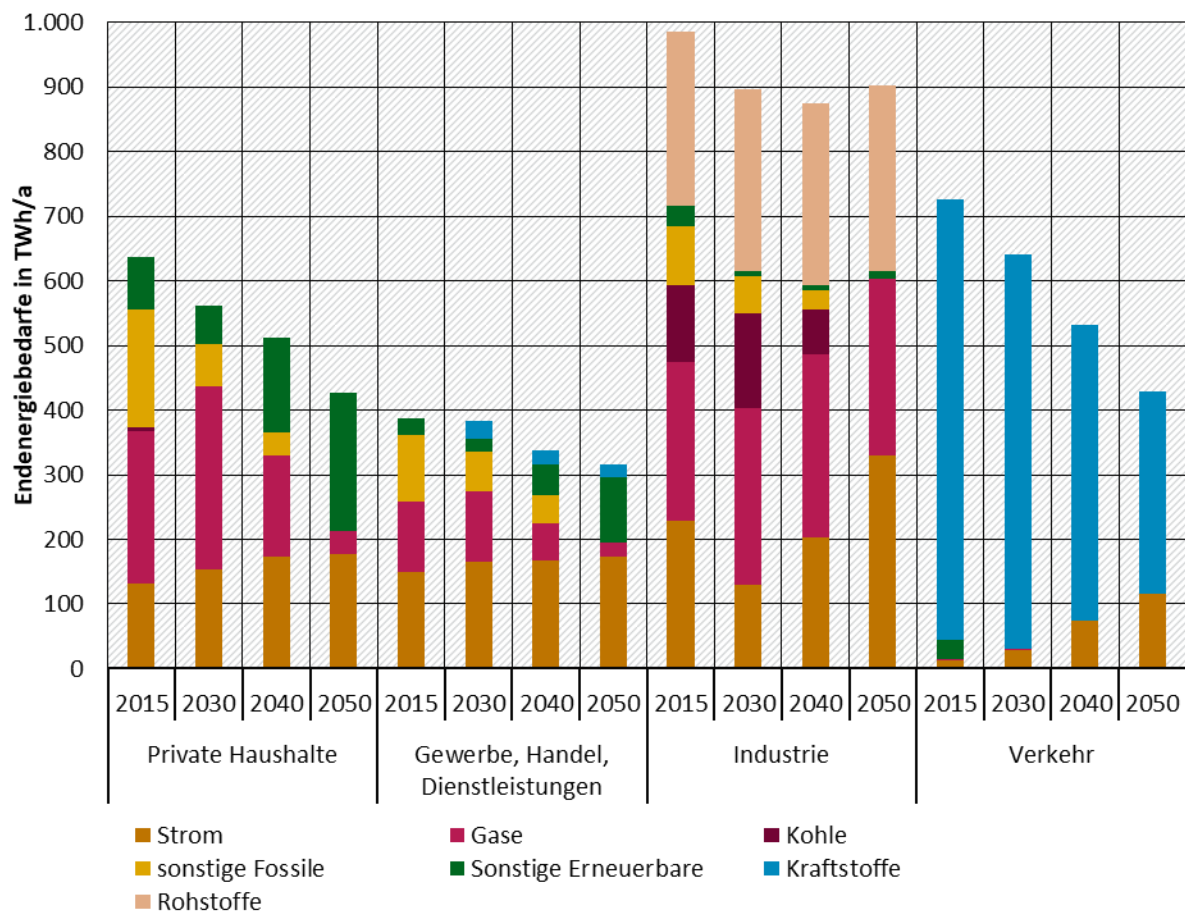
Abbildung Z-1: Entwicklung der Endenergiebedarfe in GreenLate
