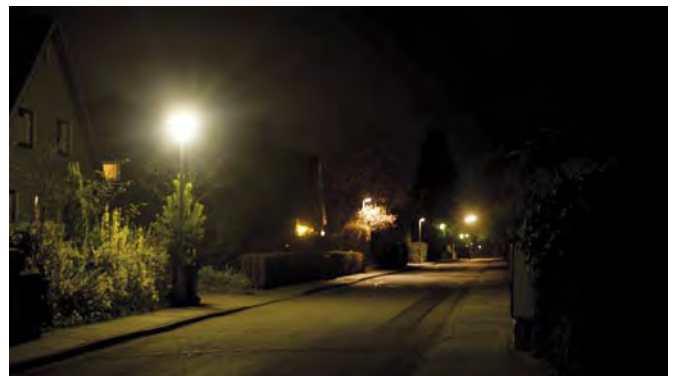
Wohnstraße in Norderstedt: 80 Prozent Energieeinsparung durch den Ersatz alter 80 W Pilzleuchten (im Vordergrund) durch moderne 14 W LED-Leuchten
