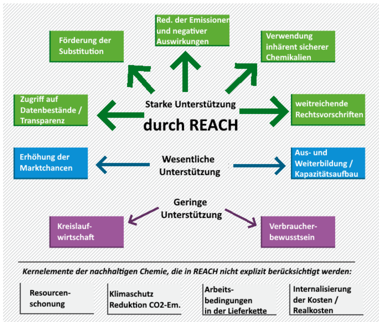
Abb. 1: Kernelemente der nachhaltigen Chemie (grüne Kästen), die in REACH ausdrücklich angesprochen werden, und Kernelemente, die nicht ausdrücklich angesprochen werden (Kästen mit grauer Farbfüllung).
