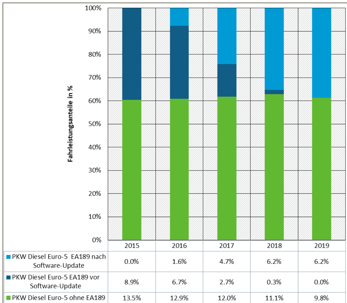
Abbildung 12: Flottenzusammensetzung der PKW-Diesel-Euro-5 nach Motorausrüstung und vorgenommenem Softwareupdate (HBEFA 4.1) für die Bezugsjahre 2015 bis 2019
