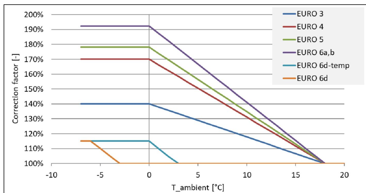
Abbildung 13: Funktion zur Berücksichtigung des Einflusses Umgebungstemperatur auf die Höhe der Stickoxid-Emissionsfaktoren der Diesel-PKW-EURO-3 – EURO-6
