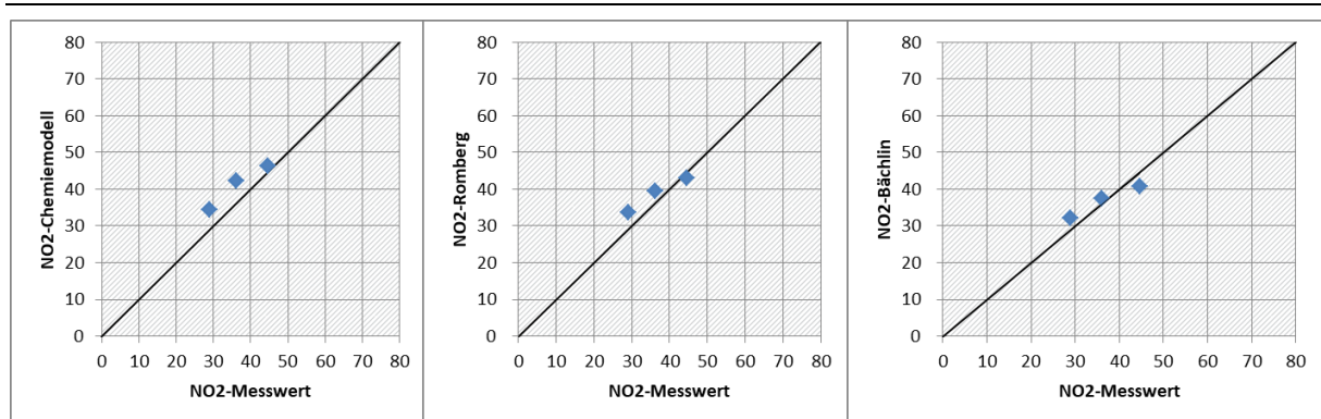
Abbildung 21: Mit MISKAM berechnete NO 2 -Jahresmittelwerte unter Verwendung des Chemiemodells nach Düring et al. (2011) sowie der statistischen Ansätze nach Romberg et. al (1996) sowie Bächlin et al. (2008) für 2015 (höchster Wert), 2018 (mittlerer Wert) und 2019 (niedrigster Wert) in 2.6 m über Grund im Vergleich zu den Messwerten. Werte in µg/m 3 .
