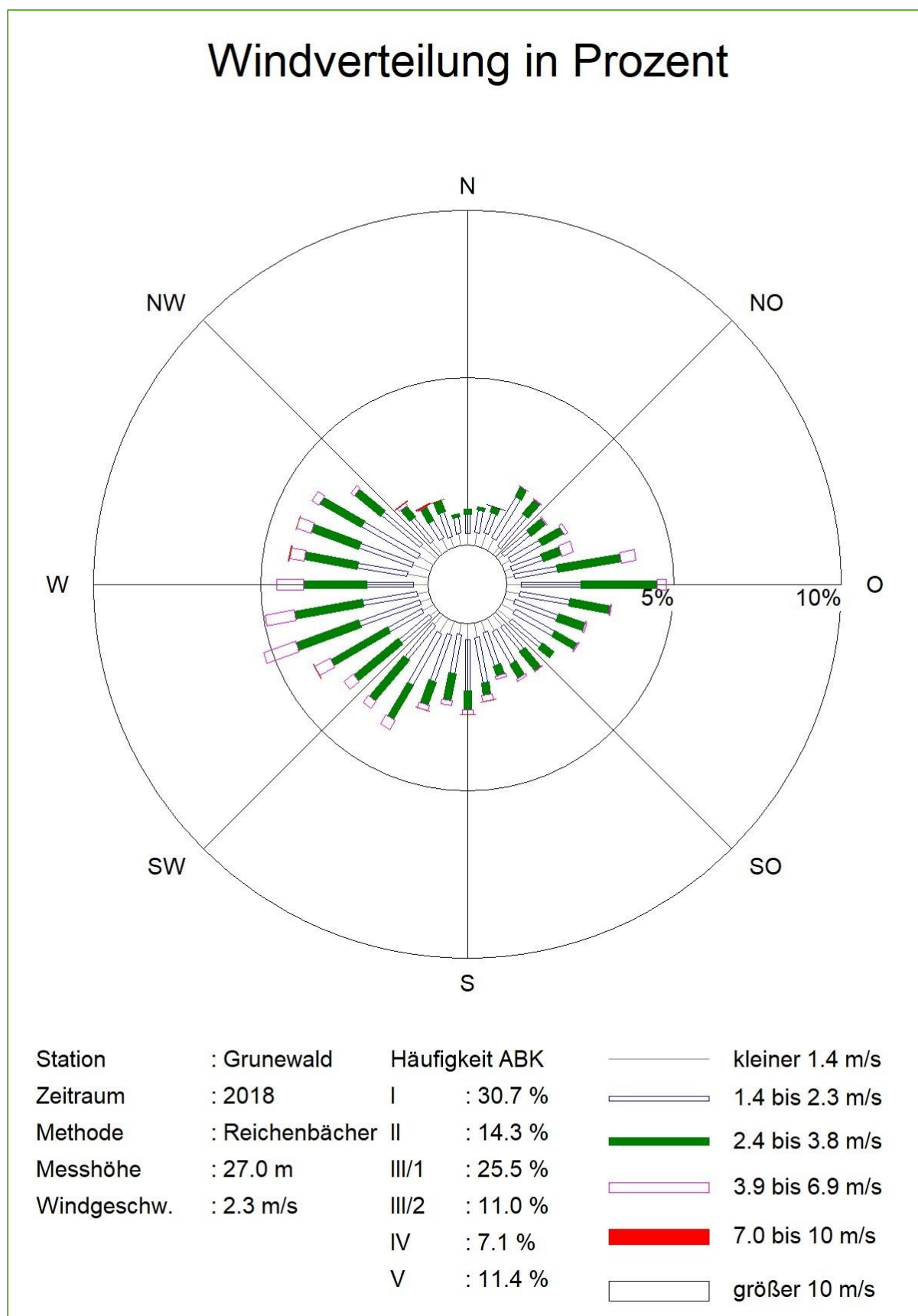
Abbildung 7: Verwendete Wind- und Ausbreitungsklassenstatistik an der Station Grunewald für Bezugsjahr 2018
