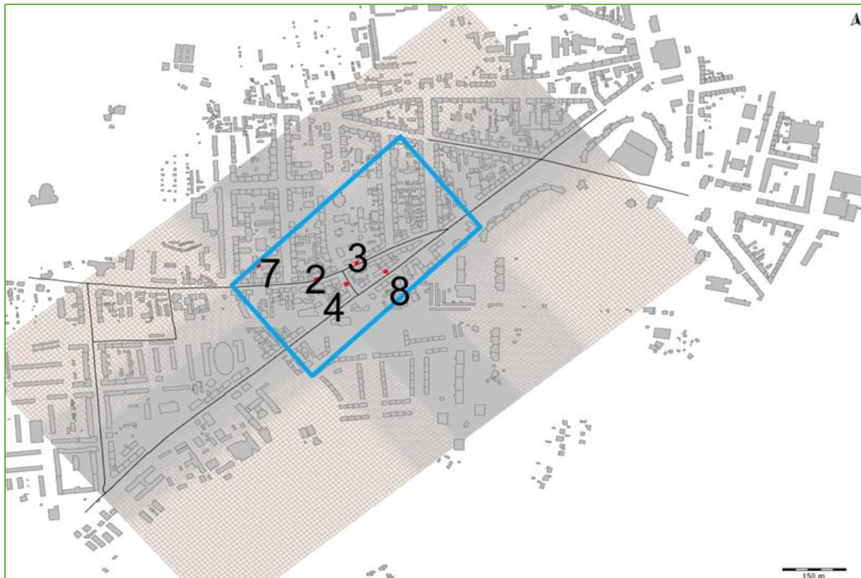
Abbildung 5: MISKAM-Rechengebiet sowie MISKAM-Auswertegebiet. Markiert sind auch Lagen von Messstellen
