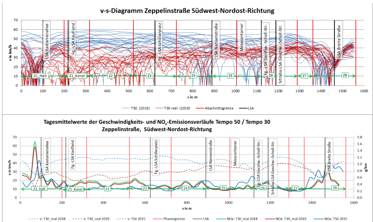
Abbildung 16: Vergleich der Fahrprofile und der NO x -Emissionsverläufe der Vorher- und Nachhersituation: Zeppelinstraße stadteinwärts
