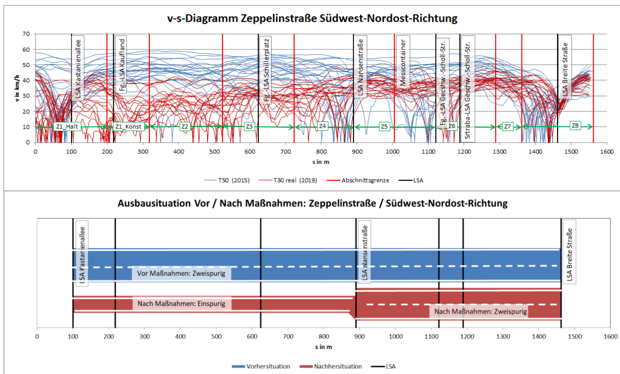
Abbildung 15: Vergleich der Fahrprofile und des Ausbauzustandes der Vorher- und Nachhersituation: Zeppelinstraße stadteinwärts
