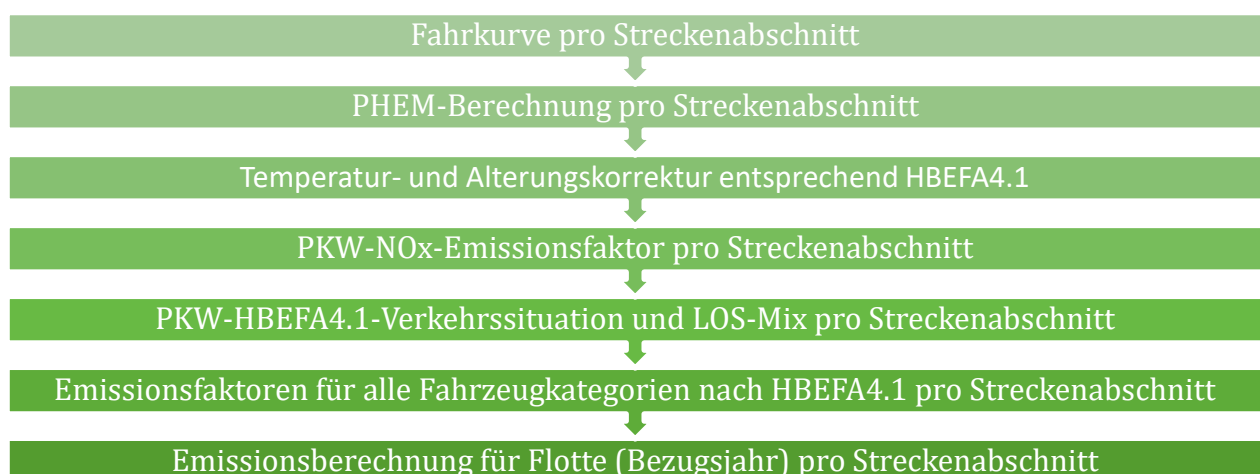
Abbildung 9: Arbeitsablauf für die LOS- und Emissionsberechnung
