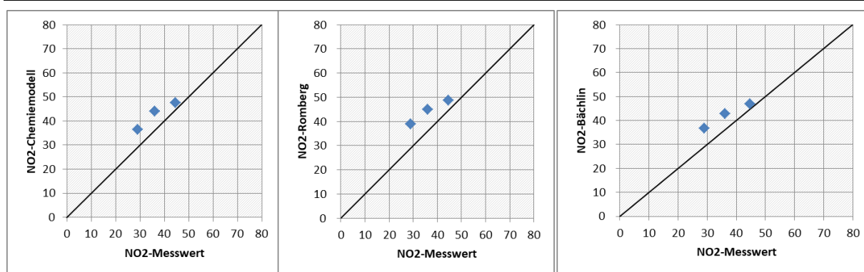
Abbildung 24: Mit PROKAS/PROKAS_B berechnete NO 2 -Jahresmittelwerte unter Verwendung des Chemiemodells nach Düring et al. (2011) mit halbierten NO 2direkt -Anteilen sowie der statistischen Ansätze nach Romberg et. al (1996) sowie Bächlin et al. (2008) für 2015, 2018 und 2019 in 1.5 m über Grund im Vergleich zu den Messwerten in 2.6 m über Grund. Werte in µg/m 3 .
