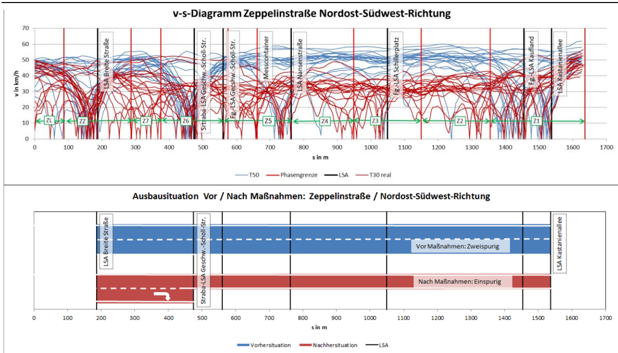
Abbildung 17: Vergleich der Fahrprofile und des Ausbauszustandes der Vorher- und Nachhersituation: Zeppelinstraße stadtauswärts
