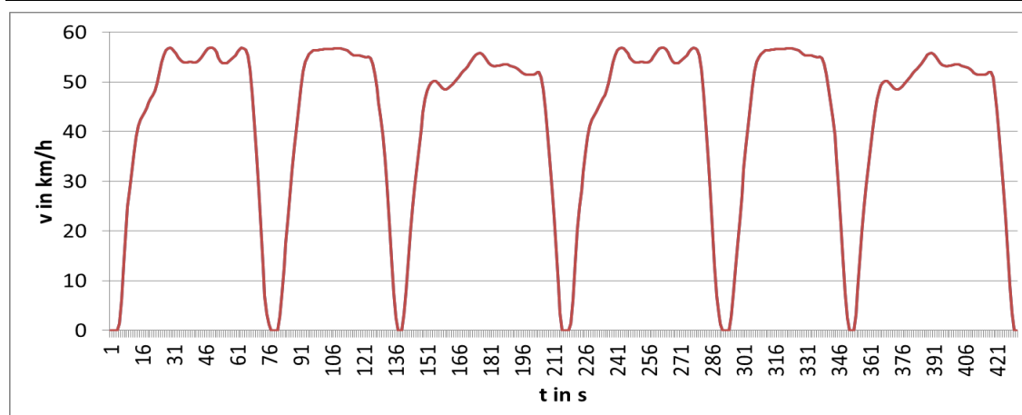
Abbildung 19: Fahrzyklus nach HBEFA4.1 für IOS-HVS50 LOS1 (flüssig)
