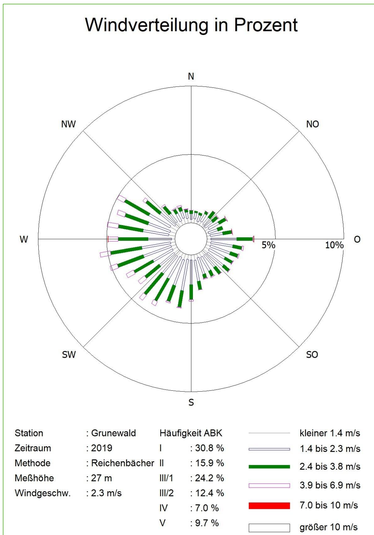
Abbildung 8: Verwendete Wind- und Ausbreitungsklassenstatistik an der Station Grunewald für Bezugsjahr 2019
