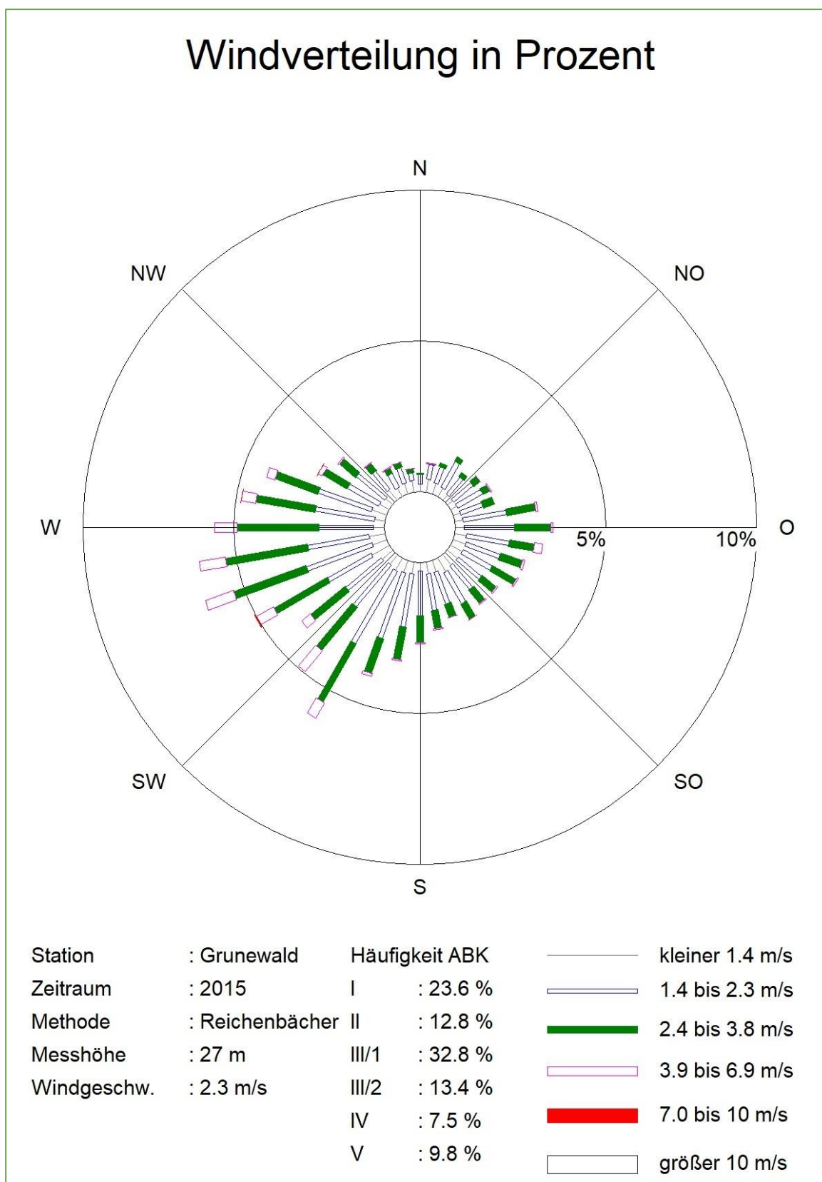
Abbildung 6: Verwendete Wind- und Ausbreitungsklassenstatistik an der Station Grunewald für Bezugsjahr 2015
