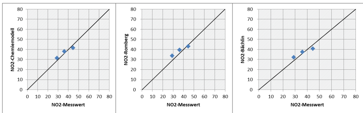
Abbildung 22: Mit MISKAM berechnete NO 2 -Jahresmittelwerte unter Verwendung des Chemiemodells nach Düring et al. (2011) mit halbierten NO 2direkt -Anteilen sowie der statistischen Ansätze nach Romberg et. al (1996) sowie Bächlin et al. (2008) für 2015 (höchster Wert), 2018 (mittlerer Wert) und 2019 (niedrigster Wert) in 2.6 m über Grund im Vergleich zu den Messwerten. Werte in µg/m 3 .
