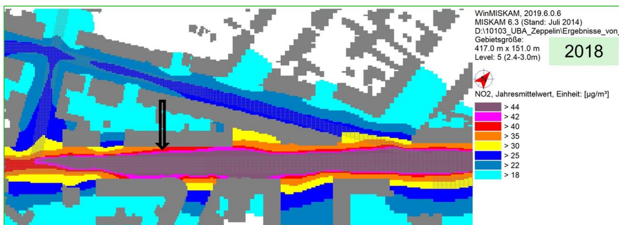
Abbildung 20: Mit MISKAM berechnete NO 2 -Jahresmittelwerte für 2018 in 2,6 m über Grund. NO-NO 2 -Konversion nach Düring et. al (2011) und NO 2 -Direktanteile aus HBEFA4.1
