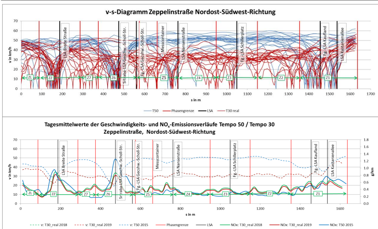
Abbildung 18: Vergleich der Fahrprofile und der NO x -Emissionsverläufe der Vorher- und Nachhersituation: Zeppelinstraße stadtauswärts
