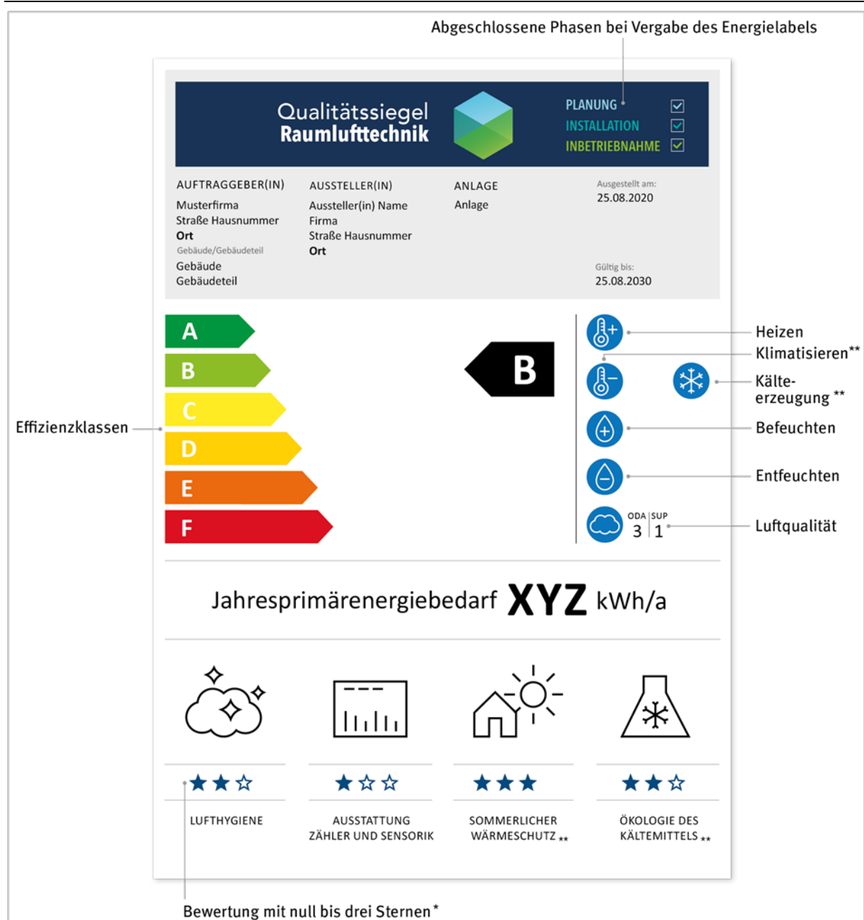
Abbildung 38: Das Energielabel für neue RLT- und Kälteanlagen: Komponenten für eine RLT-Anlage mit kombinierter Kälteanlage
