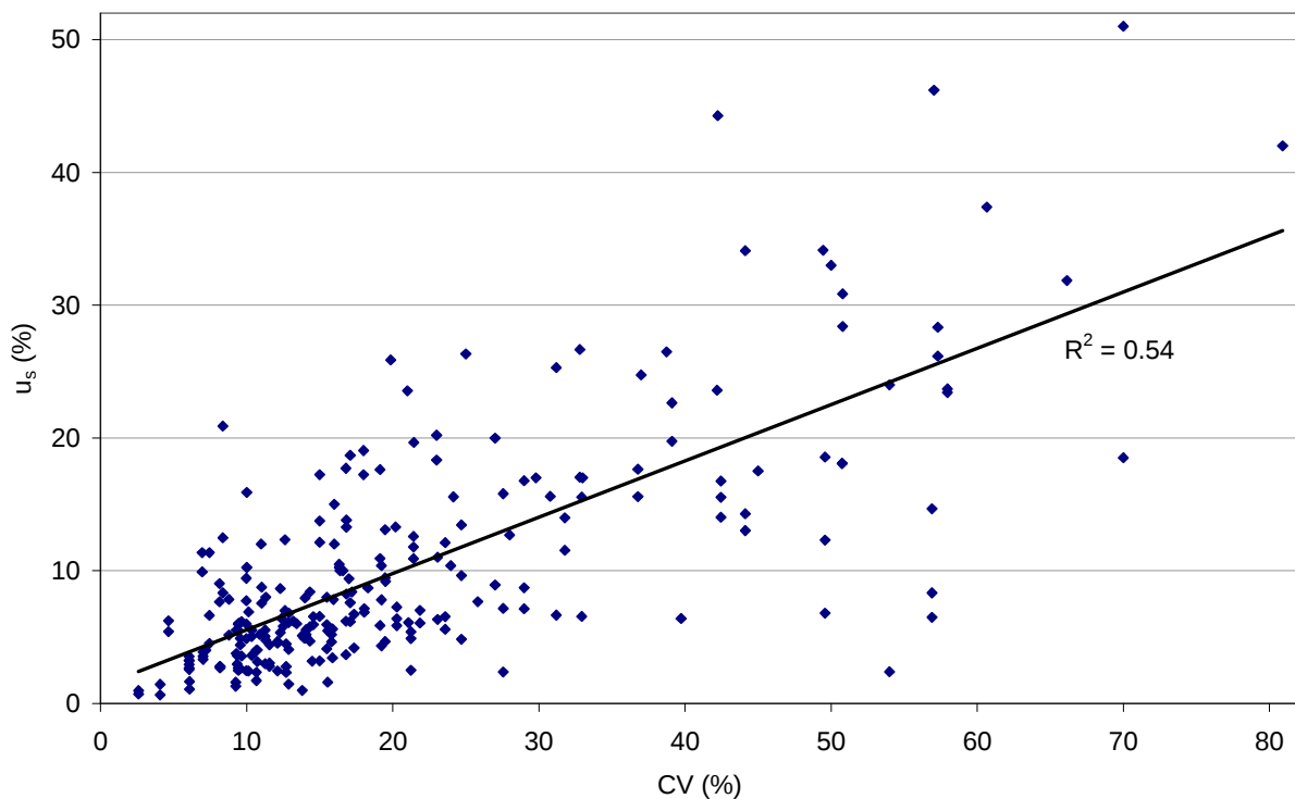
Abbildung 7: u_s -Werte vs CV (d.h., Feldheterogenität).
