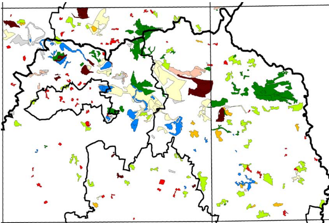
Abbildung 32: Landnutzungsänderungen in den TK100-Blättern Hoyerswerda und Niesky in der Niederlausitz gemäß CLC2000_Change. Die gesamten Änderungen, die meist im Zusammenhang mit dem Braunkohletagebau und nachfolgenden Rekultivierungsmaßnahmen sowie Stilllegungen von Truppenübungsplätzen stehen, betragen hier 12% der Gesamtfläche. Dargestellt sind die Änderungen in zusammengefassten Transformationsklassen. Zur Legende siehe Abbildung 24 bzw. Abbildung 25.
