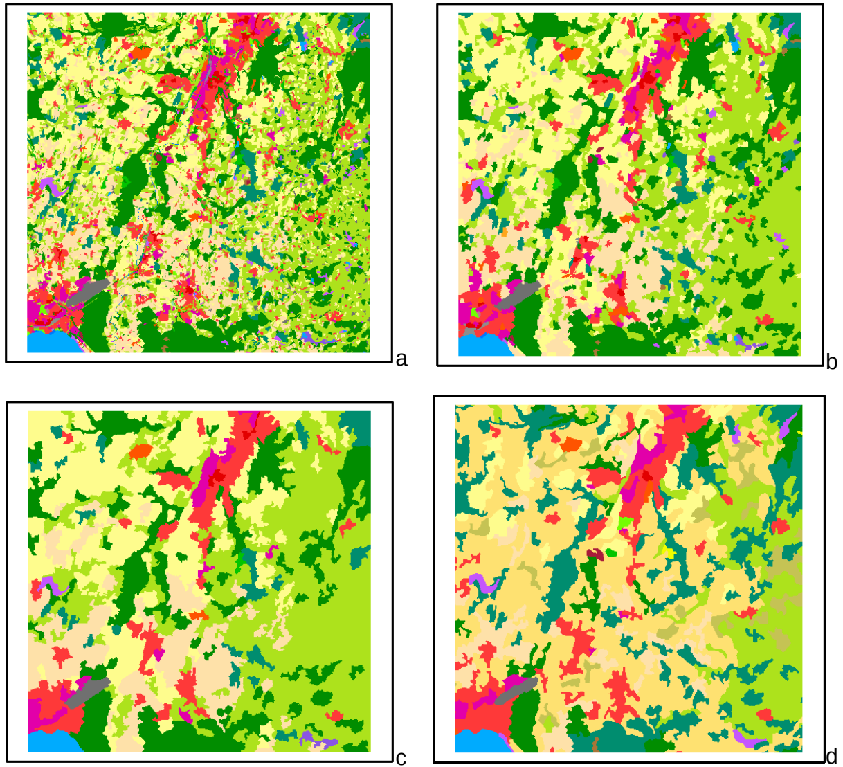
Abbildung 40: Testgebiet Friedrichshafen a) 1 ha MMU; b) 5 ha MMU; c) 25 ha MMU; d) CLC2006 laut EEA, 25 ha MMU
