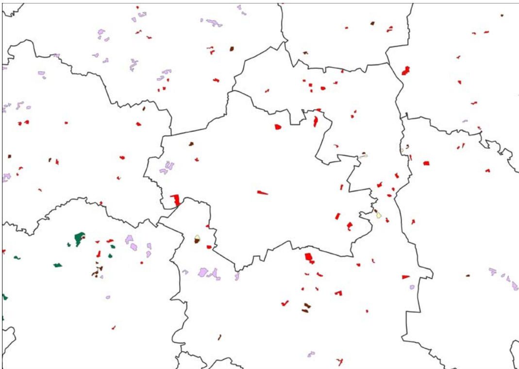
Abbildung 30: Landnutzungsveränderungen zum Status CLC2006 im Großraum München (Legende siehe Abbildung 24 bzw. Abbildung 25)
