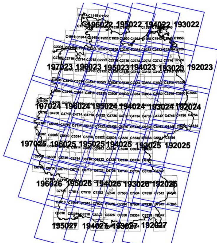
Abbildung 2: Landsat-Überdeckung von Deutschland in der Datenbasis IMAGE2000, mit den Kartierungs-einheiten der TK100. Dabei entsprechen die ersten drei Ziffern der Szenenbezeichnung dem Path, die letzten beiden Ziffern der Row der Landsat7 ETM+ Daten.
