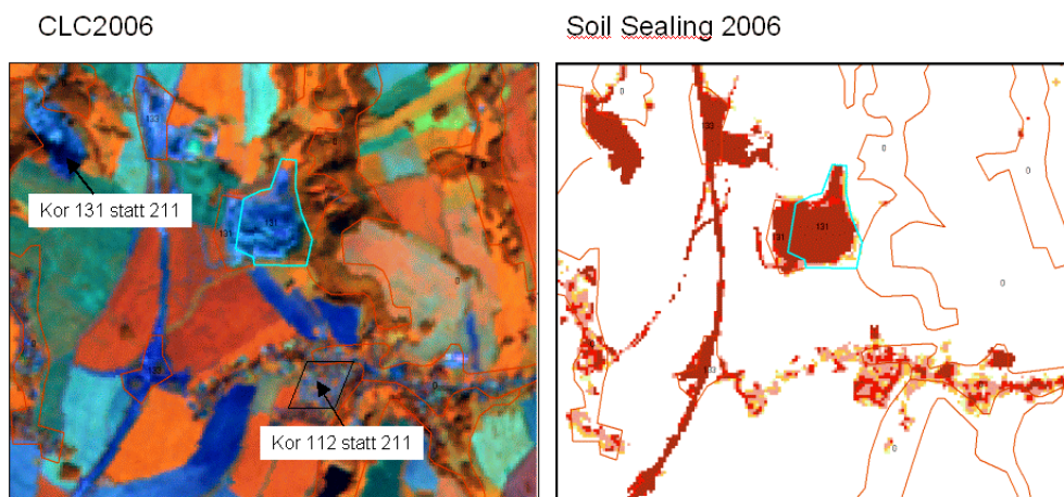
Abbildung 14: Beispiel für den Einsatz des Soil Sealing Layers zur Überarbeitung bzw. Änderungserfassung von bebauten Flächen und Abbauflächen.
