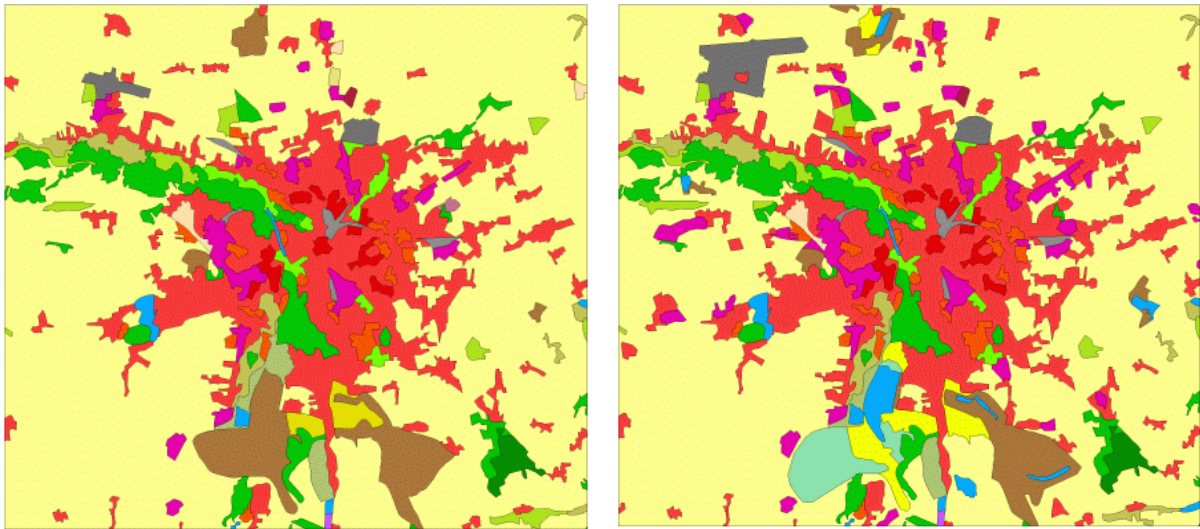
Abbildung 22: Ergebnisse der Interpretation CLC1990_rev (links) und CLC2000 (rechts) für die Region Leipzig. Die Farbgebung entspricht der Farblegende aus Abbildung 4.
