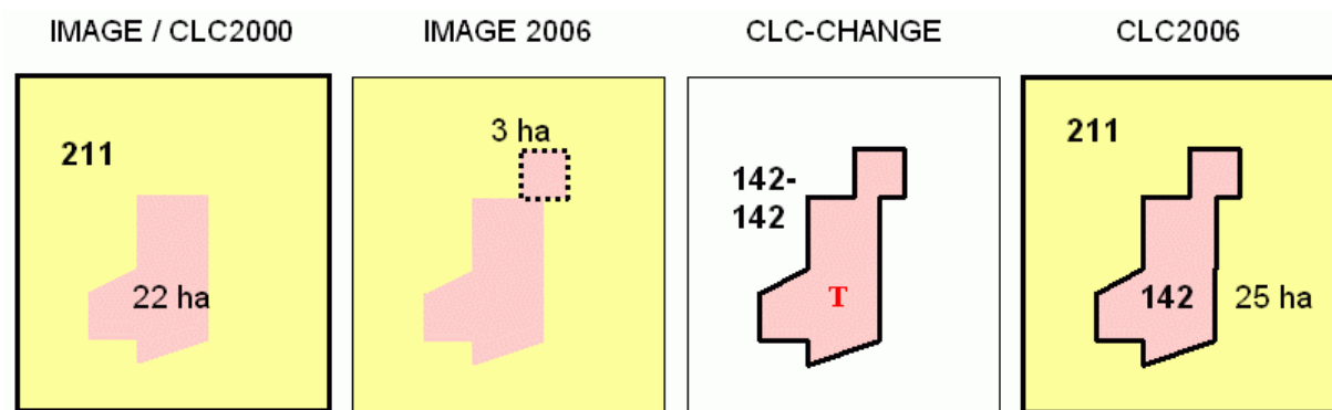
Abbildung 7: Einsatz einer technischen Änderung bei neuer Erholungsfläche. In diesem Beispiel wird das Gesamtpolygon (mit der Altfläche von 22 ha und der Änderung 3 ha, also unter den 5 ha Mindesterfassungsfläche im Change-Layer) als technische Änderungsfläche erfasst, um die Erholungsfläche 142 in CLC2006 erfassen zu können.
