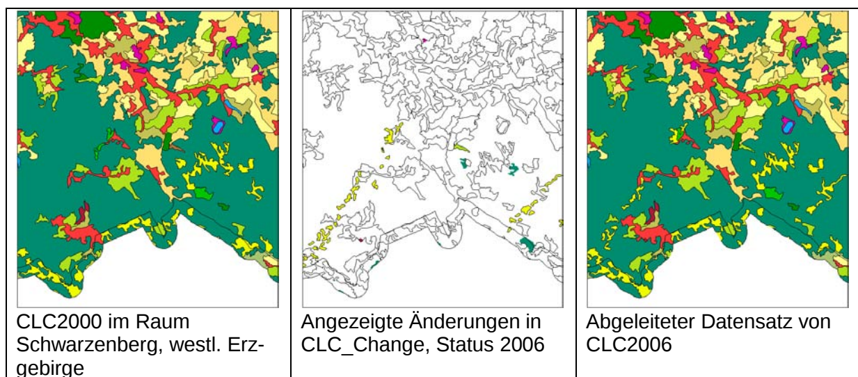
Abbildung 35: Die resultierenden Vektordaten der Region Schwarzenberg, westliches Erzgebirge. Als hauptsächliche Änderungen zwischen 2000 und 2006 werden neue Flächen in der Klasse 324 (Wald-Strauch-Übergangsstadien) angezeigt.
