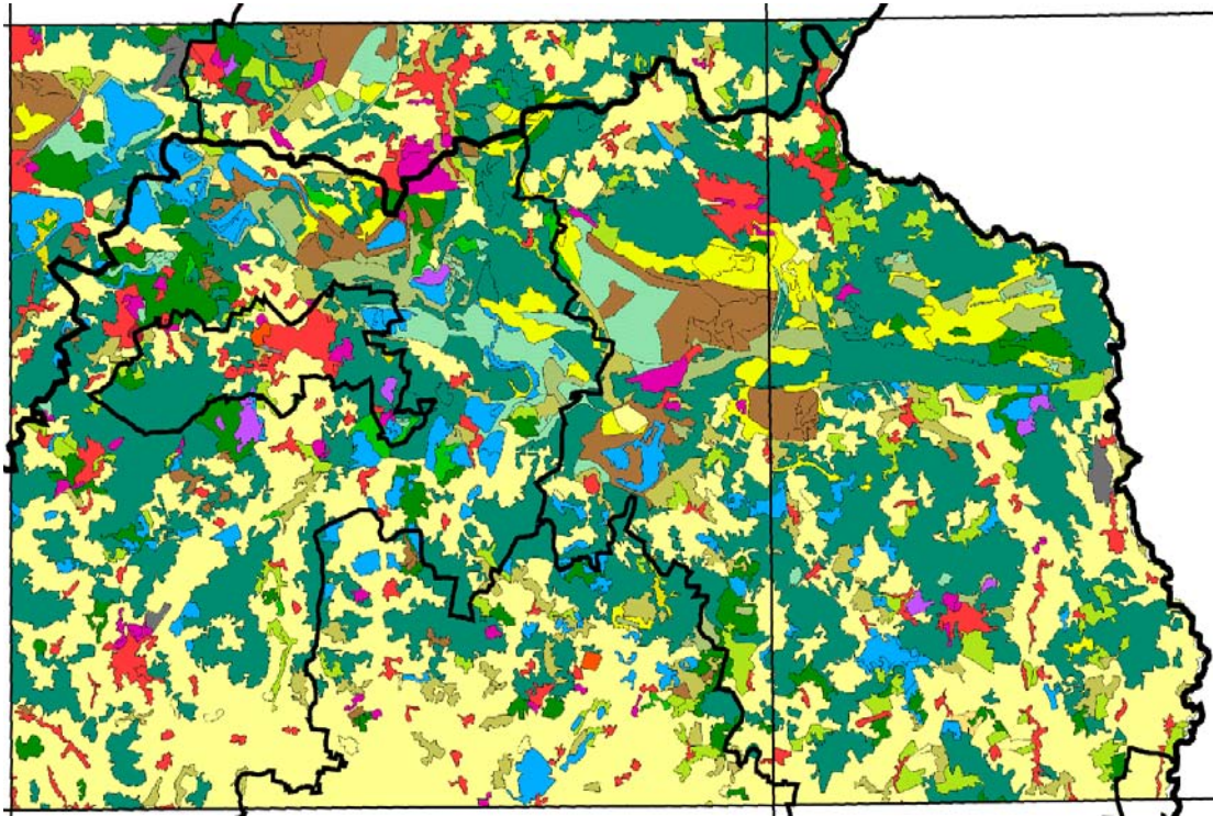
Abbildung 31: Bodenbedeckung laut CLC2000 in den TK100-Blättern Hoyerswerda und Niesky in der Niederlausitz. Legende siehe Abbildung 4.
