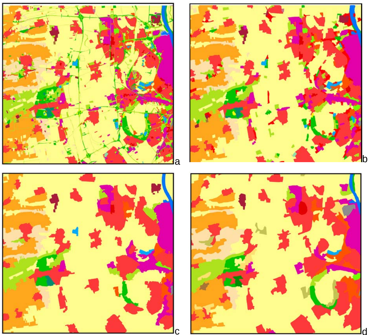
Abbildung 36: Subregion Frankenthal, a) aktualisiertes DLM-DE, 1 ha MMU; b) aktualisiertes DLM-DE, 5 ha MMU; c) aktualisiertes DLM-DE, 25 ha MMU; d) CLC2006 laut EEA, 25 ha MMU
