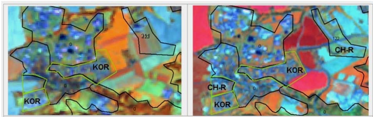
Abbildung 16: Beispiel für das Nebeneinander von Korrekturen und realen Änderungen bei der Aktualisierung bebauter Flächen.
