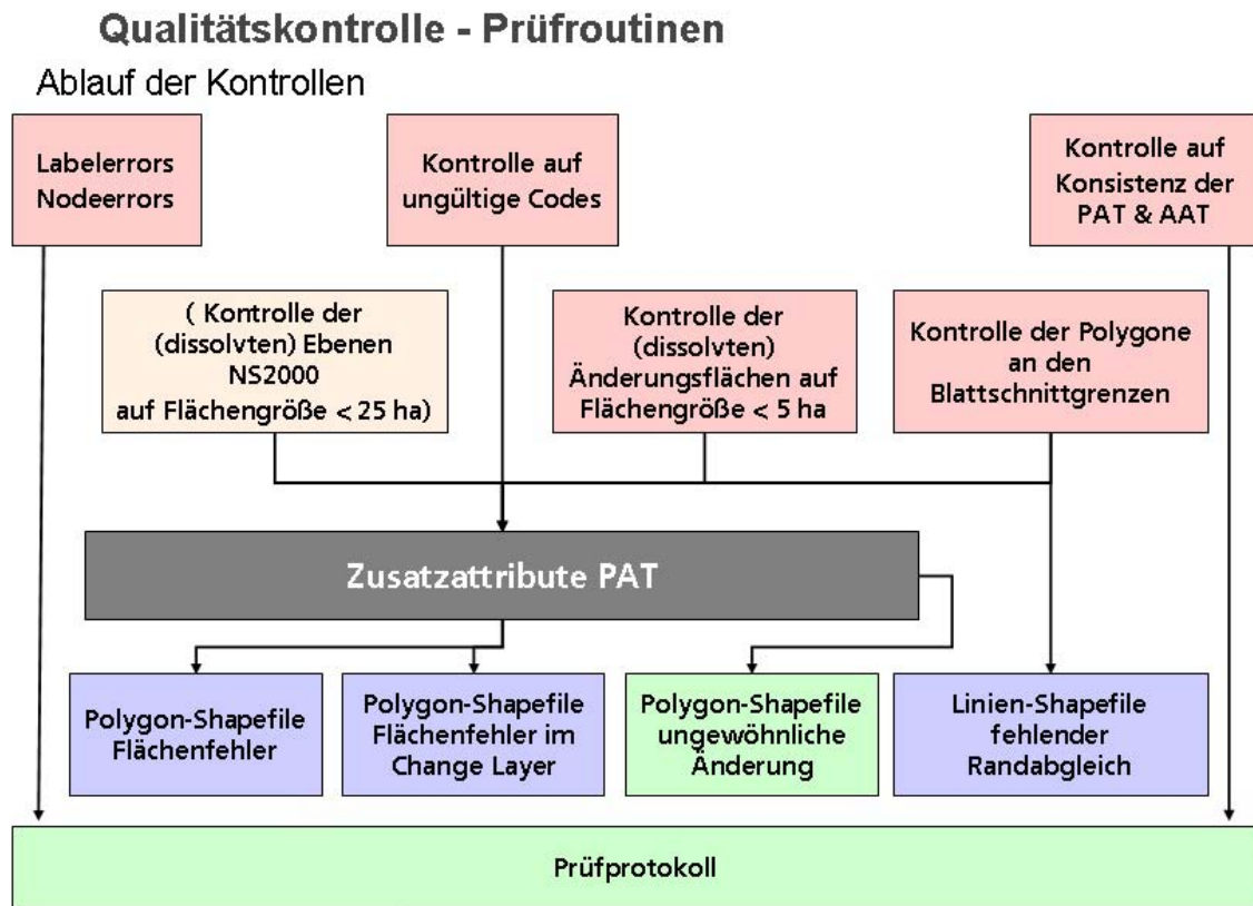
Abbildung 11: Ablauf der technischen Kontrolle der Interpretations- und Kartierungsergebnisse am DFD
