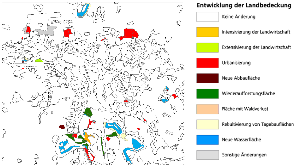
Abbildung 25: Die Region Leipzig in abgeleiteten Entwicklungen der Landbedeckung zwischen 2000 (bzw. 1999) und 2006 in generalisierten Transformationsklassen, siehe nebenstehende Legende
