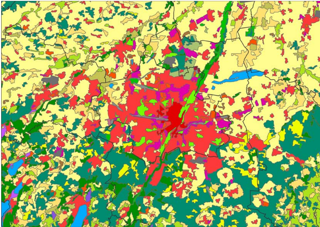
Abbildung 29: Bodenbedeckung laut CLC2006 für den Großraum München (Legende siehe Abbildung 4)
