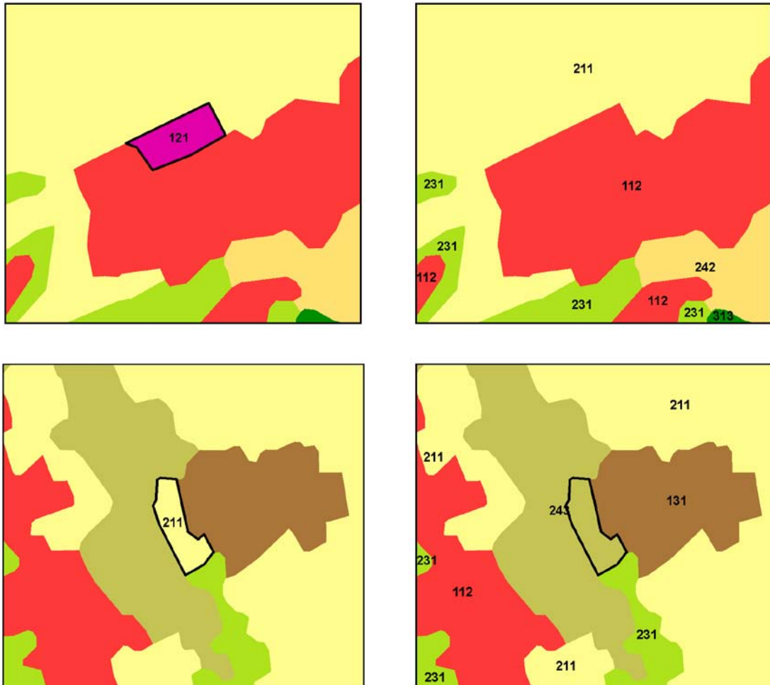
Abbildung 9: Beispiele der automatischen Aggregation zu kleiner entstandener CLC2006-Polygone. Die automatische Zuweisung konnte akzeptiert werden.
