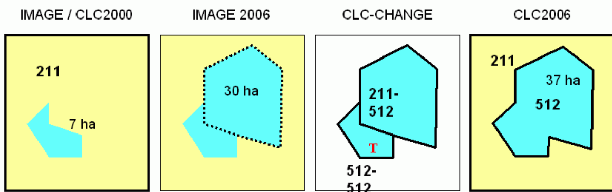
Abbildung 6: Beispiel zur Einführung eines Polygons mit technischer Änderung (Ch-T 512-> 512), um die frühere Wasserfläche von 7 ha (diese war aus Generalisierungsgründen mit einer Fläche unter 25 ha nicht in CLC2000 erfasst) für die Gesamtfläche des Gewässers in CLC2006 einbeziehen zu können.
