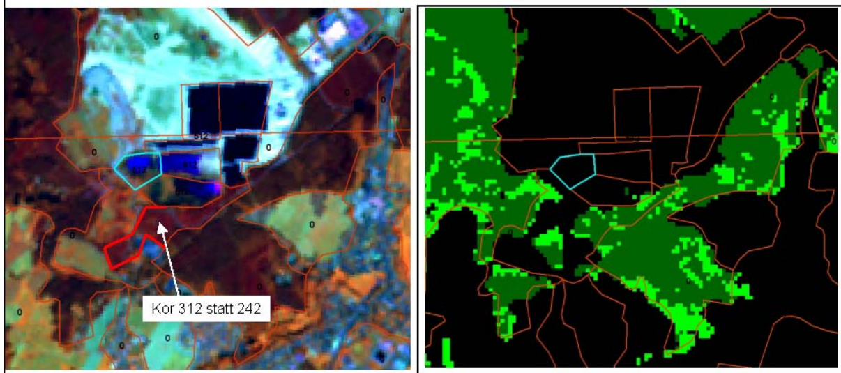
Abbildung 15: Beispiel für den Einsatz des GMES-Forest-Layers als Zusatzinformation bei der Abgrenzung von Waldflächen und landwirtschaftlich genutzten Flächen.
