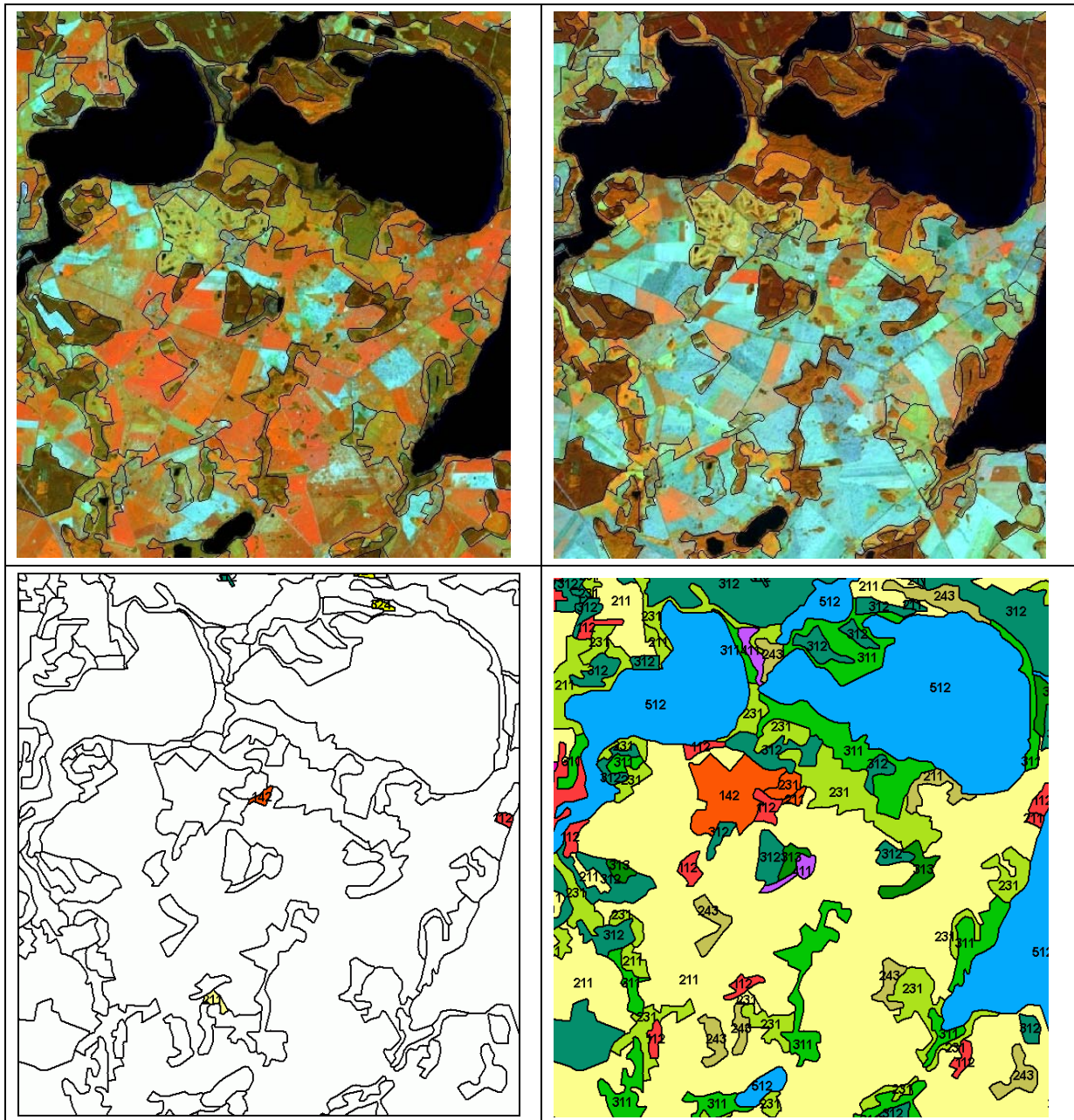
Abbildung 18: Vorteile der multisaisonalen Datengrundlage: Die LISS-III- Szenen aus Mai 2006 (oben links) und September 2006 (oben rechts) machen das erhöhte Potential multisaisonaler Datensätze bei der Abgrenzung von Grünland und Ackerland deutlich, hier für eine Region westlich des Müritz-Sees in Mecklenburg. Die abgeleiteten Veränderungen (links) und der Status in 2000 (rechts) sind im unteren Bereich dargestellt.
