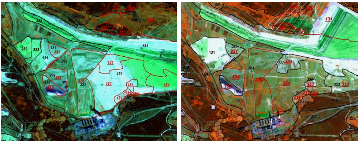
Abbildung 17: Tagebauflächen im Wandel, dargestellt für eine Region in Sachsen. Links: CLC-Polygone in 2000 über Landsat-Daten von 2000 (IMAGE2000), rechts: CLC-Polygone in 2006 über den Satellitendaten von IMAGE2006. Neben den schwarzen Abgrenzungen und Beschriftungen des Status 2000 / 2006 sind die Änderungsflächen (zum Status von 2000 / 2006) in rot eingetragen.
