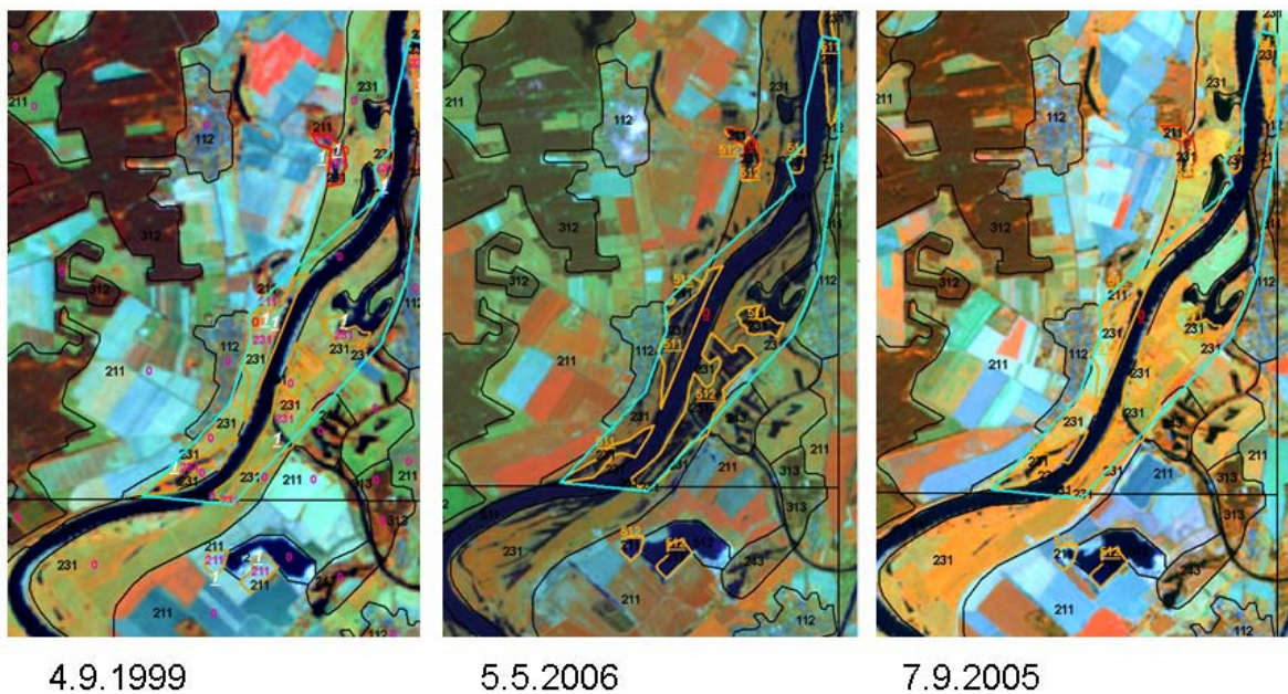
Abbildung 21: Beispiel für temporäre Wasserstände. Das Nebeneinander von Sommer- und Frühjahrsszenen macht deutlich, dass die abgegrenzten neuen Wasserflächen in der Elbaue in der Mai-Szene 2006 nicht als Transformationen der Landbedeckung, sondern nur als temporäre Situationen nach einem Hochwasser zu werten sind und die Änderungen eliminiert werden mussten.
