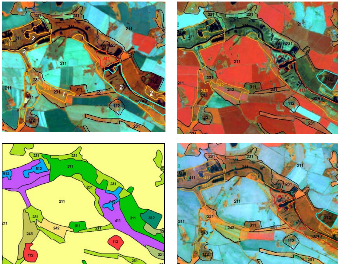
Abbildung 20: Vorteile der multisaisonalen Datengrundlage, Teil 2: Landsat-Subszene von August 2000 (links) sowie von Mai 2006 (r.o.) und Juli 2006 (r. u.) mit der Abgrenzung von Feuchtgebieten (421), Wiesen (231) und Waldgebieten (311, 312). Für die Abgrenzung der Übergänge sind mehrere Jahreszeiten und oft Referenzdaten mit feinerer Auflösung/ Textur notwendig.
