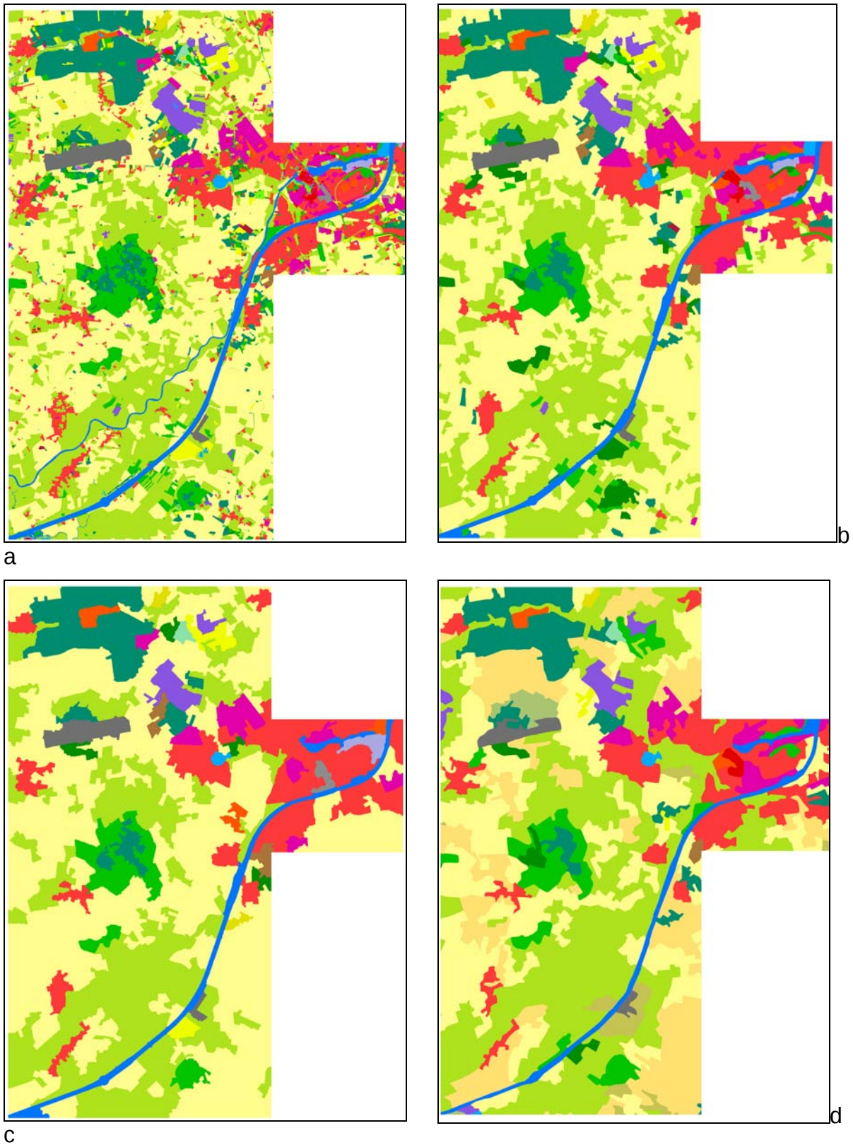
Abbildung 37: Testgebiet Rendsburg a) aktualisiertes DLM-DE, 1 ha MMU; b) aktualisiertes DLM-DE, 5 ha MMU; c) aktualisiertes DLM-DE, 25 ha MMU; d) CLC2006 laut EEA, 25 ha MMU
