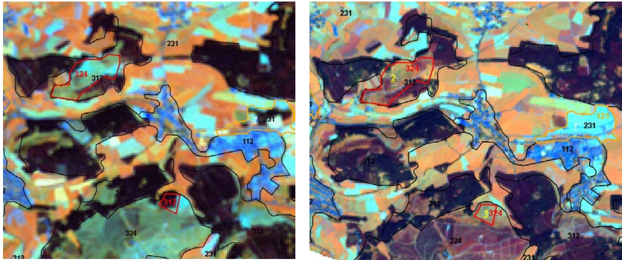
Abbildung 19: Waldstadien in der Interpretation von Satellitendaten aus 2000 (links) und 2006 (rechts): Die große Aufforstungsfläche im Süden (324 in 2000) kann auch in 2006 gerade noch diesem Stadium zugeordnet werden, d. h. sie ist keine Änderungsfläche. Im oberen Teil dieser Fläche ist aus dem restlichen Altbestand ein Polygon der Klasse Wald-Strauch-Übergang (324), also eine reale Änderung, geworden.
