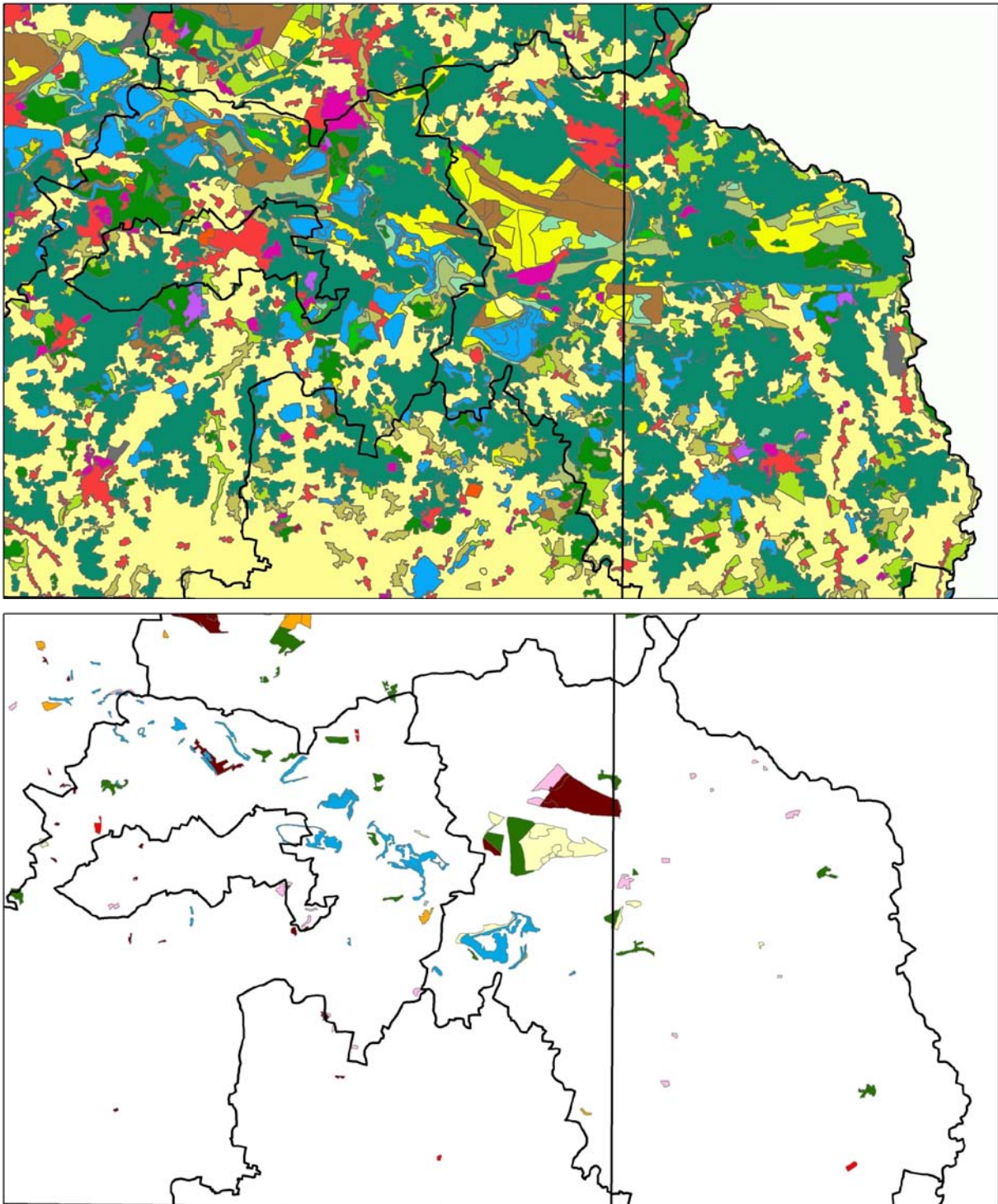
Abbildung 33: Bodenbedeckung zum Status 2006 (oben) und Landnutzungsänderungen (unten) in den TK100-Blättern Hoyerswerda und Niesky in der Niederlausitz zwischen 2000 und 2006. Dargestellt für die Änderungen sind wiederum zusammengefasste Transformationsklassen. Als hauptsächlicher Änderungsprozess sind die gefluteten ehemaligen Tagebauflächen zu erkennen (zur Legende für die obere Abbildung siehe Abbildung 4, zur Legende für die untere Abbildung siehe Abbildung 24 bzw. Abbildung 25).
