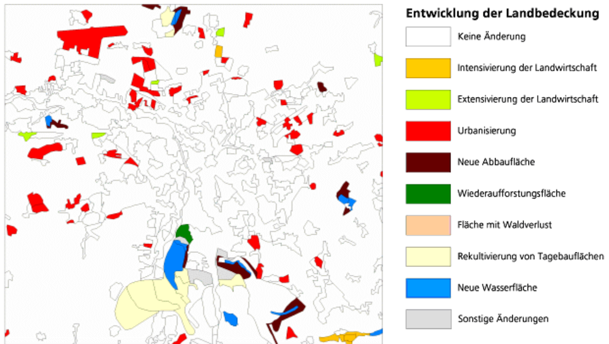
Abbildung 24: Die Region Leipzig in abgeleiteten Entwicklungen der Landbedeckung zwischen 1990 und 2000 (bzw. 1999) in generalisierten Transformationsklassen, siehe nebenstehende Legende; nach: Keil et al., 2005a
