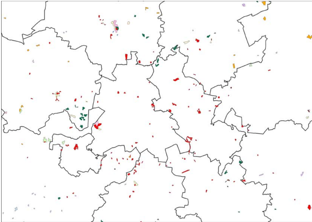
Abbildung 28: Veränderungen der Landbedeckung zwischen 2000 und 2006 in der Metropolregion Berlin (zur Legende siehe Abbildung 24 bzw. Abbildung 25)
