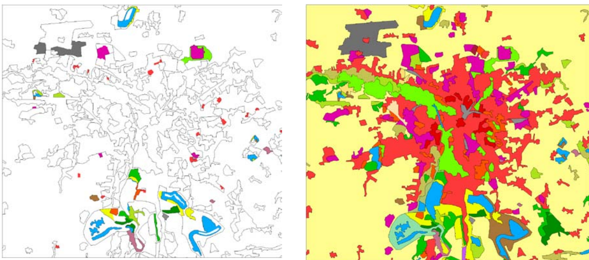
Abbildung 23: Ergebnisse der Interpretation der Änderungen zwischen 2000 und 2006, CHANGE_CLC_2006 (links) und des abgeleiteten Datensatzes CLC2006 (rechts) für die Region Leipzig. Die Farbgebung entspricht der Farblegende aus Abbildung 4.
