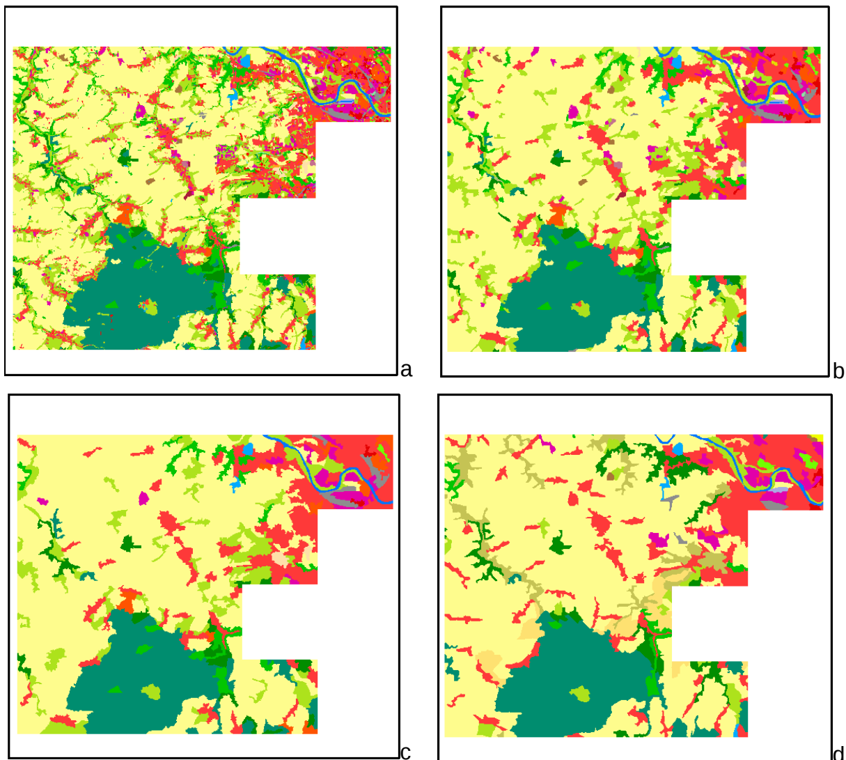
Abbildung 39: Testgebiet Dresden a) 1 ha MMU; b) 5 ha MMU; c) 25 ha MMU; d) CLC2006 laut EEA, 25 ha MMU
