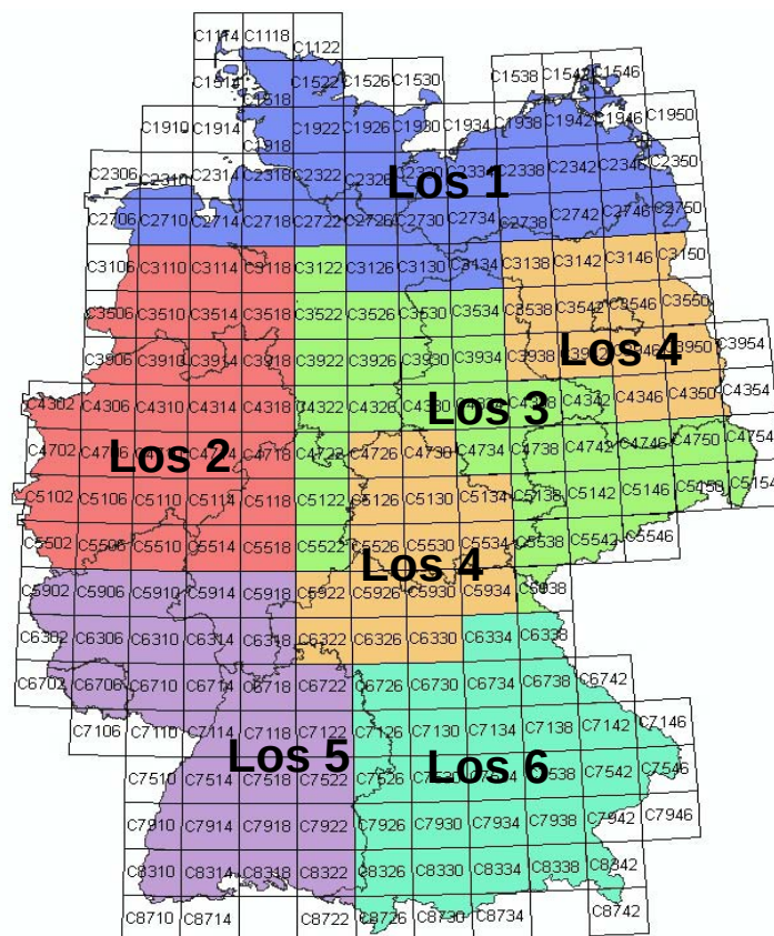
Abbildung 1: Aufteilung der Lose in den Phasen 1 und 2. Neben der Erstreckung der Lose 1 bis 3 (Phase 1) und der Lose 4 bis 6 (Phase 2) sind die Kartiereinheiten der TK100 dargestellt. Beteiligung der Firmen in Phase 1: Los 1: GAF, Los 2: EFTAS, Los 3: Infoterra; in Phase 2: Los 4 & 5: Infoterra, Los 6: EFTAS.
