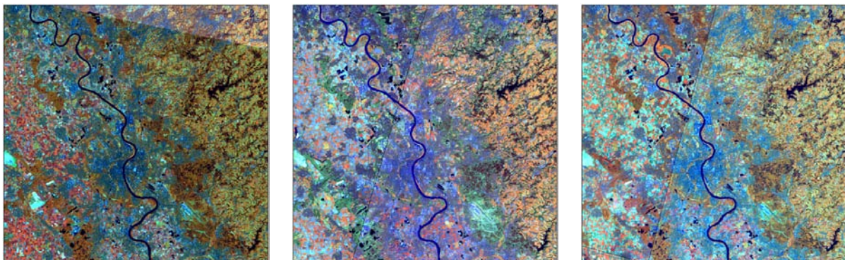
IMAGE2000-Datensatz: Landsat-7 ETM+, v. 15.5.2000 (im N) und 5.7.2001 (im S)
