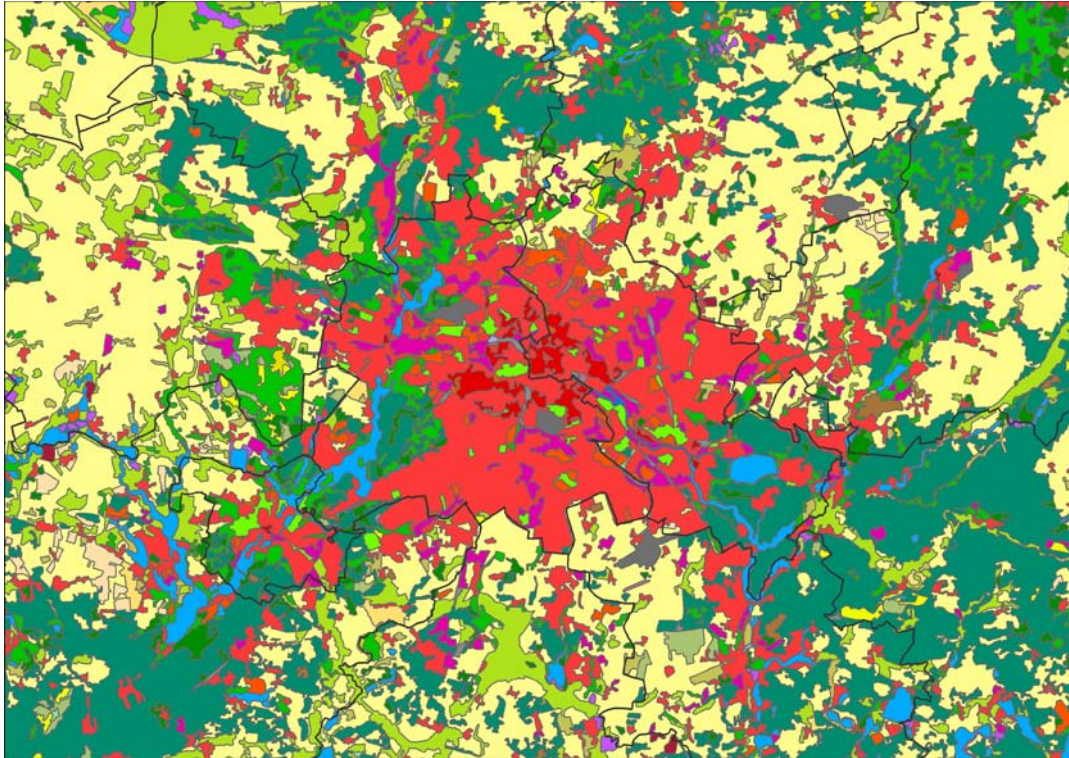
Abbildung 27: Landbedeckung zum Status 2006 in der Metropolregion Berlin (zur Legende siehe die Abbildung 4)
