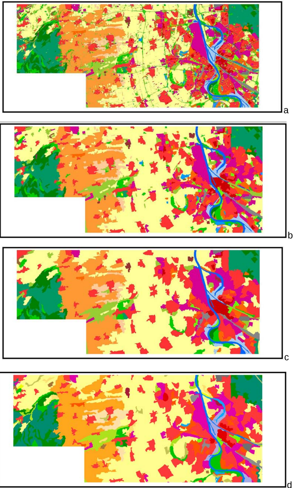
Abbildung 38: Testgebiet Mannheim a) aktualisiertes DLM-DE, 1 ha MMU; b) aktualisiertes DLM-DE, 5 ha MMU; c) aktualisiertes DLM-DE, 25 ha MMU; d) CLC2006 laut EEA, 25 ha MMU
