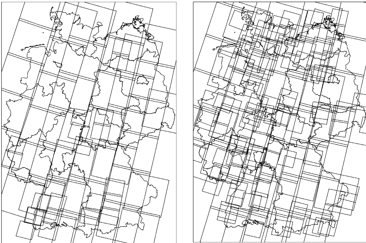
Abbildung 3: Überdeckung von Deutschland in der Datenbasis IMAGE2006 mit den Daten von SPOT-4 und SPOT-5 MS sowie von IRS-P6 LISS III, links die Frühjahrsüberdeckung und rechts die Sommerüberdeckung
