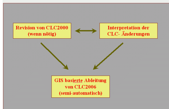
Abbildung 5: Schematische Darstellung der beiden unterschiedlichen Ansätze zur Aktualisierung von CLC
