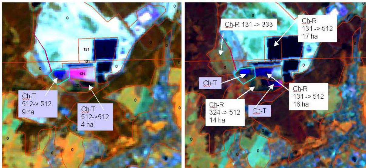
Abbildung 8: Einsatz von technischen Änderungen („technical changes“ - Ch-T) neben realen Änderungen („real changes“ – Ch-R) bei der Entwicklung in einem Tagebaugebiet (Tagebau: CLC-Code 131).
