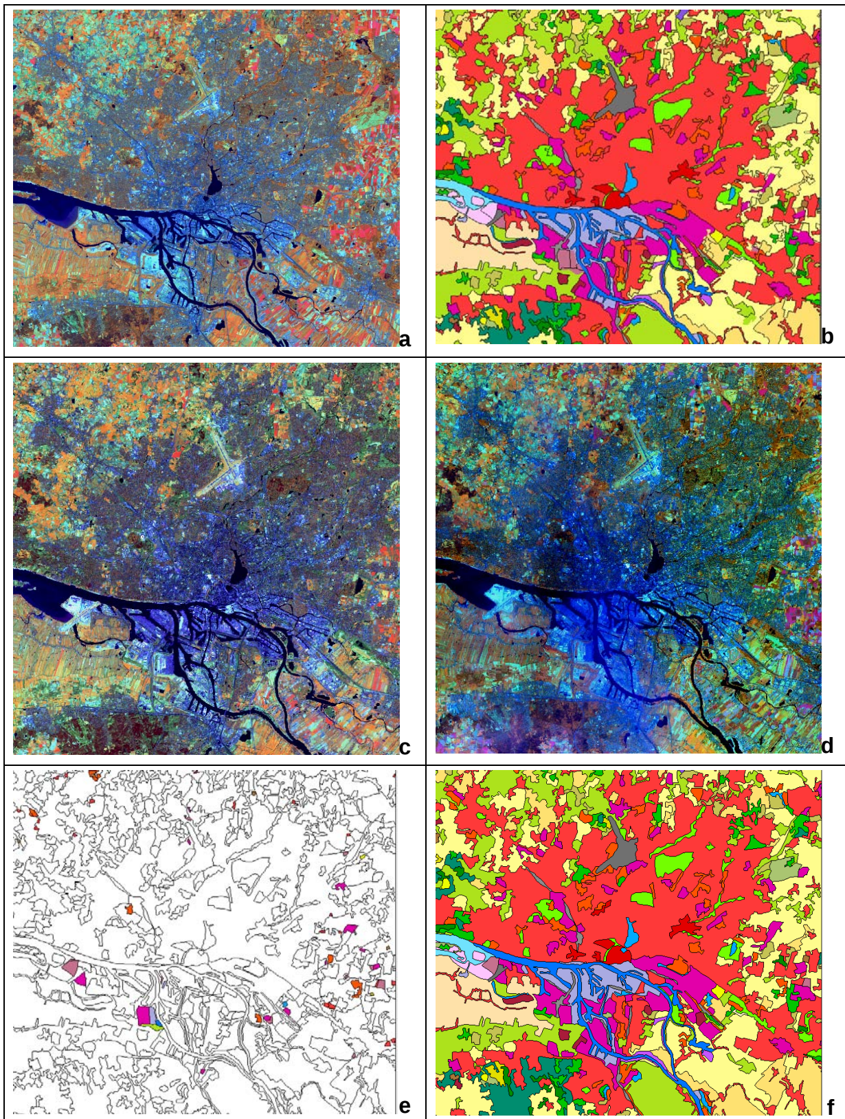
Abbildung 26: Darstellung der Region Hamburg bei der Aktualisierung von CLC. Landsat-Szene aus 2000 (a), CLC2000_kor (b); IMAGE2006 – Frühjahr (c), IMAGE2006 – Sommer (d); CLC_Change zum Status 2006 (e), CLC2006 (f). Erkennbar bei den Änderungen ist insbesondere der neue Containerhafen von Altenwerder.
