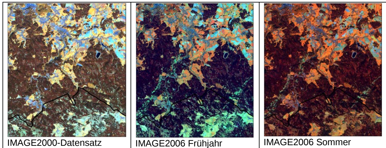
Abbildung 34: Beispiel von Änderungen in Waldgebieten in der Region westliches Erzgebirge südlich Schwarzenberg - die Satellitendaten für die Interpretation und Kartierung der Änderungen. Links: Landsat-7 Datensatz aus IMAGE2000; Mitte: Frühjahrsszene aus IMAGE2006; rechts: Sommerszene aus IMAGE2006. Das Beispiel bezieht sich auf die Region westliches Erzgebirge südlich Schwarzenberg.
