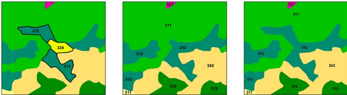
Abbildung 10: Komplexe Ausgangssituation bei Waldflächen im abgeleiteten CLC2006 (links), mit nicht befriedigender Aggregation (Mitte) und der korrigierten Aggregation (rechts).
