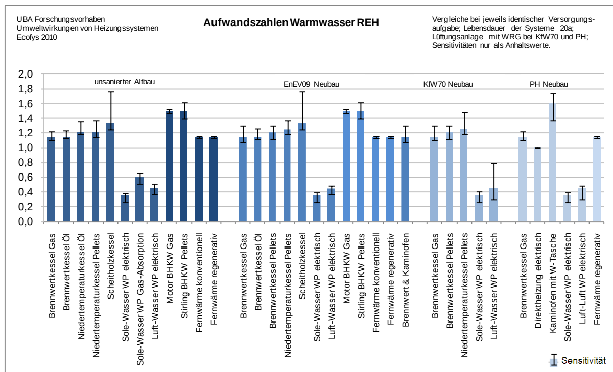
Abb. 29: Aufwandszahlen zur Warmwasserbereitstellung im Einfamilienhaus
