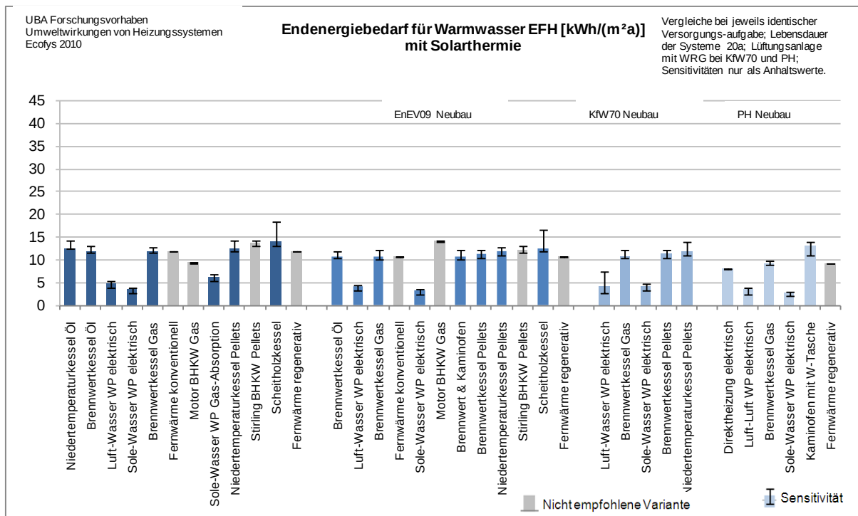
Abb. 14: Endenergiebedarf Warmwasser EFH (mit Solarthermie)
