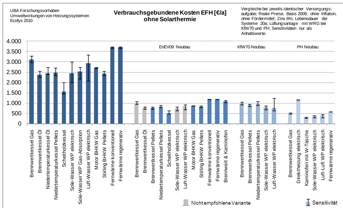
Abb. 7: Verbrauchsgebundene Kosten im Einfamilienhaus (ohne Solarthermie)
