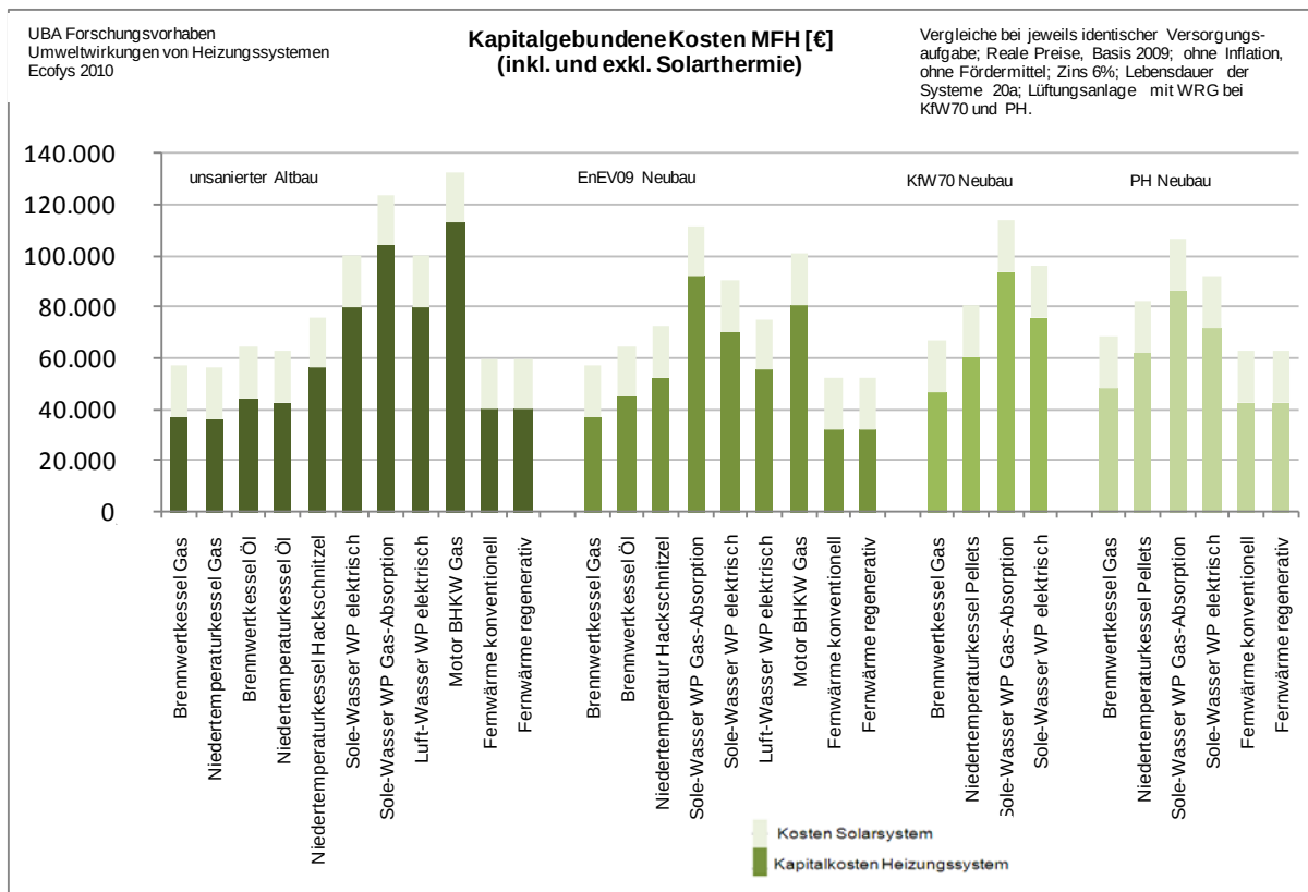
Abb. 4: Kapitalgebundene Kosten im Mehrfamilienhaus
