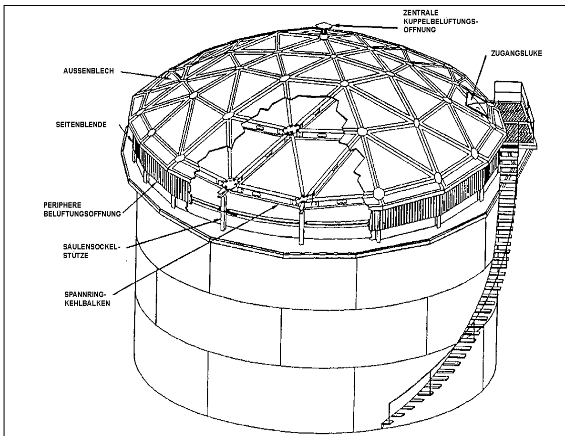
Abbildung 4.1: Schwimmdachtank, ausgerüstet mit einer geodätischen Aluminiumkuppel [166, EEMUA, 2003]
