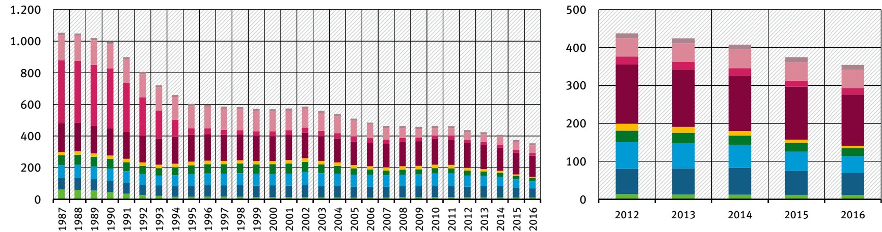
Chrom-Einträge in Tonnen/Jahr
