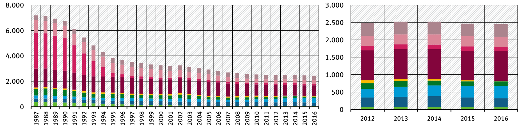
Kupfer-Einträge in Tonnen/Jahr
