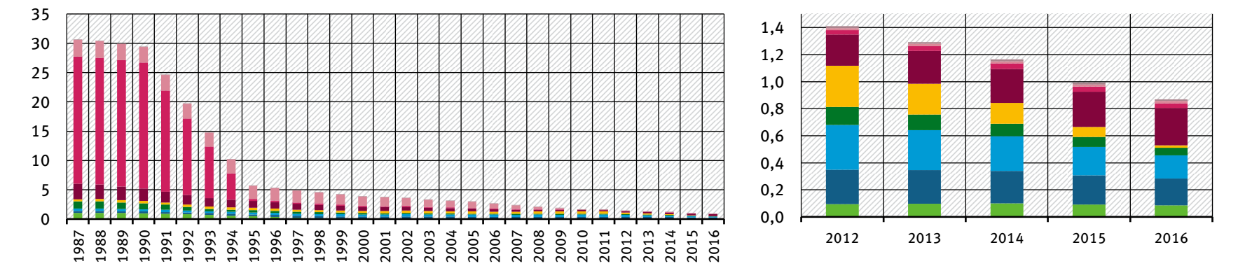
Nickeleinträge als 5-jährige gleitende Mittel in Tonnen/Jahr
