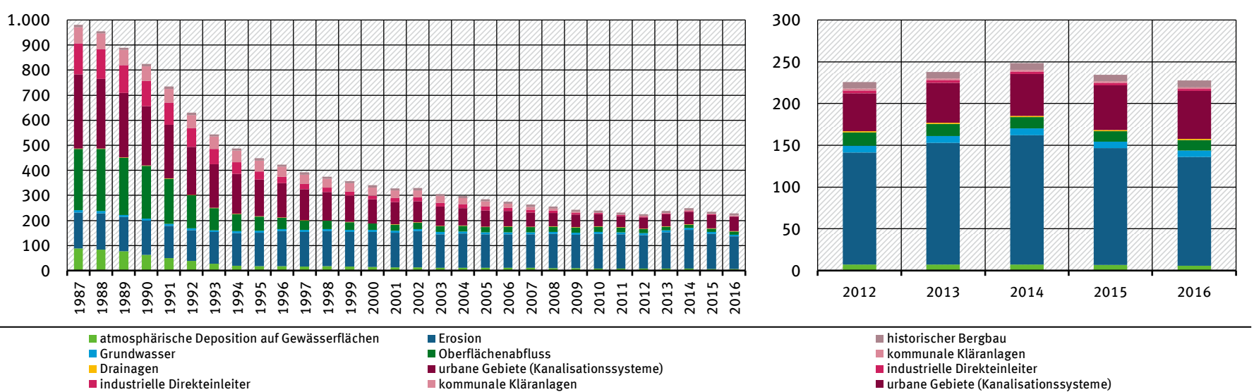
Bleienträge als 5-jährige gleitende Mittel in Tonnen/Jahr
