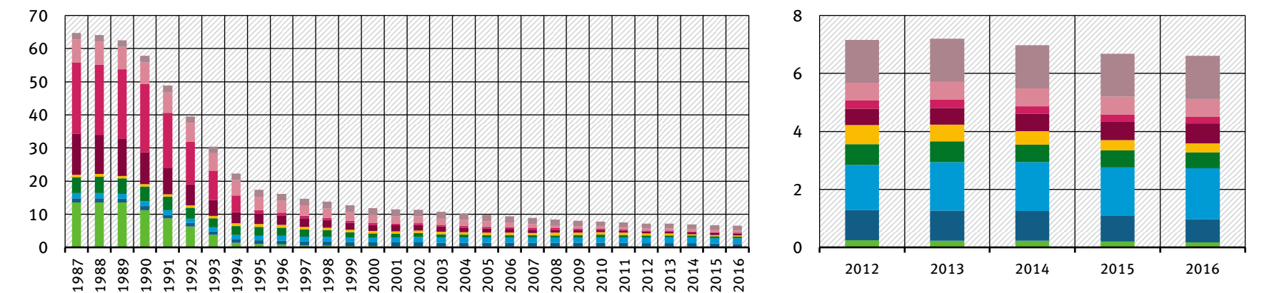
Bleienträge als 5-jährige gleitende Mittel in Tonnen/Jahr
