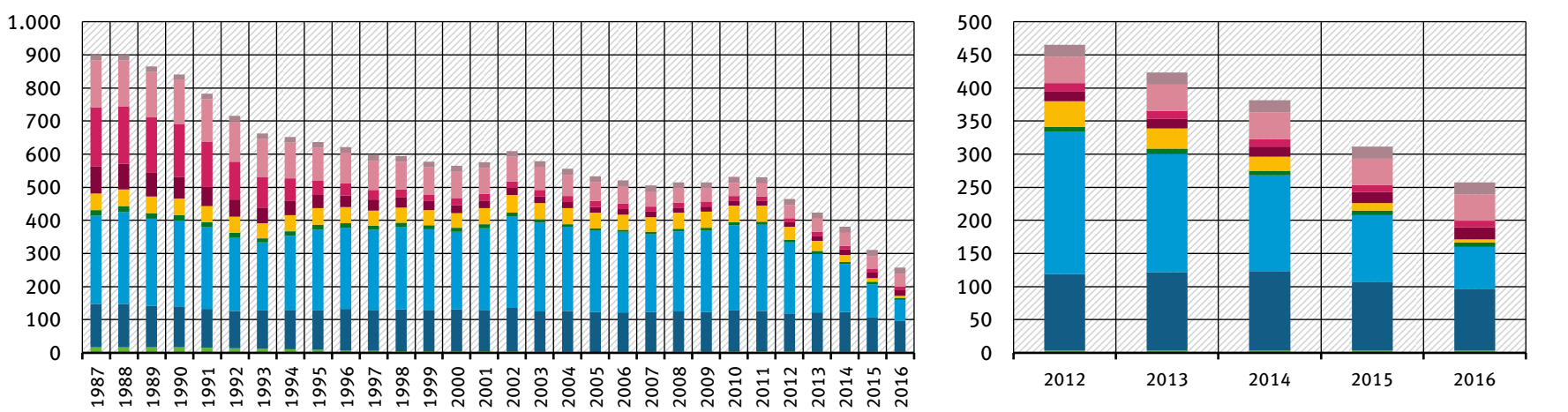
Cadmumeinträge als 5-jährige gleitende Mittel in Tonnen/Jahr
