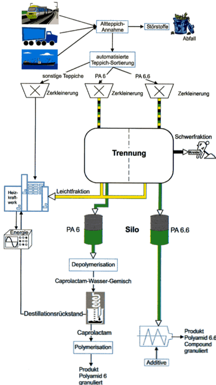
Abb.1.: In Deutschland zur Anwendung gebrachtes Verfahrensschema für das Recycling von Polyamid-Alteppichen (Quelle: Polyamid2000)
