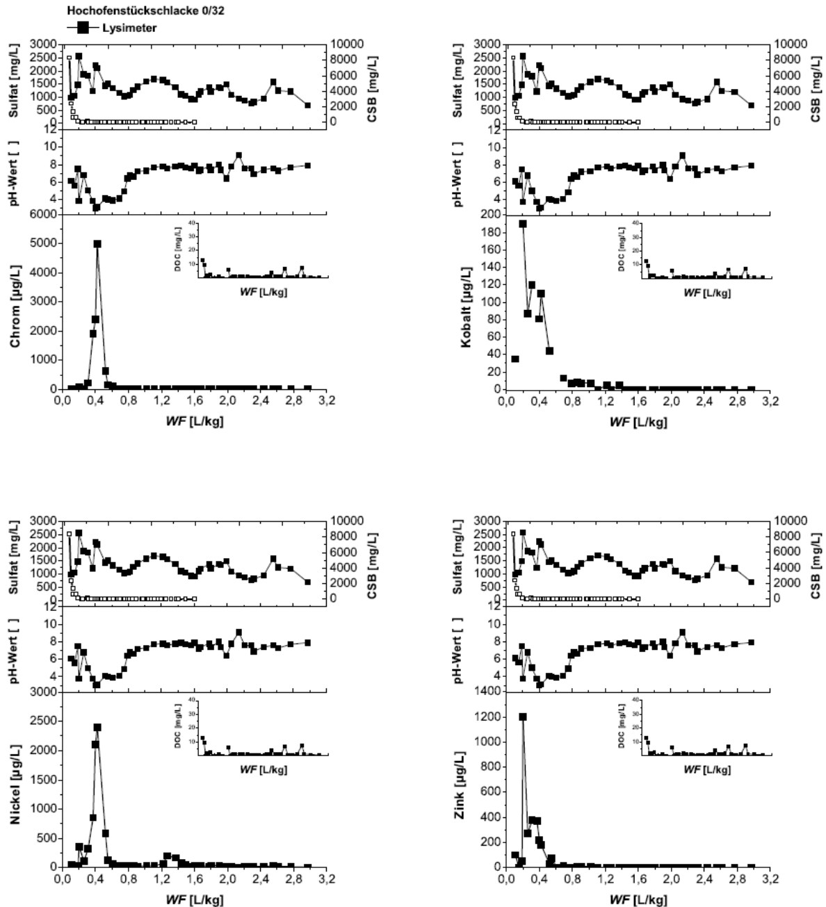
Abb. 6.3: Gegenüberstellung der zeitlichen Verläufe von Schadstoffkonzentrationen und verschiedenen physikochemischen Parametern im Sickerwasser an der Unterseite der Hochofenschlacke versus WF. Im Lysimeterablauf der Hochofenschlacke sinken die pH-Werte mit abnehmendem CSB (Umwandlung von Thiosulfat zu Sulfat und damit einhergehende Freisetzung von Protonen) vorübergehend bis auf pH = 3,0 ab. Während der „sauren Elutionsphase“ steigen die Konzentrationen einiger Schwermetalle im Lysimeterablauf auf ein Vielfaches der GFS an (aus Susset & Leuchs, 2008b).
