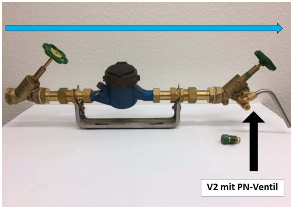
Wasserzähleranlage mit Entnahmeverrichtung für mikrobiologische und chemische Wasserproben am Ventil V2 (Entleerung/Kundenseite)
