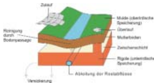
Funktionsweise des Mulden-Rigolen-Systems (schematisch)
