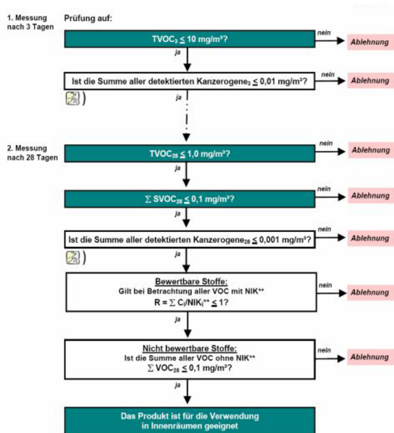
Abbildung 1: Die Stufe 2 der Zulassungsgrundsätze: das Schema zur gesundheitlichen Bewertung von VOC und SVOC-Emissionen aus Bauprodukten [AgBB 2005]
