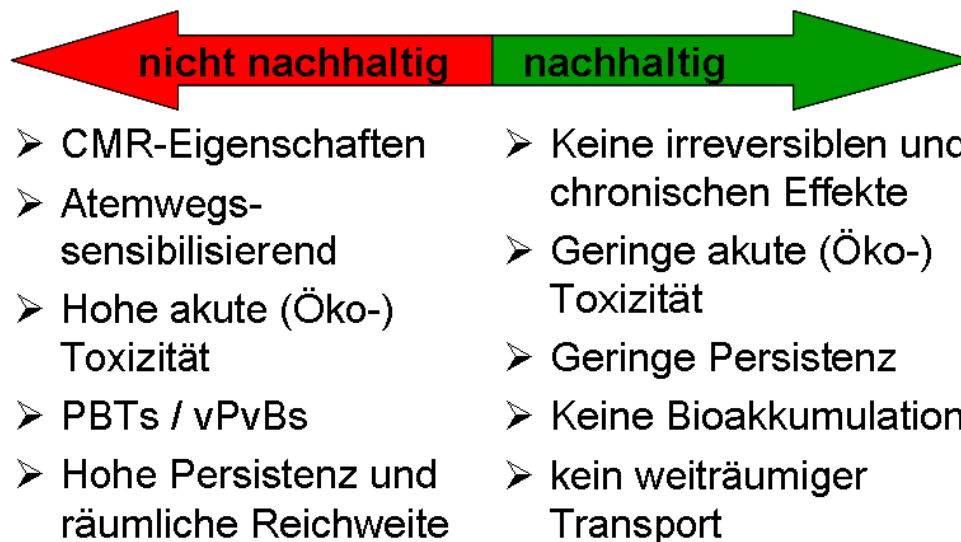
Abbildung 3: Charakteristika für nachhaltige und inhärent sichere Chemikalien
