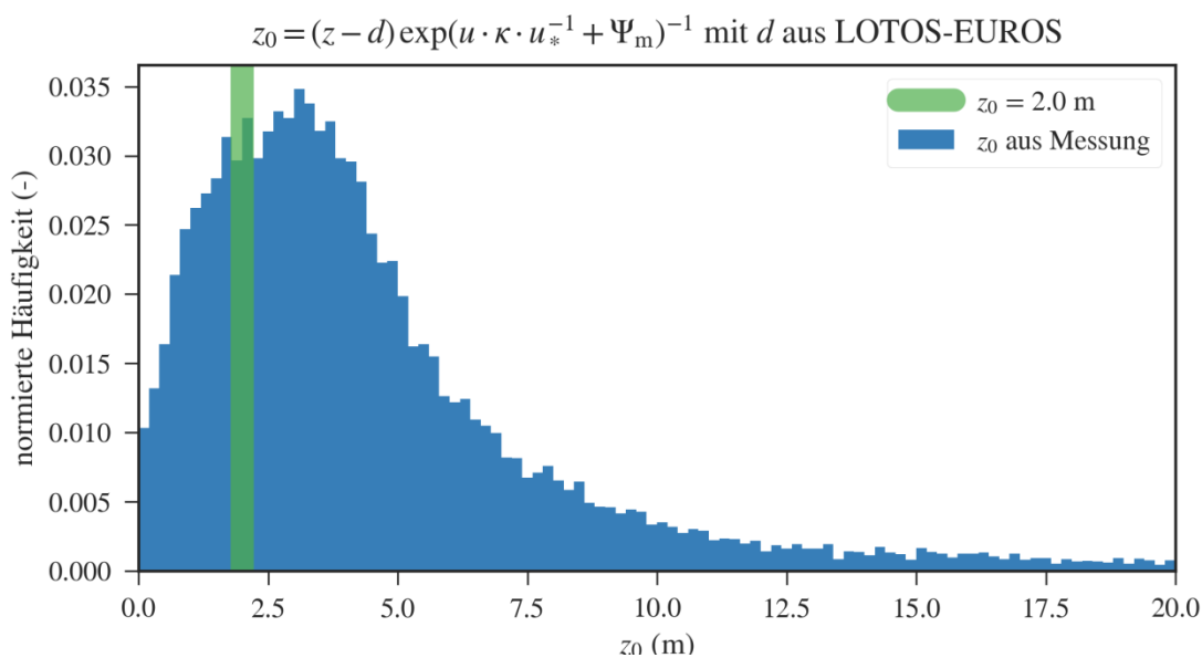
Abbildung 14: Bestimmung der Rauigkeitslänge aus Ultraschallanemometer-Messungen.
