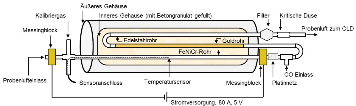
Abbildung 3: Aufbauskinne des TRANC.
