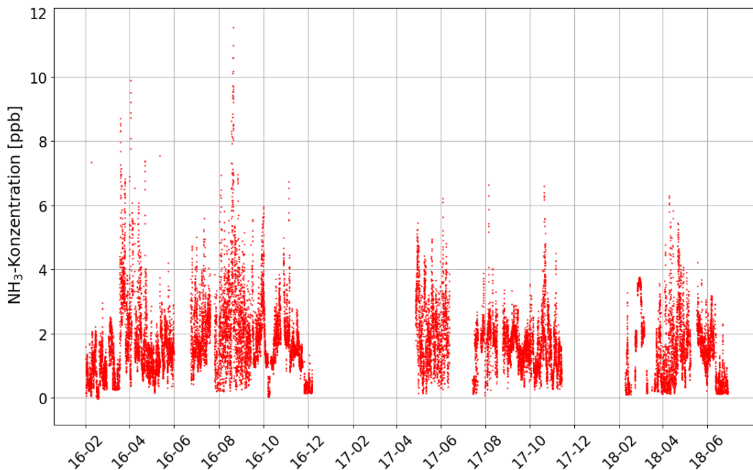
Abbildung 18: Mittlere \text{NH}_3 -Konzentrationen (30 min) vom Februar 2016 bis Ende Juni 2018.
