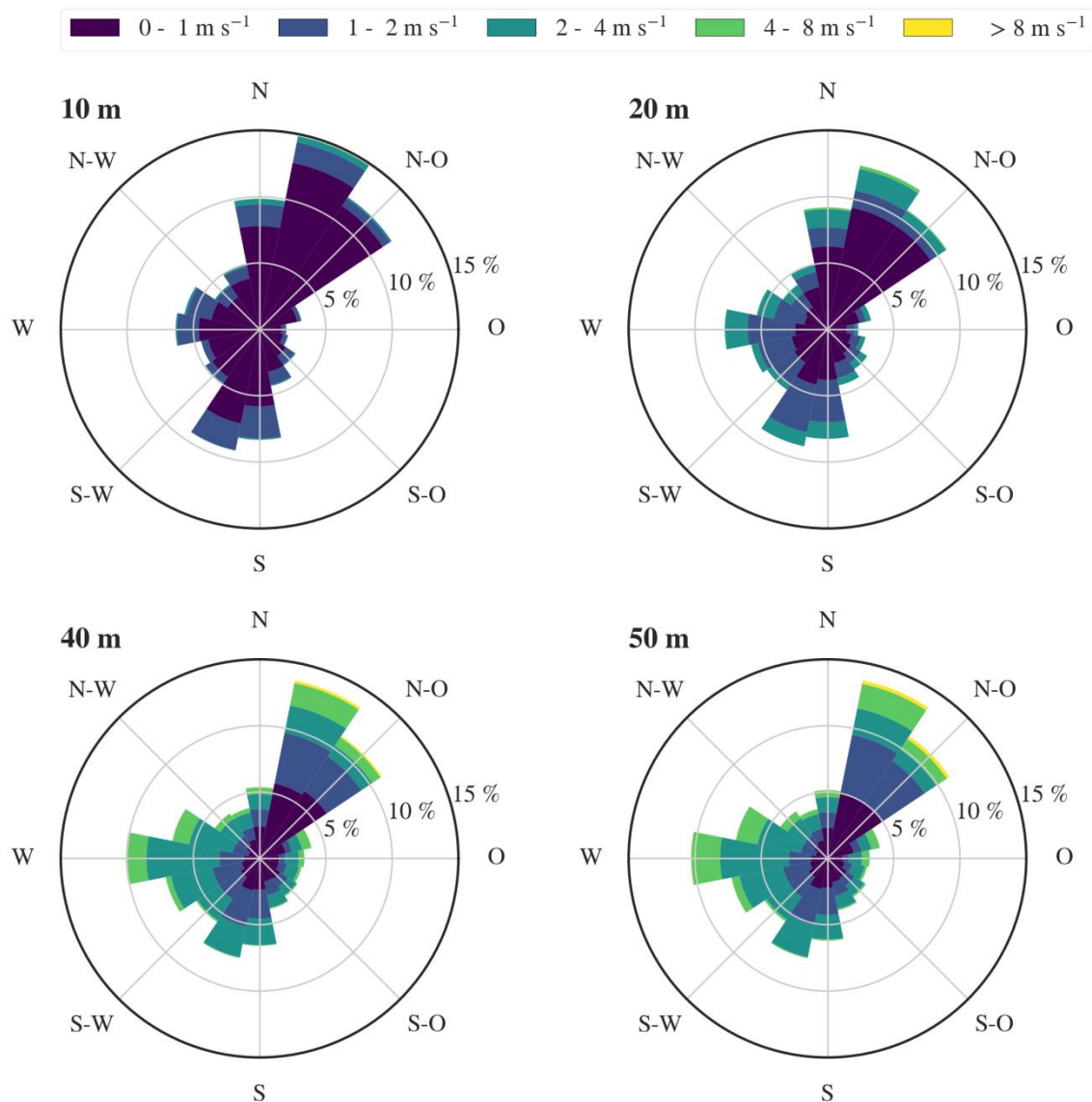
Abbildung 17: Windrosen aller vier Höhen für den Zeitraum April 2016 bis einschließlich Juni 2018 auf Halbstundenbasis.
