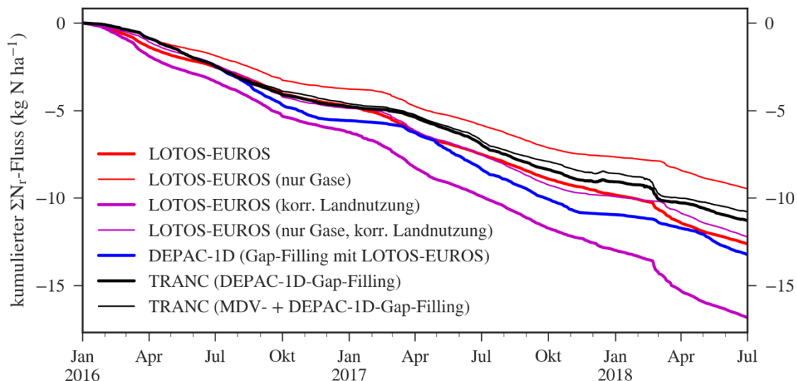
Abbildung 36: Abschätzung der trockenen Deposition am Standort Forellenbach in den Jahren 2016, 2017 und 2018 (Hochrechnung) mit verschiedenen Methoden.
