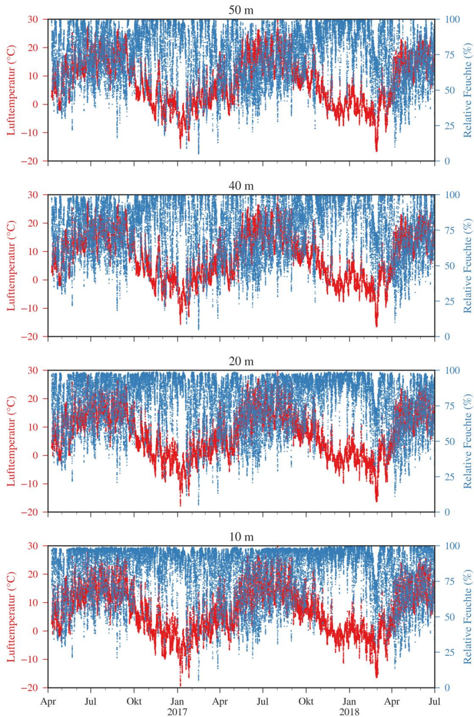
Abbildung 16: Halbstündliche Mittelwerte der Lufttemperatur (rot) und relativen Luftfeuchtigkeit (blau) auf allen vier Höhen.
