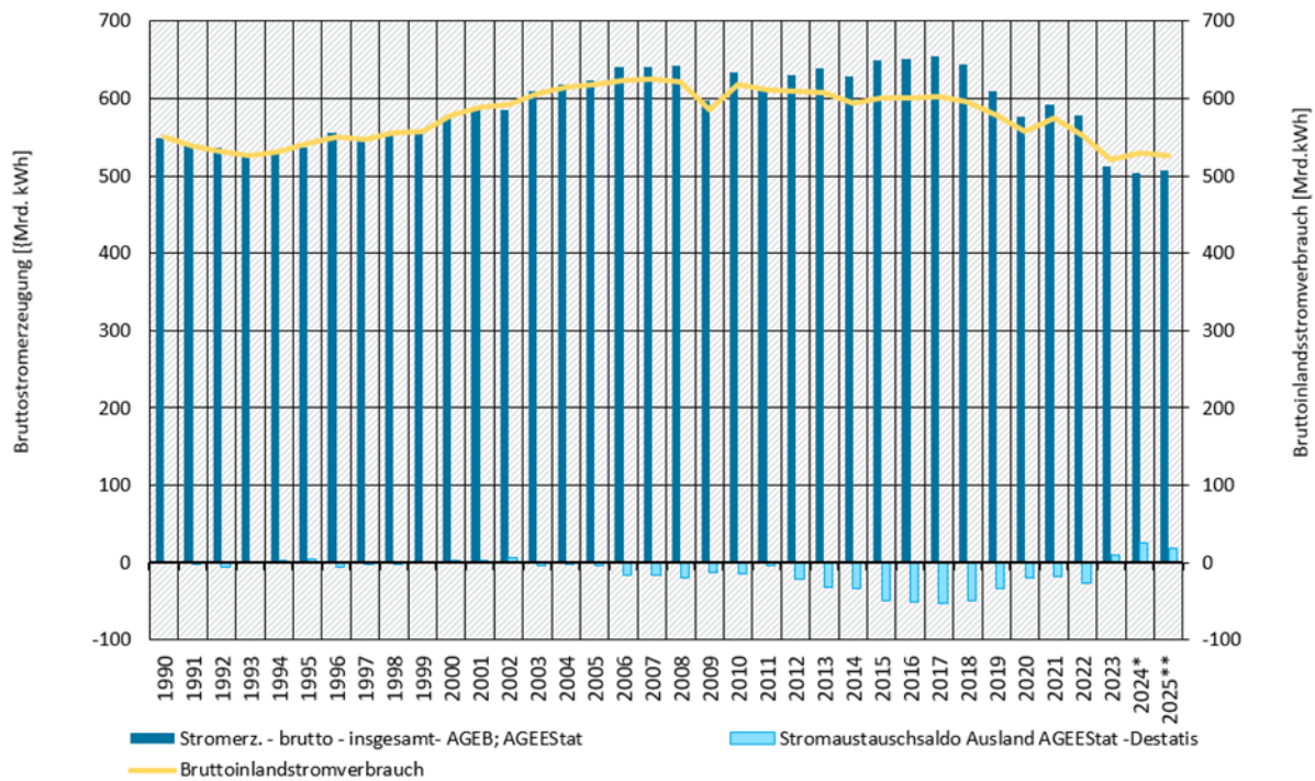
Abbildung 3: Brutto-Inlandsstromverbrauch und Stromaustauschsaldo Ausland prägen den aktuellen Trend der Bruttostromerzeugung in Deutschland
